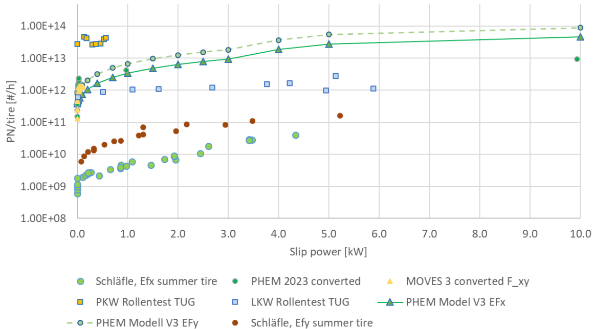
Abbildung 5-11: Charakteristische Reifenabrieb-Polygone für die PN23 Emissionen bei Längs- und Querschlupf für die Simulation in PHEM sowie verfügbare Mess- und Literaturdaten
