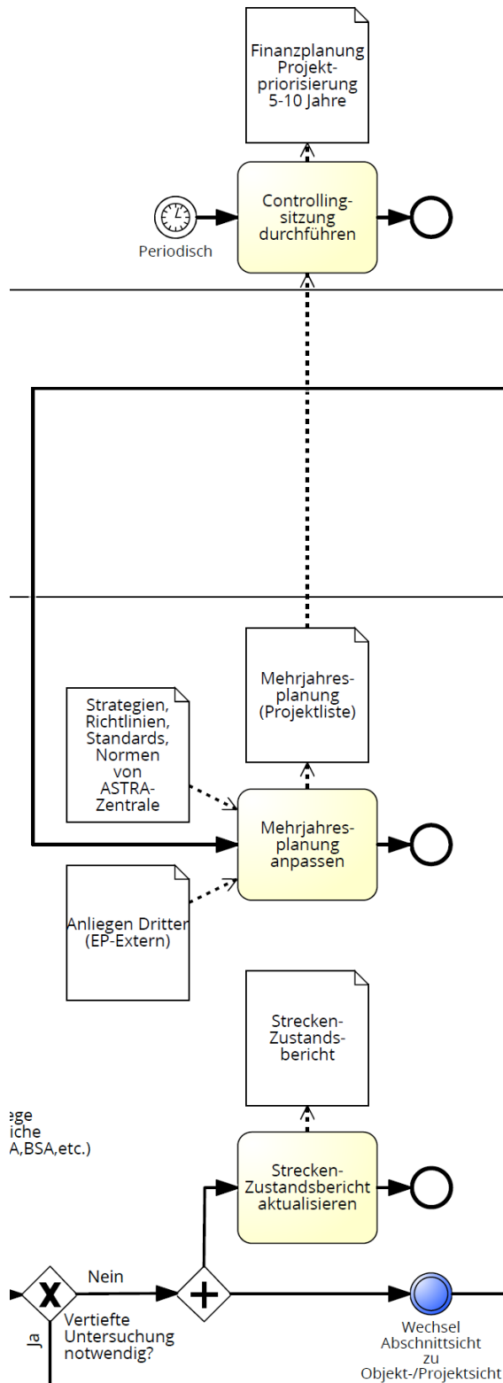
Abbildung 20: Prozessausschnitt der Erhaltungsplanung mit den Prozessschritten betreffend den Netz-, respektive Abschnitts-überblick bezüglich des Zustands und den Projekten.
