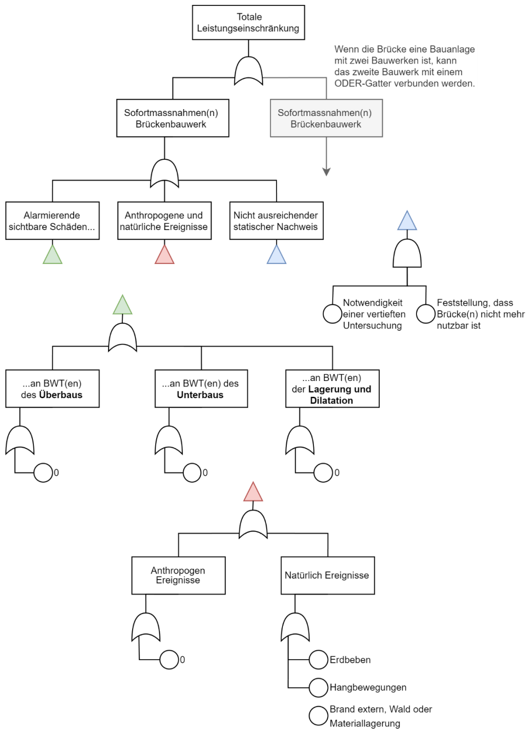
Abbildung 74: Fehlerbaum für die totale Leistungseinschränkung.
