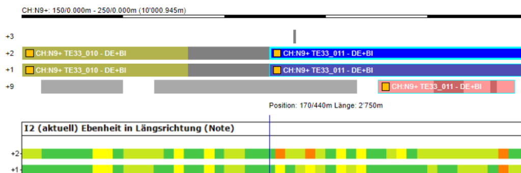
Abbildung 31: Achsbanddarstellung der potenziellen Erhaltungsobjekte und des Zustandsindex I2 (ASTRA, 2024c, S. 14).
