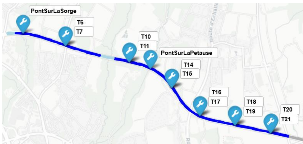
Abbildung 101: Gebündelte Massnahmen im Jahr 6 (erstes Bündel, Anlagen in dunkler Farbe, Erhaltungsabschnitt in heller Farbe).
