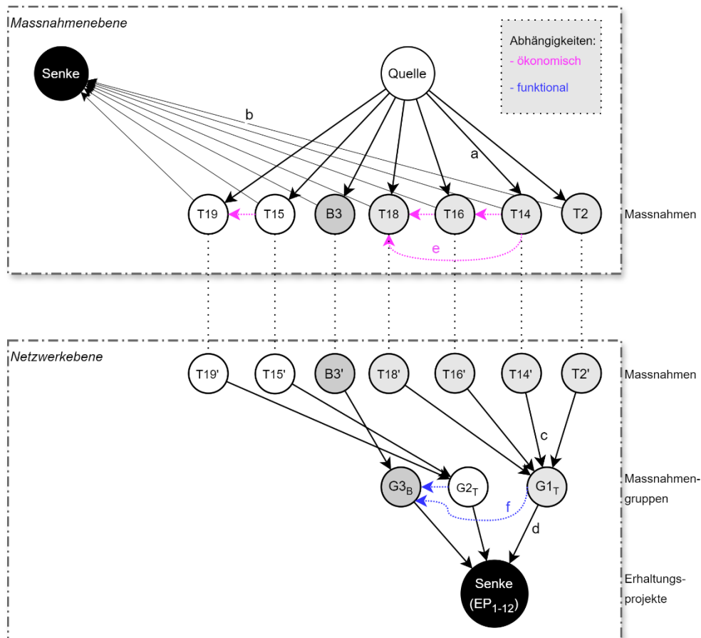
Abbildung 98: Beispielgraph G für Massnahmen an mehreren Trasse-Teilstücken und der Brücke B3.
