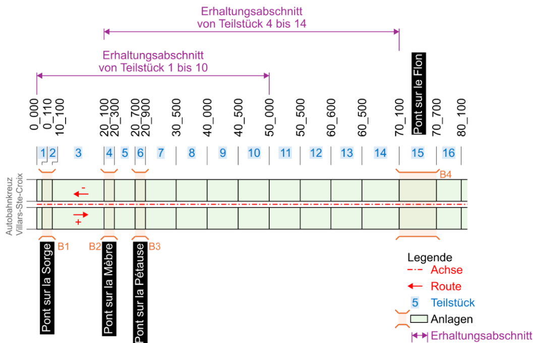
Abbildung 95: Schematische Darstellung der Erhaltungsabschnittsoptionen der ersten Kilometer der Teststrecke.
