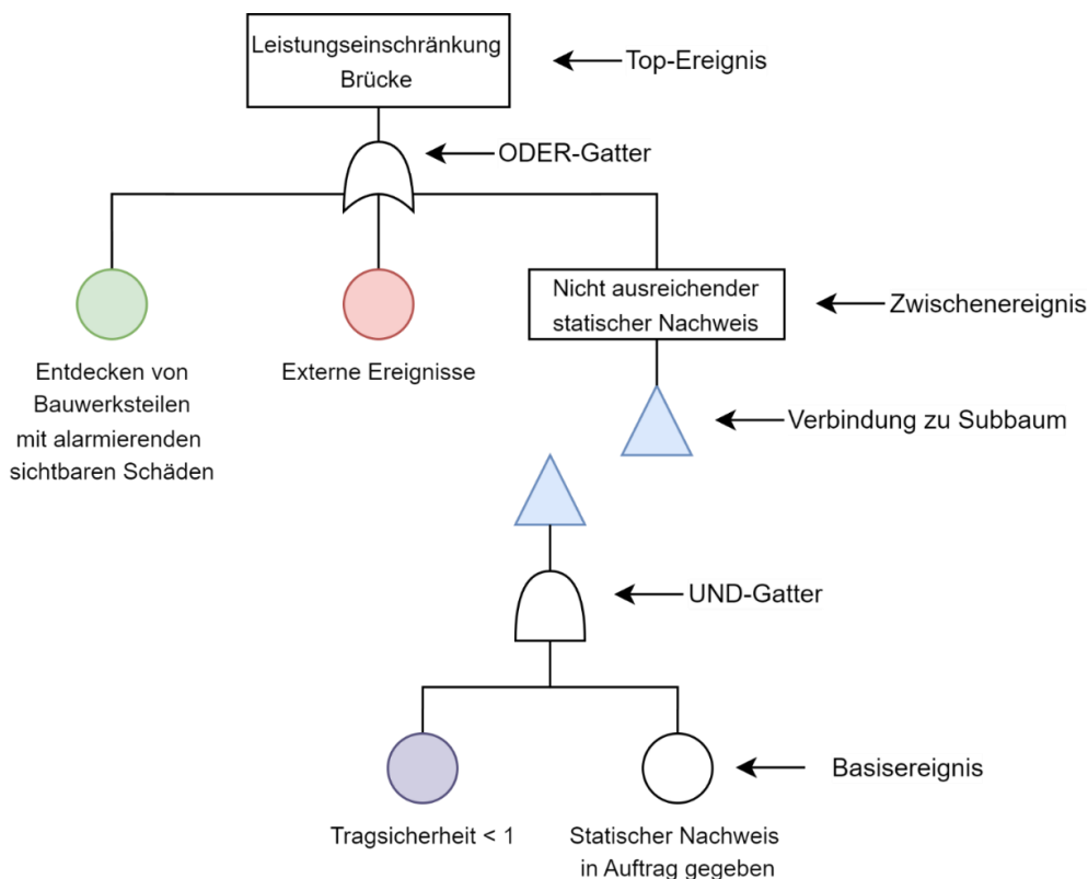
Abbildung 71: Beispiel eines Fehlerbaums.
