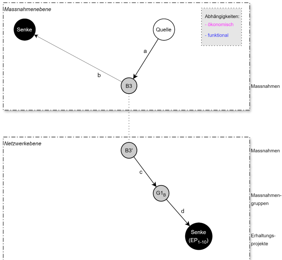
Abbildung 97: Beispielgraph G mit Unterhaltsmassnahme an Brücke B3.
