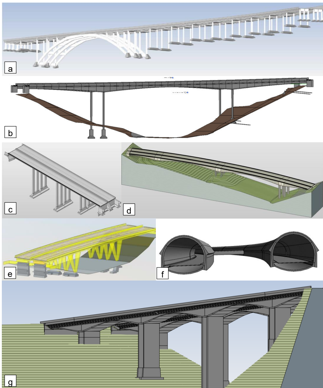
Abbildung 108: BIM-Modelle aus dem Projekt MINERVA. a) Pont sur le Flon, b) Pont sur la Sorge, c) Pont sur la Mèbre, d) Pont sur la Lutrive, e) Pont sur la Pétause, f) Tunnel du Flonzaley, g) Pont sur la Paudèze
