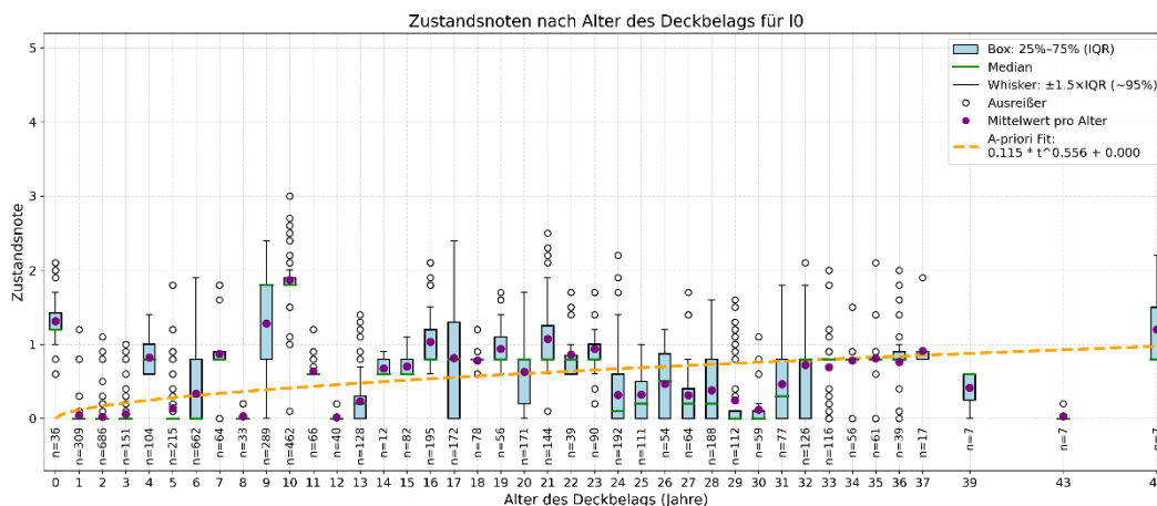
Abbildung 56: Übersicht der Zustandsnoten in Abhängigkeit des Alters des Deckbelags mit der angeglichenen a priori Prozessfunktion für den Indikator I0.
