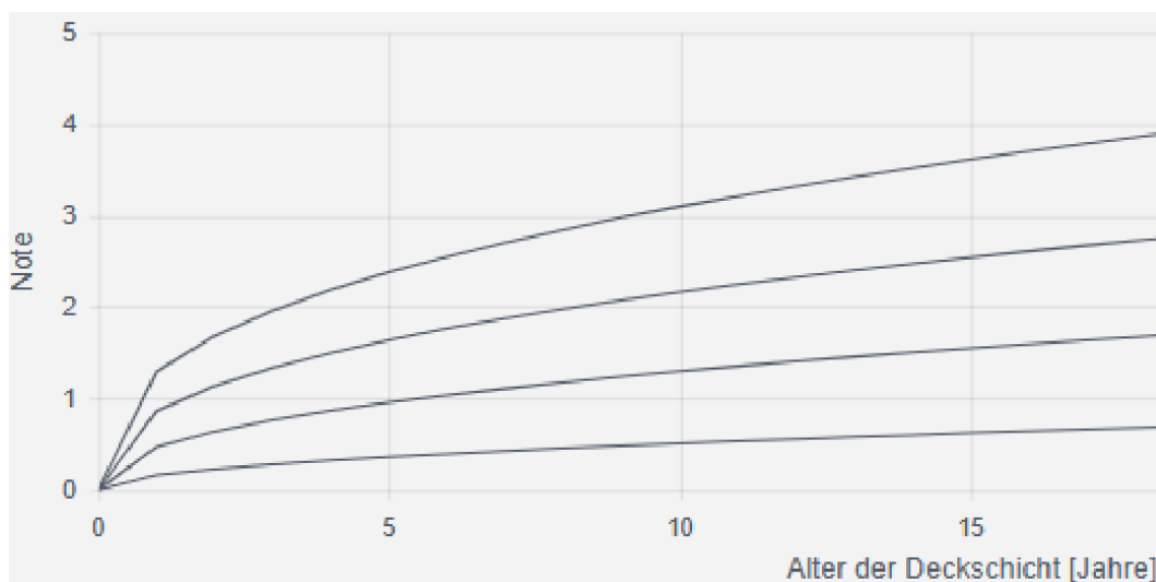
Abbildung 32: Verlaufskurve für die Zustandsprognose im ASTRA für Index I3 (ASTRA, 2024b, S. 91). Die Linien sind von unten nach oben VK1 bis VK4.
