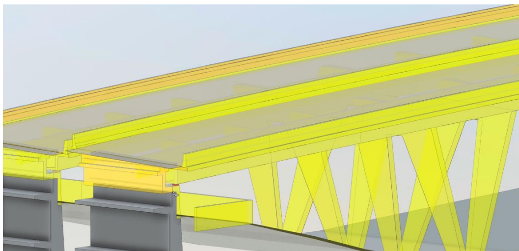
Abbildung 113: BIM-Modell mit den Bauwerksteilen gemäss dem Zustand eingefärbt.
