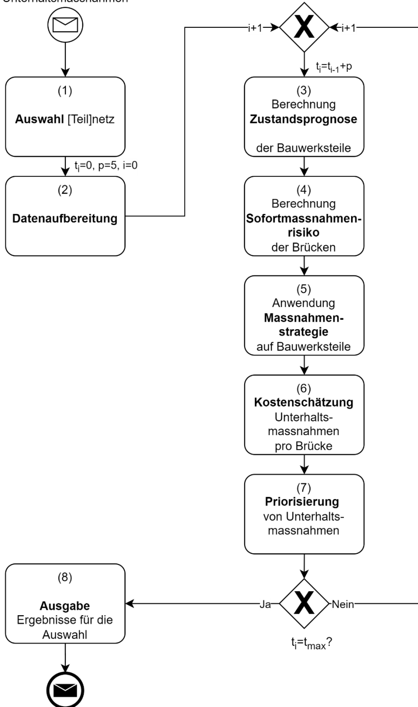
Abbildung 70: Algorithmus zur Prognose von Unterhaltsmassnahmen im ASTRA für Brücken.
