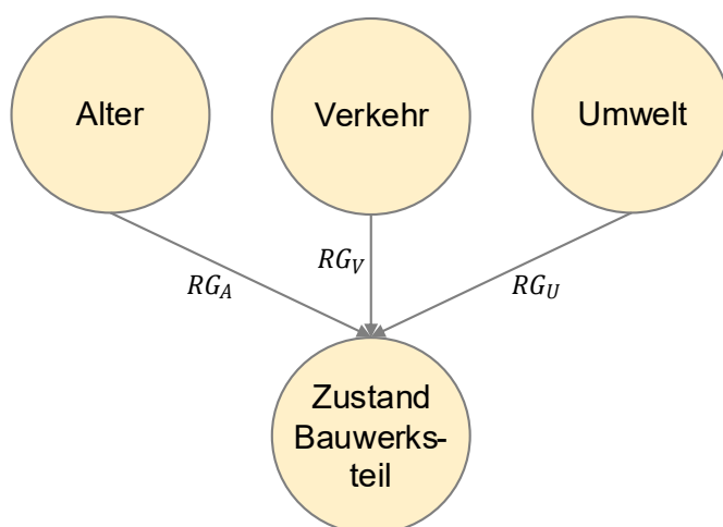
Abbildung 35: Bayes'sches Netz mit den Einflussgrössen für die Abschätzung des Zustands eines Bauwerksteils und den relativen Gewichten (RG) der einzelnen Einflussgrössen.
