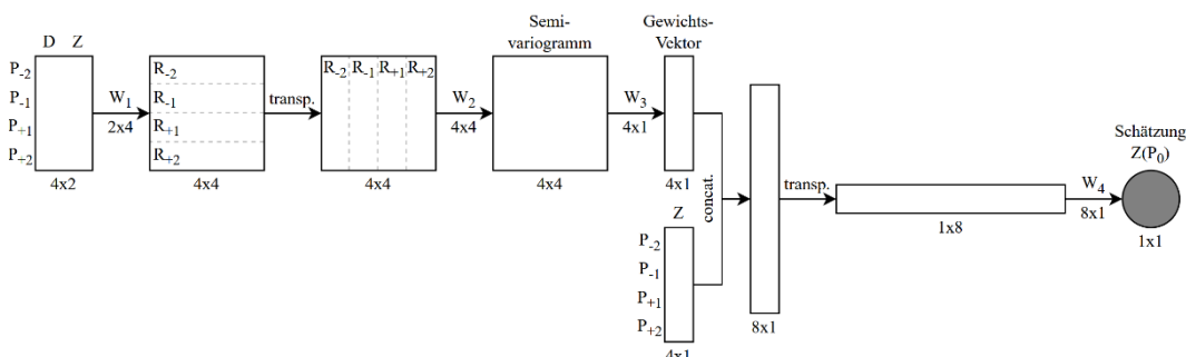
Abbildung 48: Struktur des verwendeten ANN-Kriging-Modells am Beispiel von 4 Nachbarn ( D =Distanz, Z =Zustandsnote, W =trainierte Gewichte).
