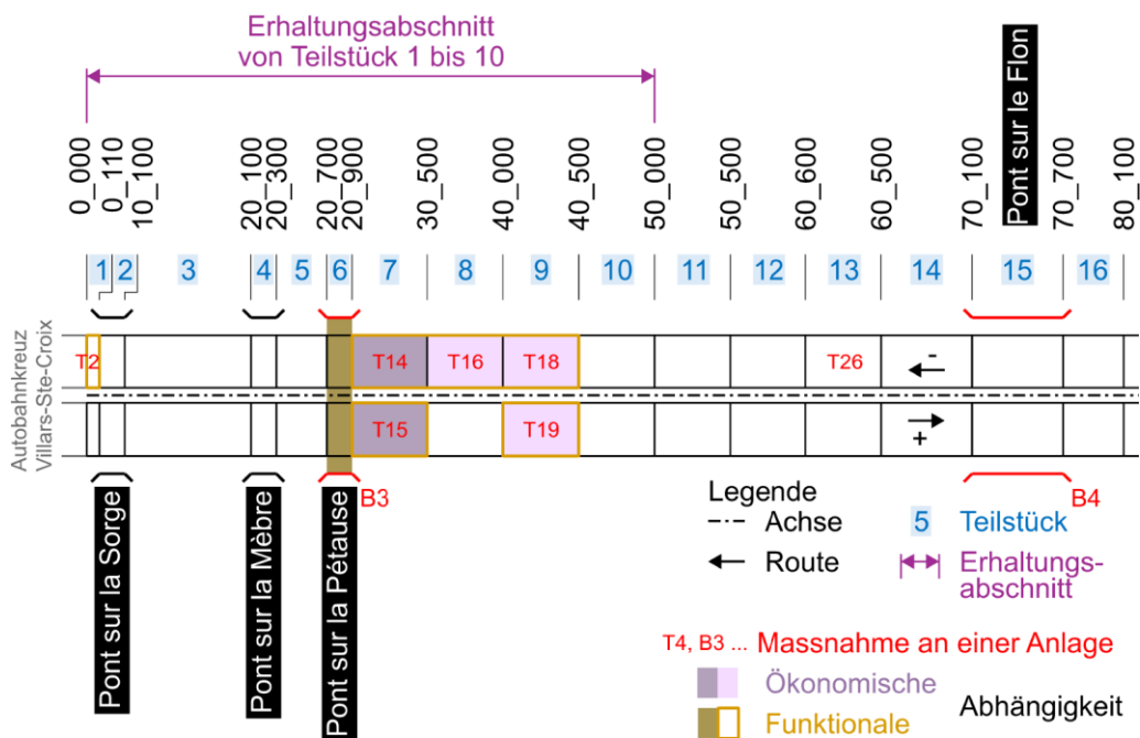
Abbildung 99: Netzwerkillustration zum Beispielgraph G für Massnahmen an mehreren Trasse-Teilstücken und der Brücke B3.
