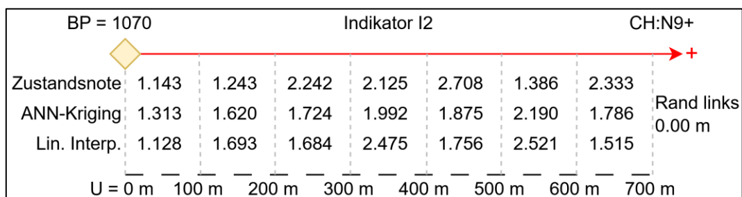
Abbildung 55: Beispiel der Abschätzung der Zustandsnote für den Indikator I2 am Datensatz des Jahres 2024 an einer Strassenbewertungsfläche.
