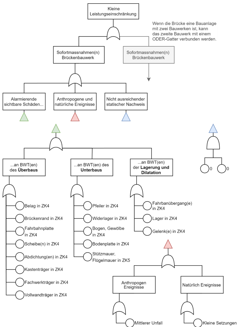
Abbildung 72: Fehlerbaum für die kleine Leistungseinschränkung.
