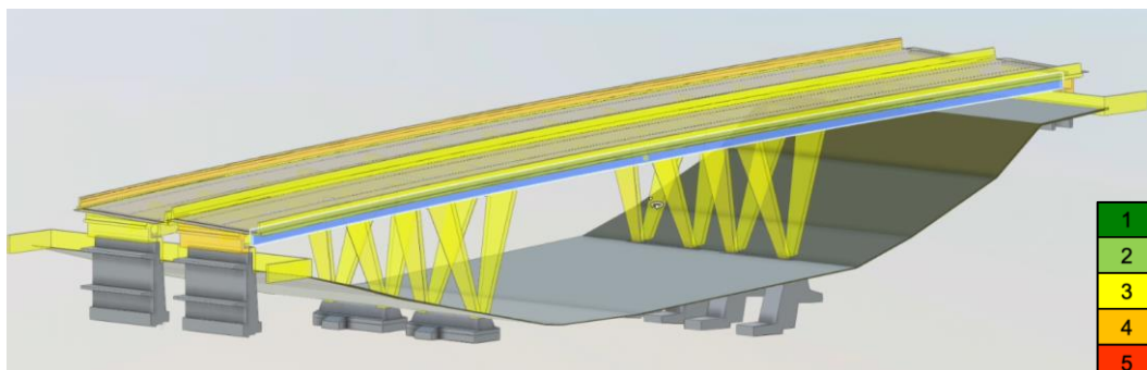
Figure 8: Modèle BIM permettant d'afficher des prévisions de l'état de différentes parties de l'ouvrage (bleu = partie de l'ouvrage sélectionnée ; vert à rouge : couleurs correspondant à la classification de l'état des ouvrages d'art définie par l'OFROU).
