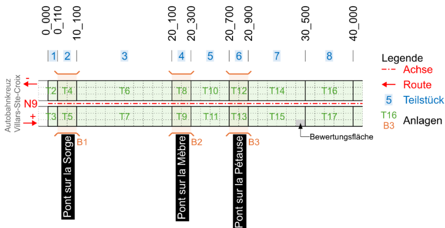
Abbildung 94: Schematische Darstellung der topologischen Modellierung der ersten Kilometer der Teststrecke.
