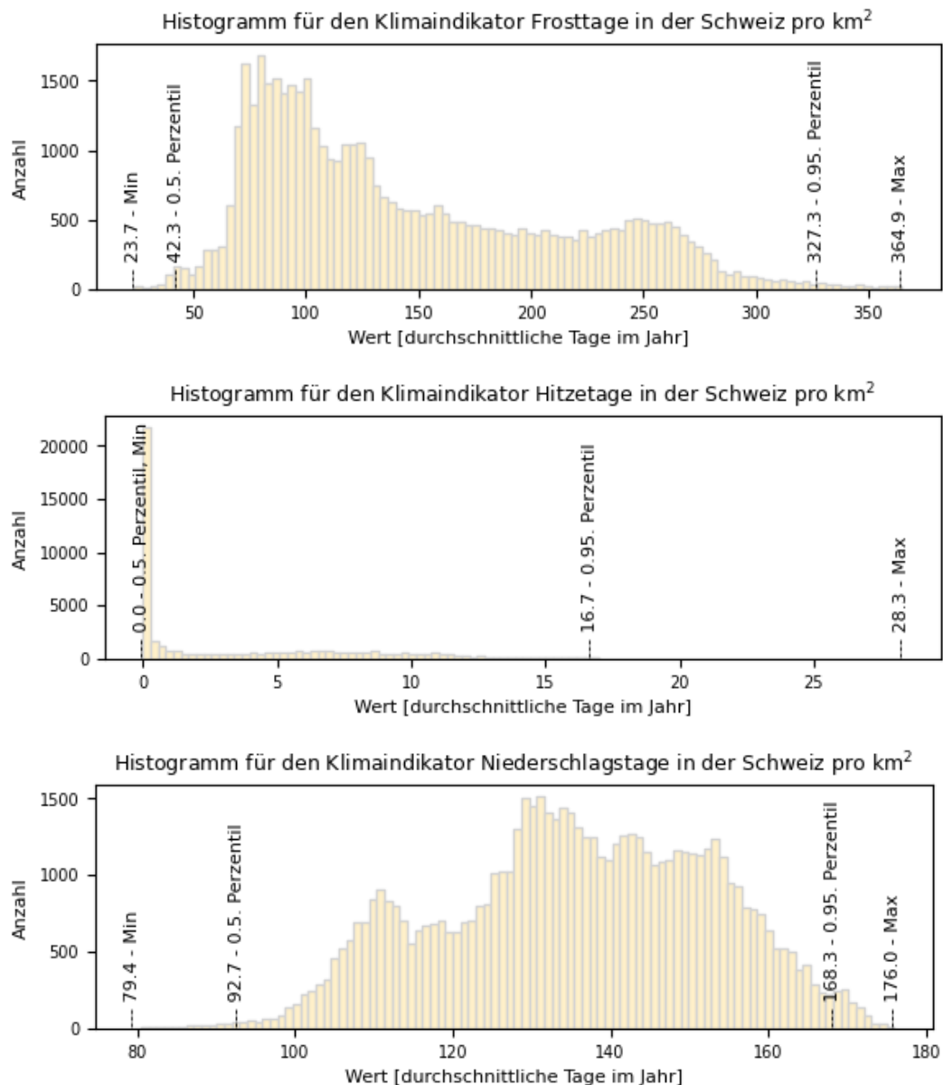
Abbildung 39: Histogramme der durchschnittlichen Anzahl Tage im Jahr für die drei Klimaindikatoren (Frost, Hitze, Niederschlag) für jeden Quadratkilometer in der Schweiz über die Jahre 1991 bis 2020 (Hervorhebung der Werte Min und Max sowie der Perzentile für die Normalisierung).
