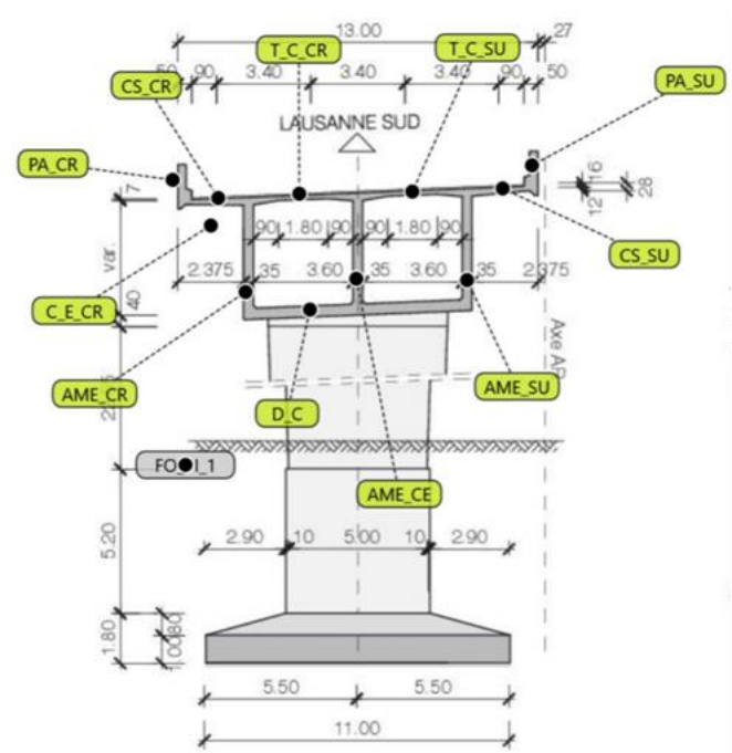
Abbildung 30: Querschnitt Pont sur La Sorge - droit mit Bauwerksteilbezeichnung (ASTRA, 2024a).
