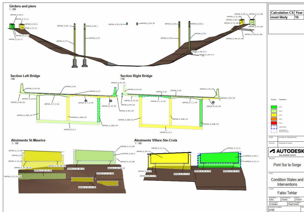
Abbildung 112: Mögliche Darstellung der Bauwerksteile eines Modells in einem Übersichtsblatt.
