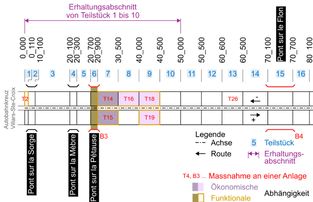
Abbildung 96: Darstellung der berücksichtigten Abhängigkeiten zwischen Bauanlagen und Trasse-Teilstücken.
