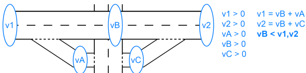
Abbildung 46: Illustration der Herleitung des maximalen Verkehrsflusses über eine Brücke zwischen Ein- und Ausfahrten.
