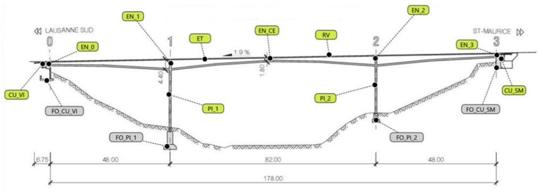
Abbildung 29: Längsschnitt Pont sur La Sorge - droit mit Bauwerksteilbezeichnung (ASTRA, 2024a).
