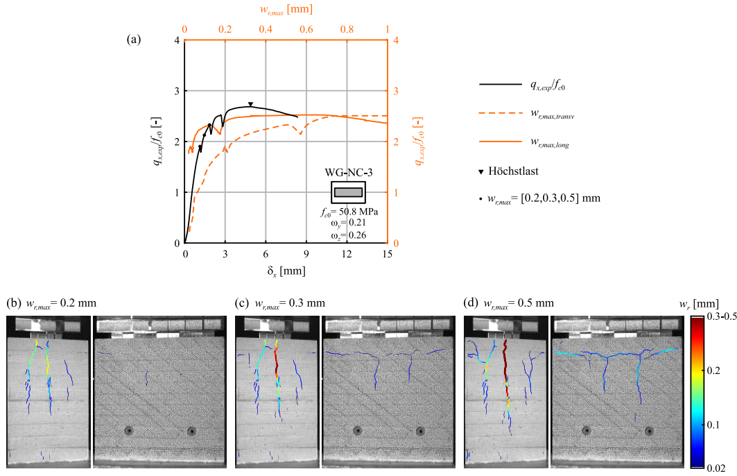
Abbildung 10: Tragverhalten und Rissentwicklung eines Blockversuchs.
