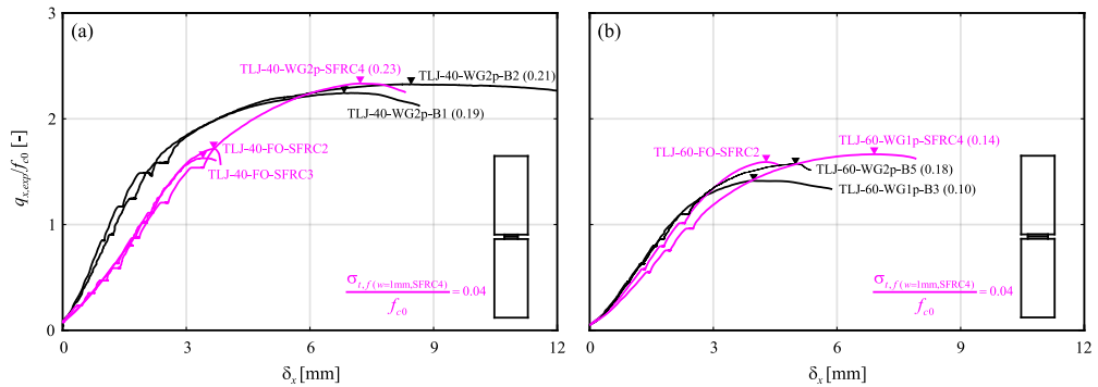
Abbildung 20: Vergleich der Fugenversuche mit stahlfaserbewehrtem Beton (lila) und konventionellem Beton (schwarz). (a) Belastungsbreite 140 mm; (b) Belastungsbreite 210 mm. Mechanischer Bewehrungsgehalt in Klammern (für hybrid bewehrte Versuchskörper Summe aus konventioneller Bewehrung und residualer Zugfestigkeit). Abkürzungen: FO = fibres only (keine konventionelle Bewehrung) und WG = Welded grids (geschweisste Leiterbewehrung). Im Vergleich zu [1] wurde Versuchskörper TLJ-60-WG2p-B5 zusätzlich in der Grafik integriert.
