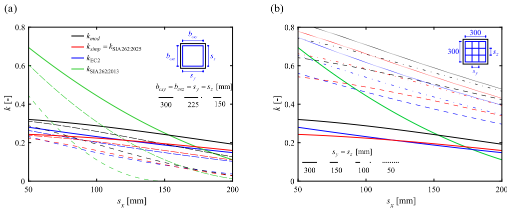
Abbildung 6: Vergleich des Effektivitätsfaktors ( A_{conf}/A_{cs} ) der verschiedenen Modelle in Funktion des vertikalen Bewehrungsabstandes s_x – (a) variable Querschnittsgrösse mit einem Bügel und (b) konstanter Querschnitt mit unterschiedlicher Bewehrungsanzahl.
