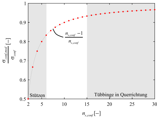
Abbildung 5: Vergleich der Umschnürungsspannung nach dem neuem Modell ( \sigma_{conf,mod} ) mit dem Ansatz bestehender Normen ( \sigma_{conf} ).
