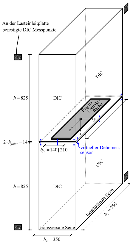
Abbildung 13: Geometrie der Fugenversuche [mm].
