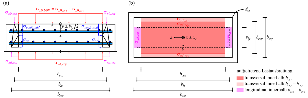
Abbildung 16: (a) Longitudinale Lastausbreitung und (b) horizontaler Schnitt mit belasteten Flächen durch Lastausbreitung.
