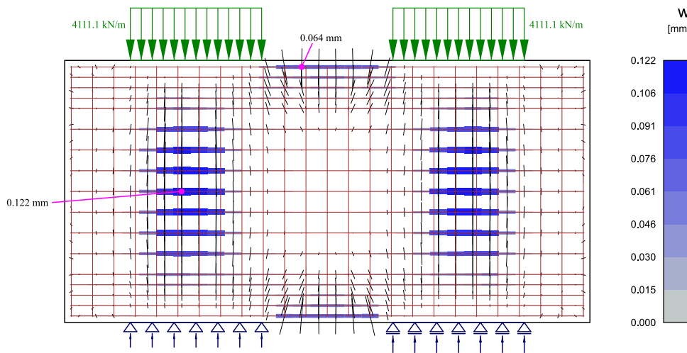
Abbildung 22: Rissbreiten ermittelt mit Idea StatiCa Detail im Grenzzustand der Gebrauchstauglichkeit (GZG).
