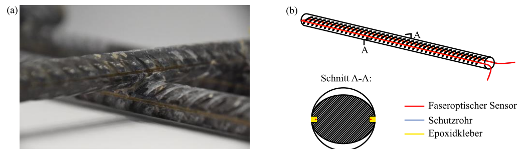
Abbildung 7: Instrumentierung der Leiterbewehrung – (a) geschweißter Kreuzungsstoss mit faseroptischem Sensor in Nut und geschützt mit einem Epoxidharz und (b) schematische Zeichnung der Sensoranordnung.
