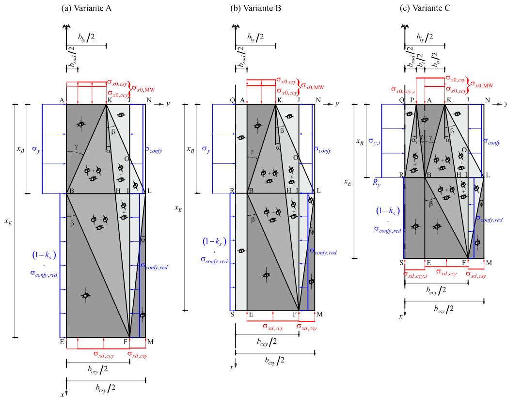
Abbildung 17: Verschiedene Varianten zur Berücksichtigung einer Fugenaussparung aufgrund eines Führungsstabes basierend auf dem Multi-Wedge Spannungsfeld.
