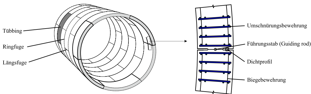
Abbildung 2: Definition der Parameter der Tübbinge und der Längsfuge.
