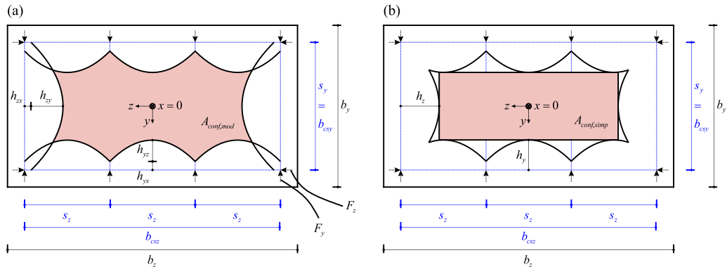
Abbildung 4: Massgebender Querschnitt – (a) umschnürte Fläche und (b) vereinfachte umschnürte Fläche.
