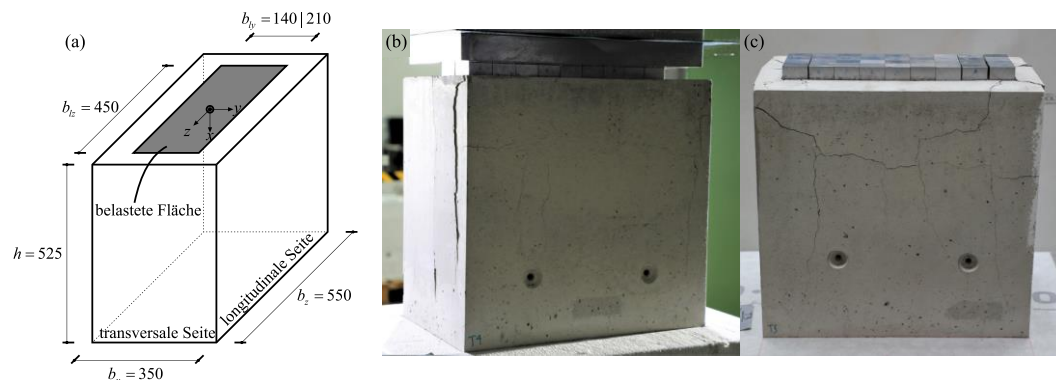
Abbildung 8: Blockversuche – (a) Geometrie Versuchskörper [mm], (b) Versuchsaufbau und (c) geprüfter Versuchskörper.
