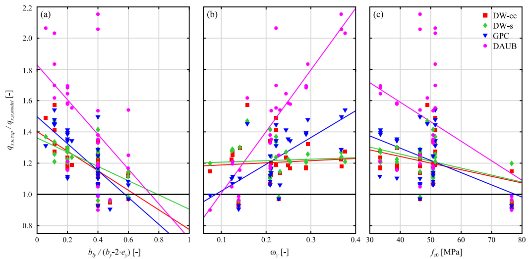
Abbildung 12: Vergleich der Modellvorhersagen mit den experimentellen Versuchsergebnissen geplotet in Funktion von (a) Last-Konzentrations-Verhältnis, (b) transversalem mechanischem Bewehrungsgehalt und (c) Betondruckfestigkeit.
