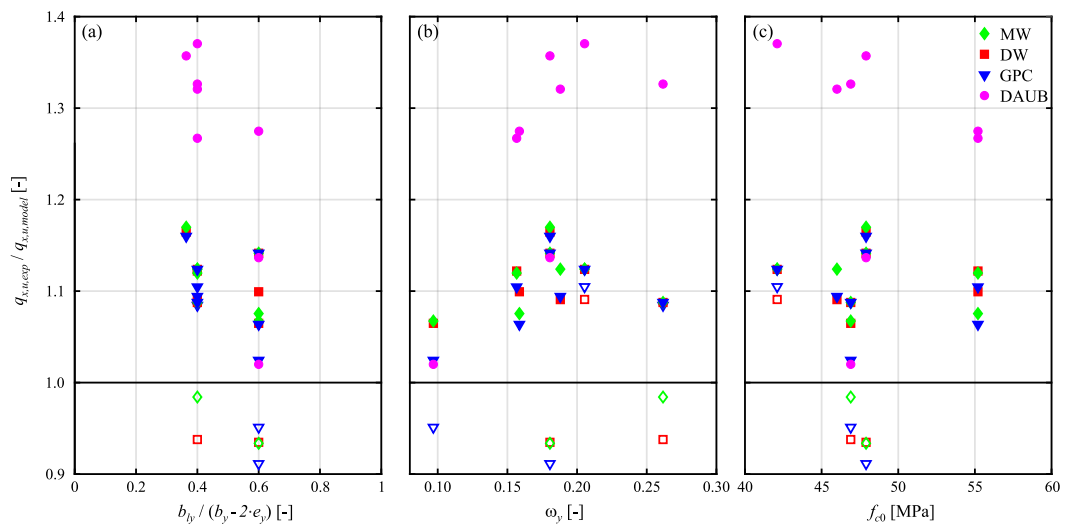
Abbildung 18: Vergleich der Modellvorhersagen mit den experimentellen Resultaten der Fugenversuche ohne Fugenaussparung geplottet in Funktion von (a) Last-Konzentrations-Verhältnis, (b) transversalem mechanischen Bewehrungsgehalt und (c) Beton-druckfestigkeit.
