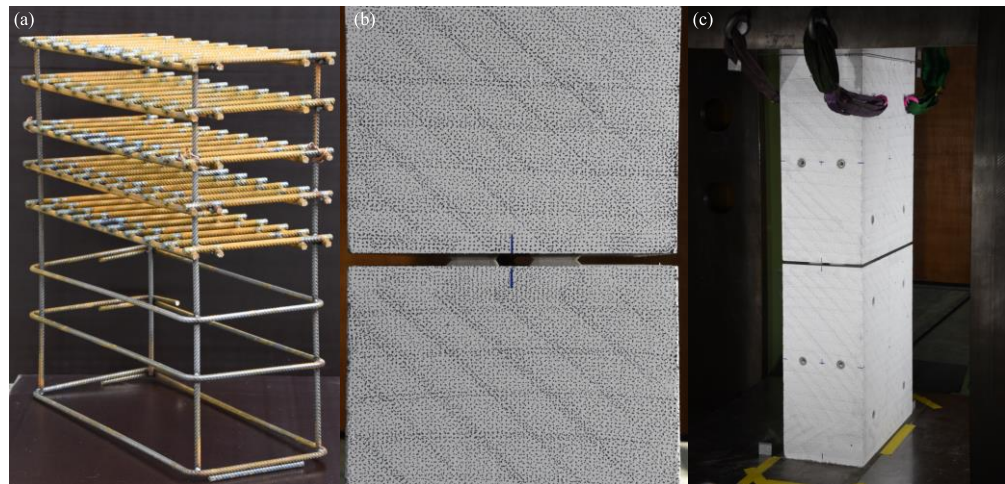
Abbildung 14: Fugenversuche – (a) Geschweisste Leiterbewehrung, (b) Fugenausbildung mit Aussparung für Führungsstab und (c) Versuchsaufbau.
