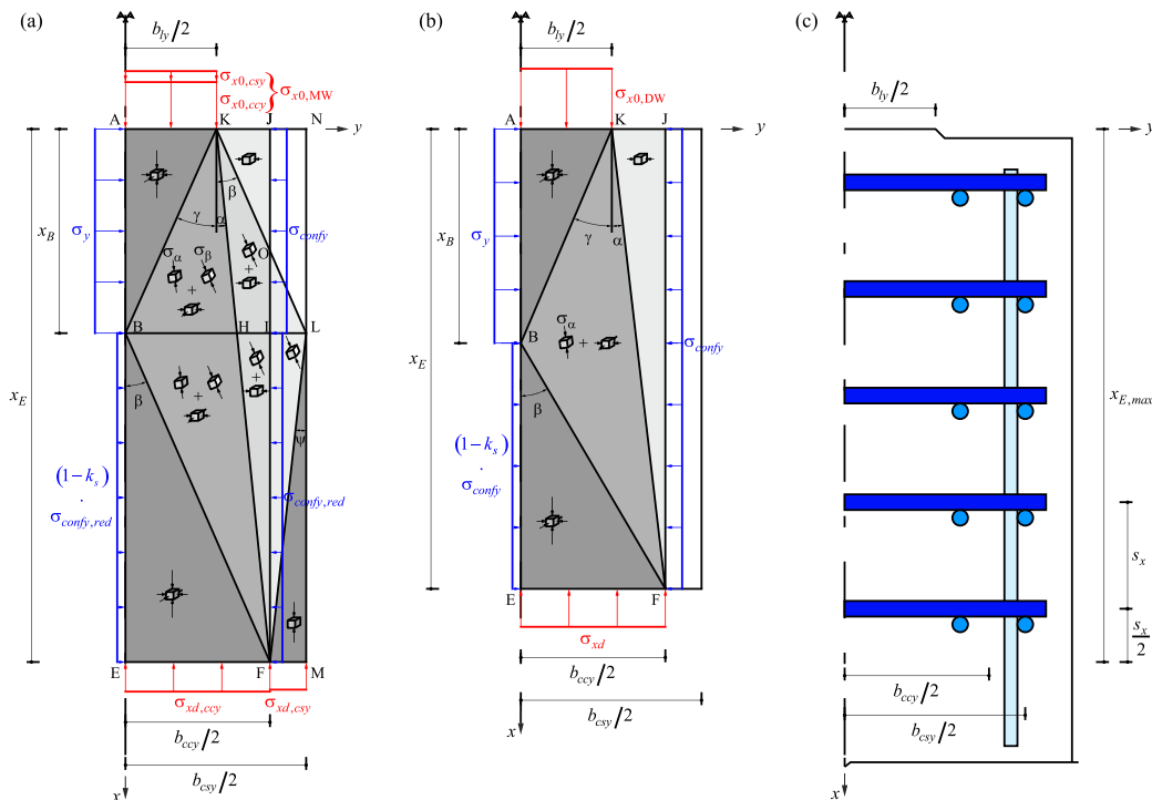
Abbildung 15: Modellierung der Längsfugen – (a) Multi-Wedge Spannungsfeld, (b) Dual-Wedge Spannungsfeld und (c) zugehöriges Bewehrungslayout. Es ist jeweils nur eine Symmetriehälfte dargestellt und die lateralen und vertikalen Spannungen sind unterschiedlich skaliert.
