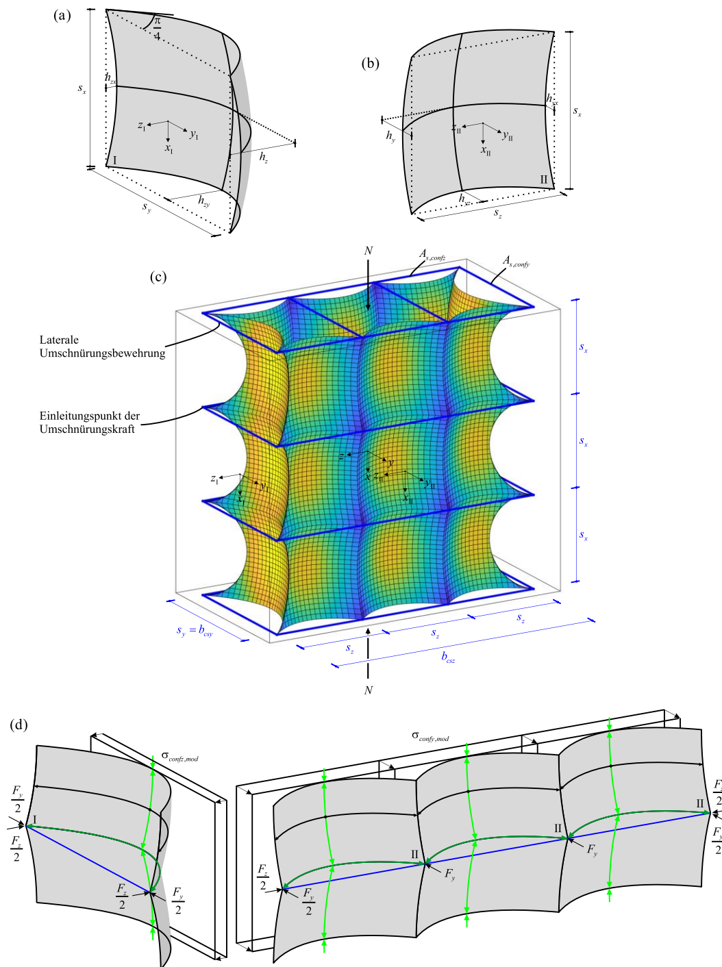
Abbildung 3: Umschnürungsmodell – (a) und (b) Definition der Paraboloiden, (c) umschnürtes Betonvolumen und (d) Kraftfluss.
