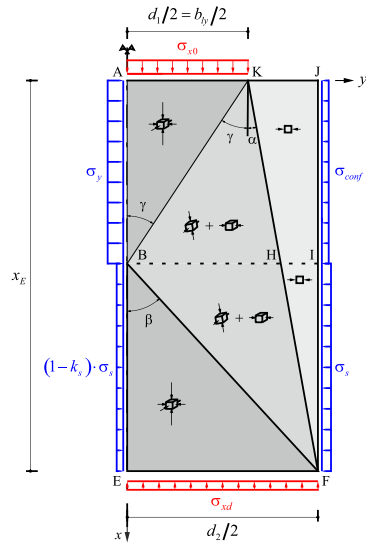
Abbildung 11: Dual-Wedge Spannungsfeld.
