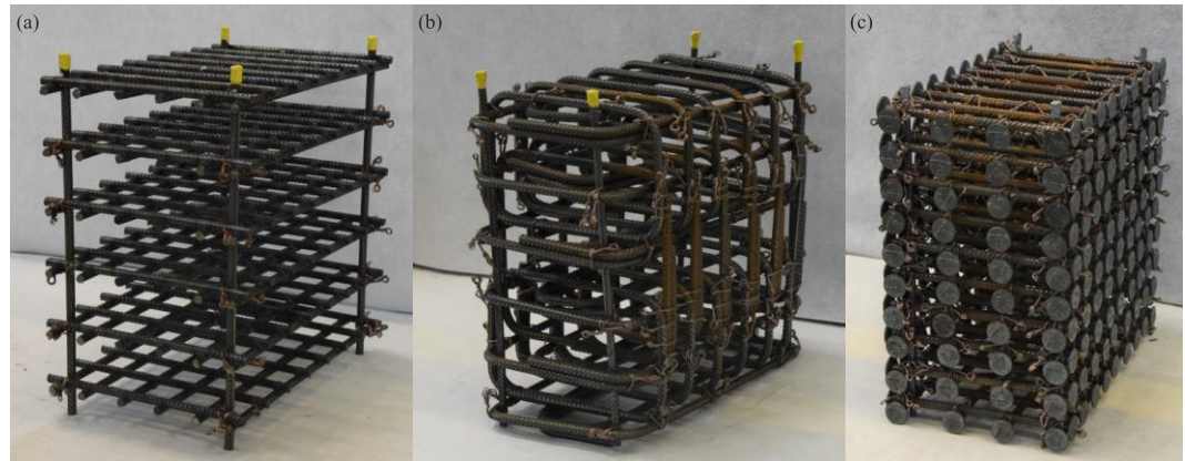
Abbildung 9: Verschiedene Bewehrungstypen. (a) geschweisste Leiterbewehrung, (b) Bügelbewehrung und (c) Dübelbewehrung.
