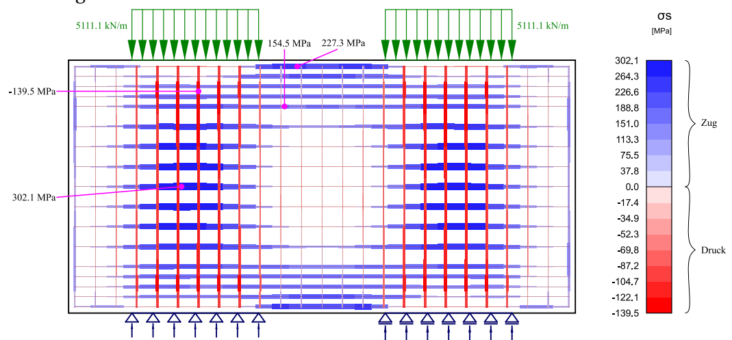
Abbildung 21: Bewehrungsspannungen ermittelt mit Idea StatiCa Detail im Grenzzustand der Tragsicherheit (GZT).
