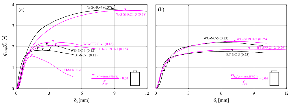
Abbildung 19: Vergleich der Blockversuche mit stahlfaserbewehrtem Beton (lila) und konventionellem Beton (schwarz). (a) Belastungsbreite 140 mm; (b) Belastungsbreite 210 mm. Mechanischer Bewehrungsgehalt in Klammern (für hybrid bewehrte Versuchskörper Summe aus konventioneller Bewehrung und residueller Zugfestigkeit). Abkürzungen: FO = fibres only (keine konventionelle Bewehrung), WG = Welded grids (geschweisste Leiterbewehrung und BT = Bent ties (Bügelbewehrung).
