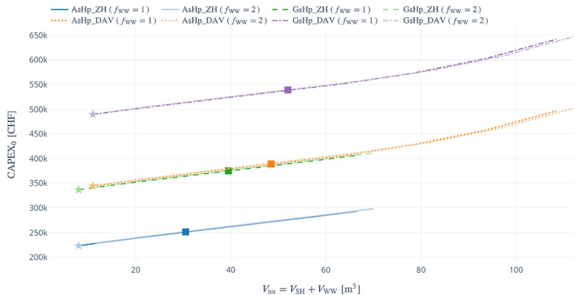
Abbildung 33: MFH145: Darstellung analog zu Abbildung 31
