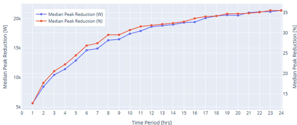
Abbildung 28: Median der Lastspitzenreduktion über alle drei Jahre der Messdaten in stündlichen Abstufungen.
