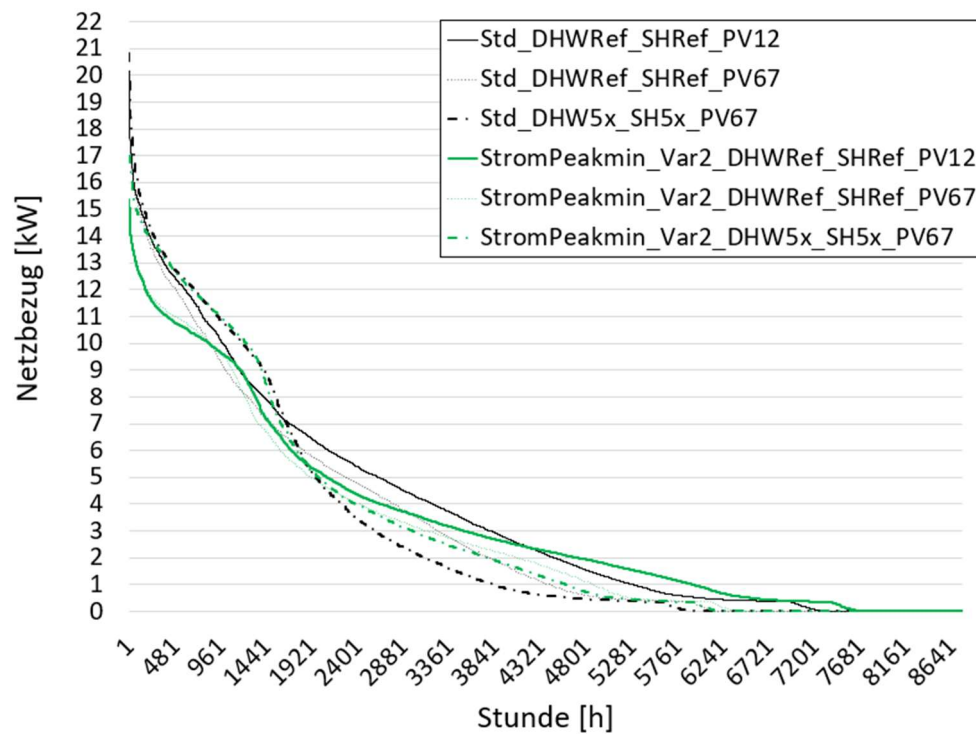
Abbildung 41: Jahresdauerlinien des elektrischen Netzbezuges für sechs Fälle der Simulationsstudie I.
