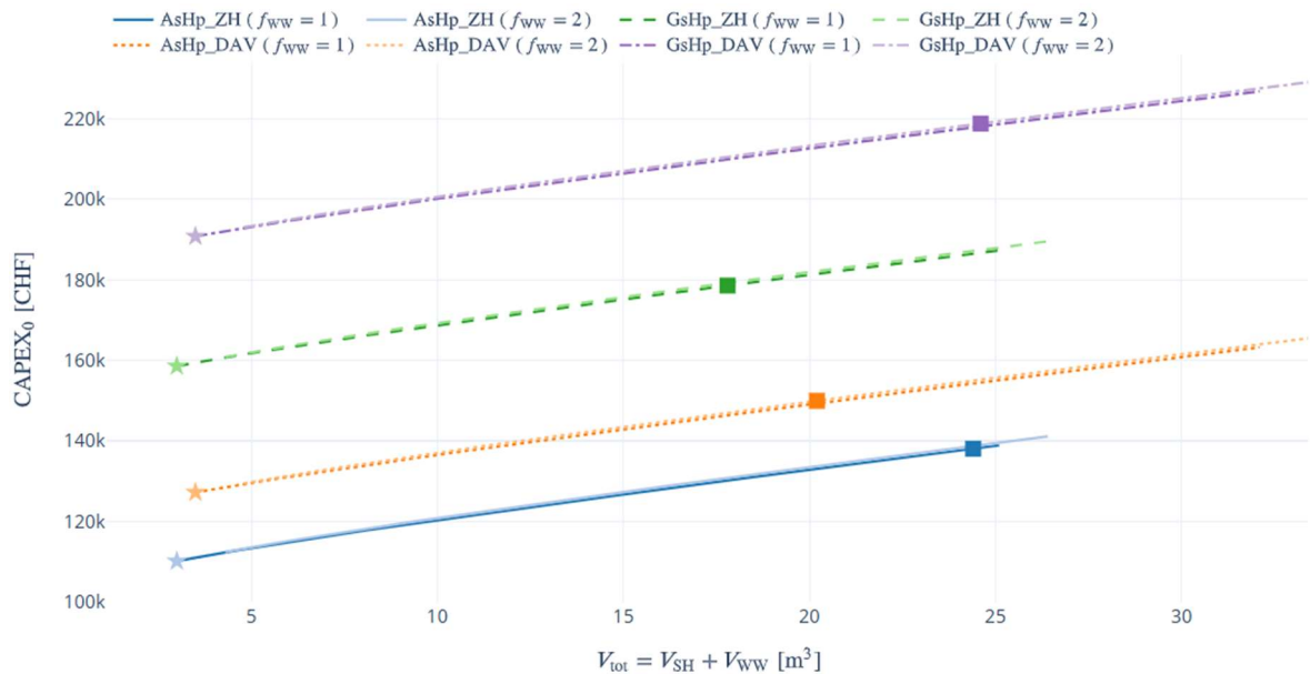
Abbildung 32: MFH25: Darstellung analog zu Abbildung 31
