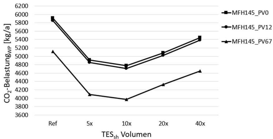
Abbildung 52: Änderung der CO 2 -Belastung der WP vs. Änderung von Pufferspeichergrosse (TES sh ) in Abhängigkeit der PV-Leistung - Gebäude MFH145
