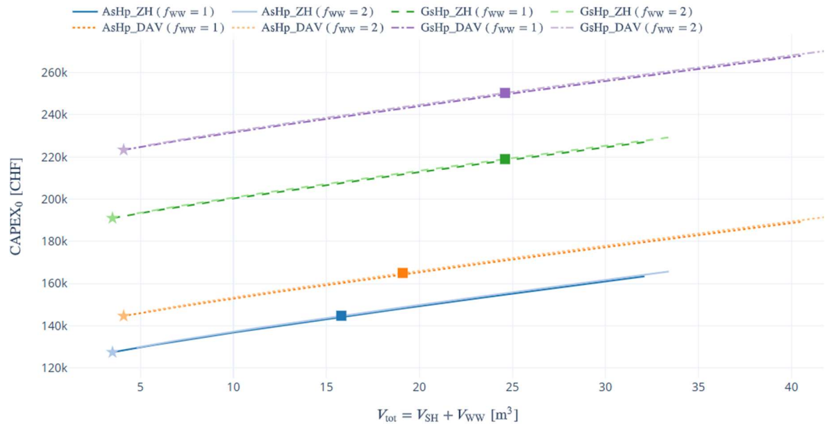
Abbildung 63: MFH45: Total CAPEX in Abhängigkeit des TES-Gesamtvolumens. Linienbänder je Kombination AsHp/GsHp \times ZH/DAV (gleicher Linienstil), Farbe differenziert f_{WW} = 1 und 2. Stern = Referenz-Volumen, Quadrat = Optimum-Volumen (AP3)
