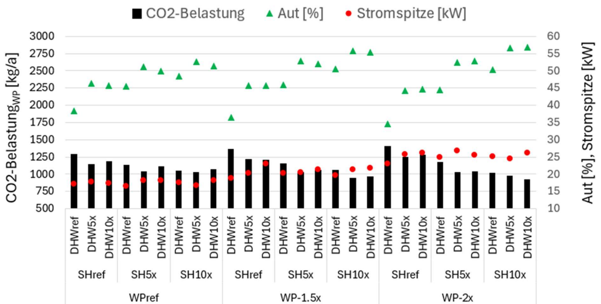
Abbildung 47: CO 2 -Belastung der Wärmepumpe, Autarkiegrad und Stromspitze in Abhängigkeit vom Speichervolumen - Kontrollstrategie "PVEigen max "
