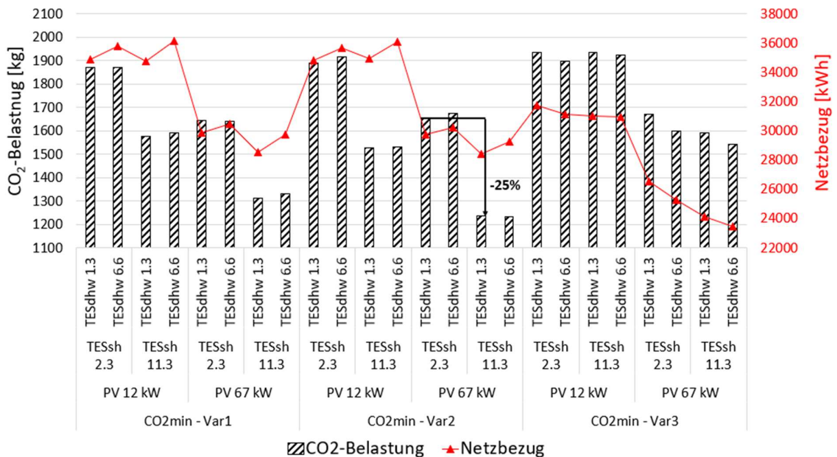
Abbildung 44: Jährliche CO 2 -Belastung (linke Achse) und Netzbezug (rechte Achse) in Abhängigkeit von der Kontrollstrategie, PV-Leistung und Speichervolumen - Simulationsstudie I (Die Speichervolumen sind in m 3 angegeben).
