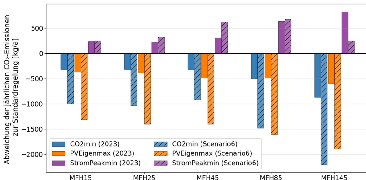
Abbildung 35: Vergleich CO 2 -Emissionen der einzelnen Regelstrategien pro Gebäudestandard. Referenzwerte sind in Tabelle 5 ersichtlich.
