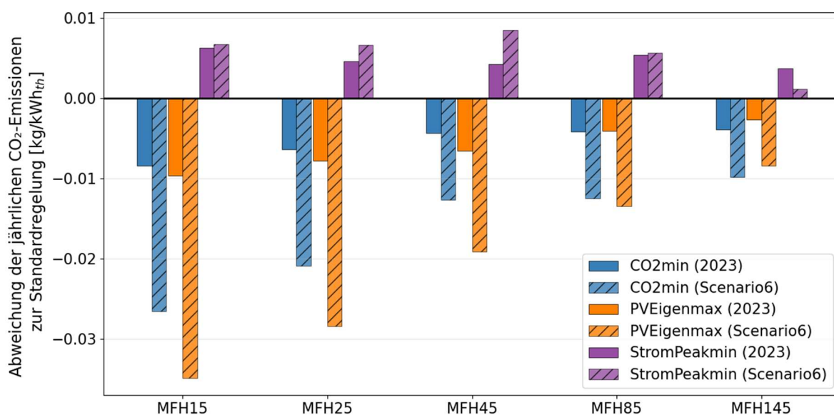
Abbildung 36: Vergleich spezifischen CO 2 -Emissionen pro kWh th der einzelnen Regelstrategien pro Gebäudestandard. Referenzwerte sind in Tabelle 5 ersichtlich.
