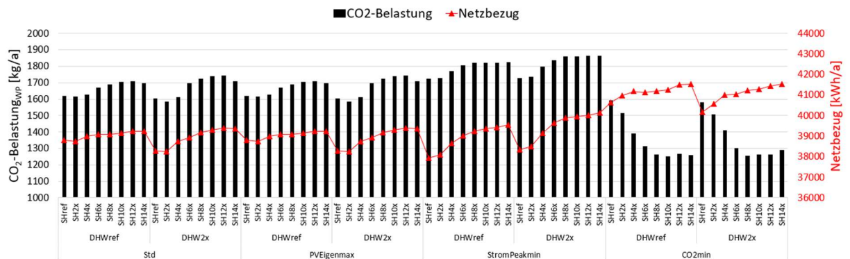
Abbildung 53: CO 2 -Belastung der Wärmepumpe (linke Achse) und Netzbezug (rechte Achse) bei unterschiedlicher Regelstrategie und Speichervolumen – PV-Leistung «PV0» (Fall «MFH25_LWP_SMA_2023»)
