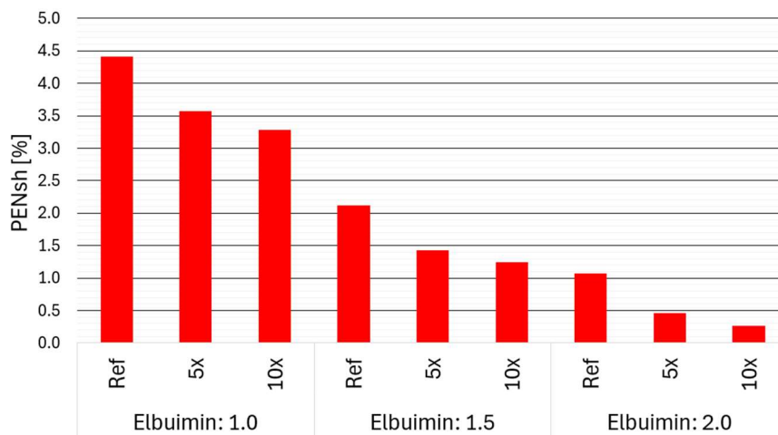
Abbildung 43: PEN_{sh} in Abhängigkeit vom Pufferspeichervolumen und dem Parameter „ EL_{bui,min} “ – „Variante 2“ der Kontrollstrategie «StromPeak min », PV-Leistung von 67 kW, WW-Speichervolumen konstant
