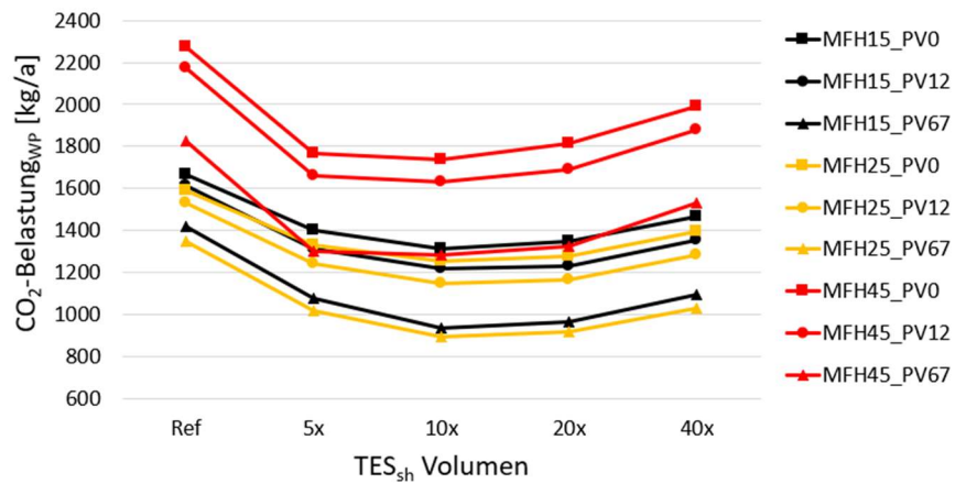
Abbildung 50: Änderung der CO 2 -Belastung der WP vs. Änderung von Pufferspeichergrosse (TES sh ) in Abhängigkeit der PV-Leistung für unterschiedliche Gebäudestandards.
