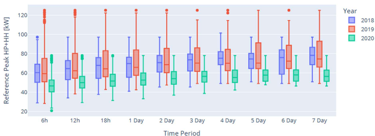
Abbildung 27: Boxplot von der Spitzenlastreduktion verschiedener Jahre und Zeitperioden.
