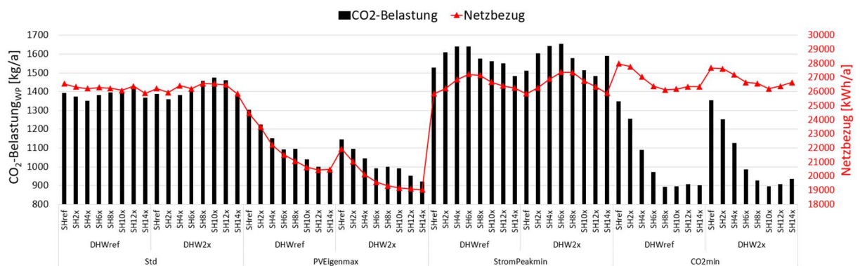
Abbildung 54: CO 2 -Belastung der Wärmepumpe (linke Achse) und Netzbezug (rechte Achse) bei unterschiedlicher Regelstrategie und Speichervolumen – PV-Leistung «PV67» (Fall «MFH25_LWP_SMA_2023»)
