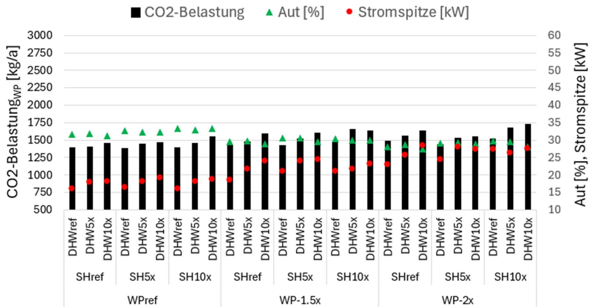
Abbildung 46: CO 2 -Belastung der Wärmepumpe, Autarkiegrad und Stromspitze in Abhängigkeit vom Speichervolumen - Kontrollstrategie "Std"
