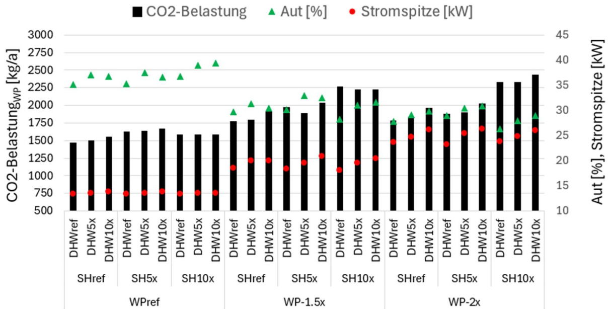
Abbildung 48: CO 2 -Belastung der Wärmepumpe, Autarkiegrad und Stromspitze in Abhängigkeit vom Speichervolumen - Kontrollstrategie "StromPeakmin"
