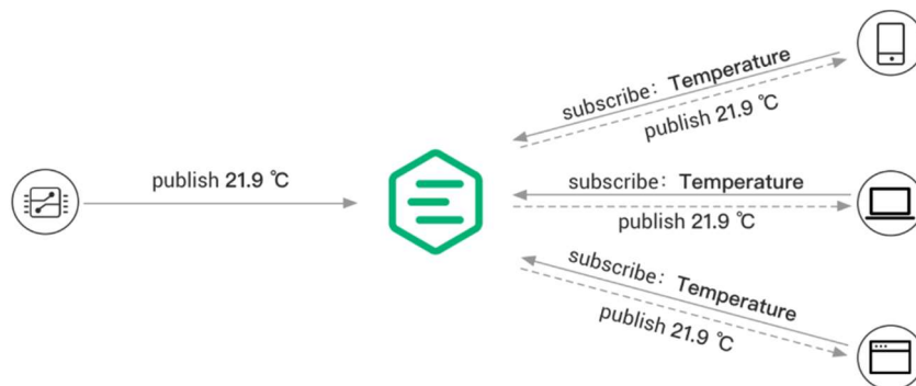
Abbildung 59: Graphische Darstellung des Publish/Subscribe-Modell von MQTT [32]. Das grüne Symbol in der Mitte stellt einen MQTT-Broker dar.
