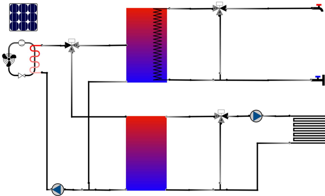
Abbildung 38: Schematische Darstellung des Wärmepumpensystems mit Luft-Wasserwärmepumpe (Quelle: pytrnsysGUI).
