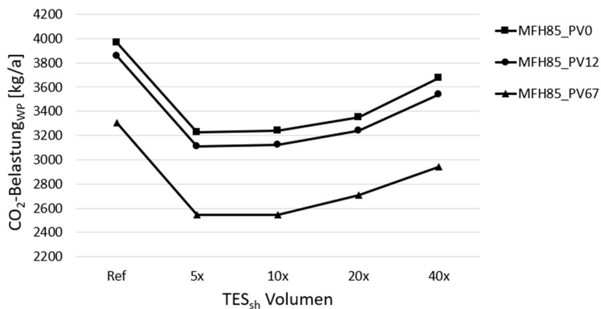
Abbildung 51: Änderung der CO 2 -Belastung der WP vs. Änderung von Pufferspeichergrosse (TES sh ) in Abhängigkeit der PV-Leistung - Gebäude MFH85
