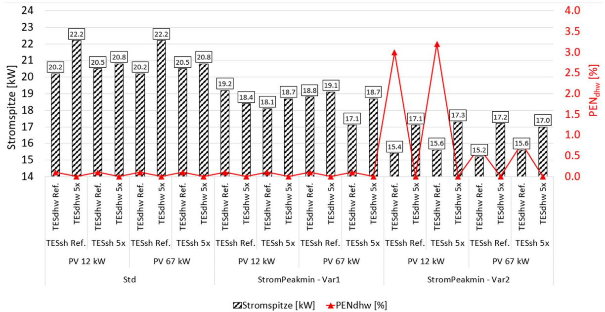
Abbildung 40: Stromspitze (linke Achse) und PEN dhw (rechte Achse) in Abhängigkeit von der Kontrollstrategie, PV-Leistung und Speichervolumen - Simulationsstudie I.
