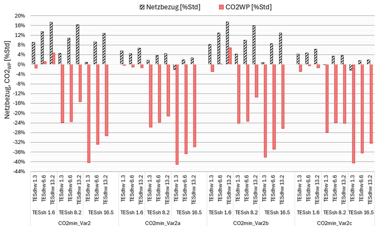
Abbildung 45: Jährliche CO 2 -Belastung der Wärmepumpe und Netzbezug des Gebäudes Variation (im Vergleich zu Kontrollstrategie "Std") in Abhängigkeit von der Kontrollstrategie und Speichervolumen - Simulationsstudie II (Die Speichervolumen sind in m 3 angegeben).
