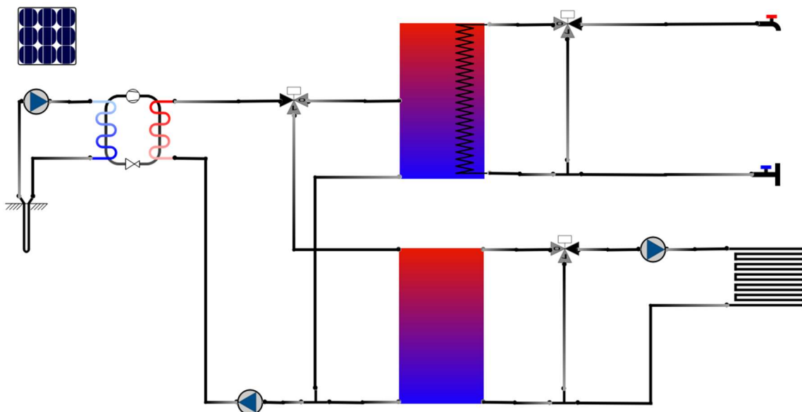
Abbildung 39: Schematische Darstellung des Wärmepumpensystems mit Erdsonden (Quelle: pytrnsysGUI)
