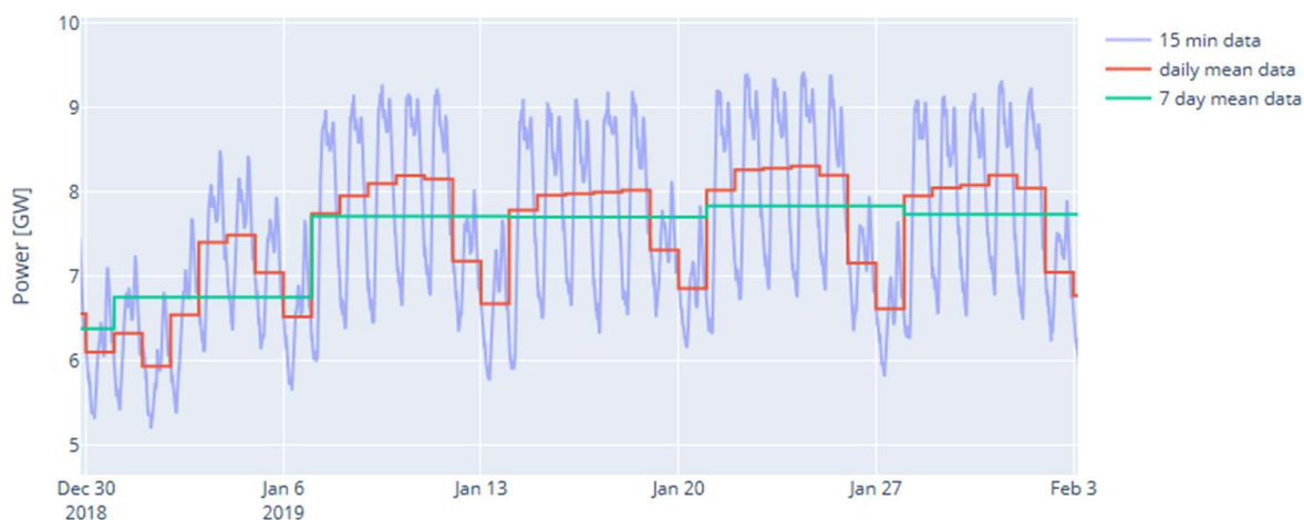
Abbildung 29: Endenergieverbrauch der gesamten Schweiz auf allen Netzebenen über denselben Fünf-Wochen-Zeitraum wie im vorherigen Quartiersbeispiel. Ausgenommen sind hierbei die Energie für Pumpen in Pumpspeicherkraftwerken, der Eigenbedarf von Kraftwerken sowie die Netzverluste.
