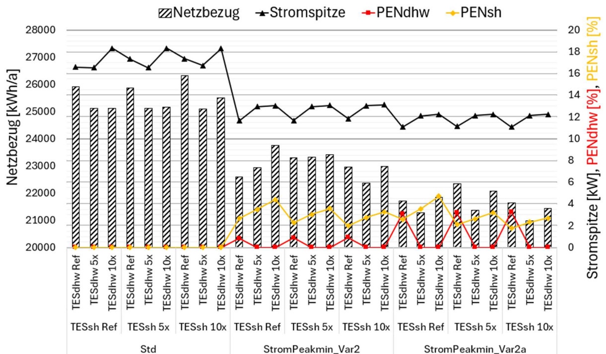
Abbildung 42: Jährliche Netzbezug (linke Achse) und Stromspitze, PENdhw und PENsh (rechte Achse) in Abhängigkeit von der Kontrollstrategie und Speichervolumen - Simulationsstudie II.
