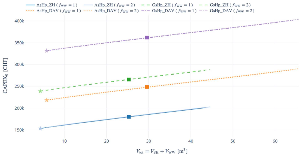
Abbildung 64: MFH85: Total CAPEX in Abhängigkeit des TES-Gesamtvolumens. Linienbänder je Kombination AsHp/GsHp \times ZH/DAV (gleicher Linienstil), Farbe differenziert f_{WW} = 1 und 2. Stern = Referenz-Volumen, Quadrat = Optimum-Volumen (AP3)
