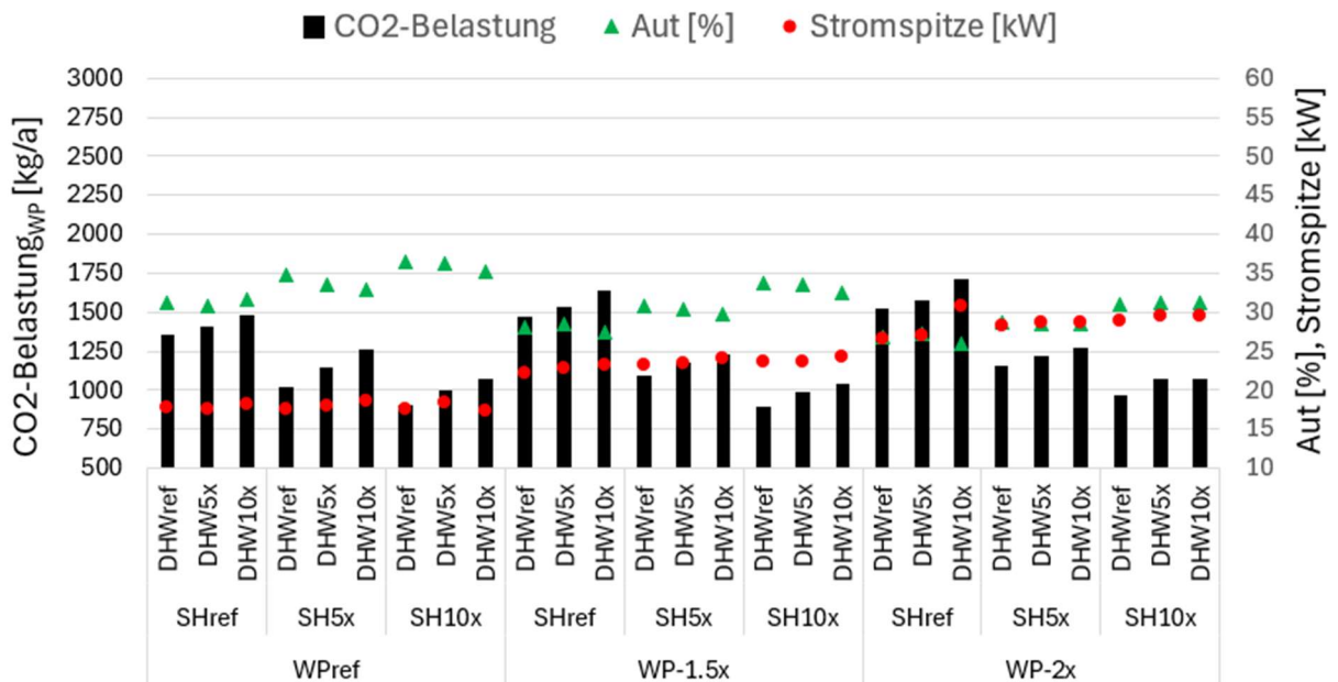
Abbildung 49: CO 2 -Belastung der Wärmepumpe, Autarkiegrad und Stromspitze in Abhängigkeit vom Speichervolumen - Kontrollstrategie "CO 2 min"
