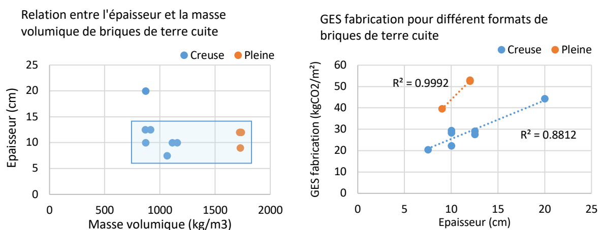
Figure 32 : Relation entre l'épaisseur, la masse volumique et les émissions de GES pour des briques de terre cuite neuves.
