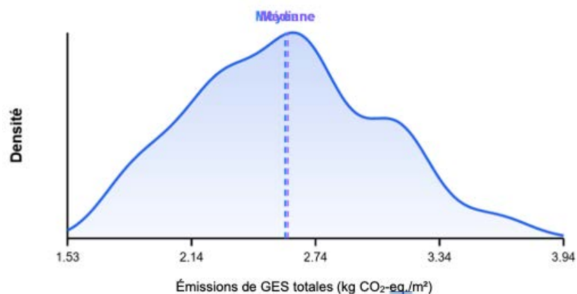
Figure 33 : Distribution de probabilité des émissions de GES totales des briques réemployées (Ecole de Meyrin) avec un échantillon de 384 valeurs potentielles.
