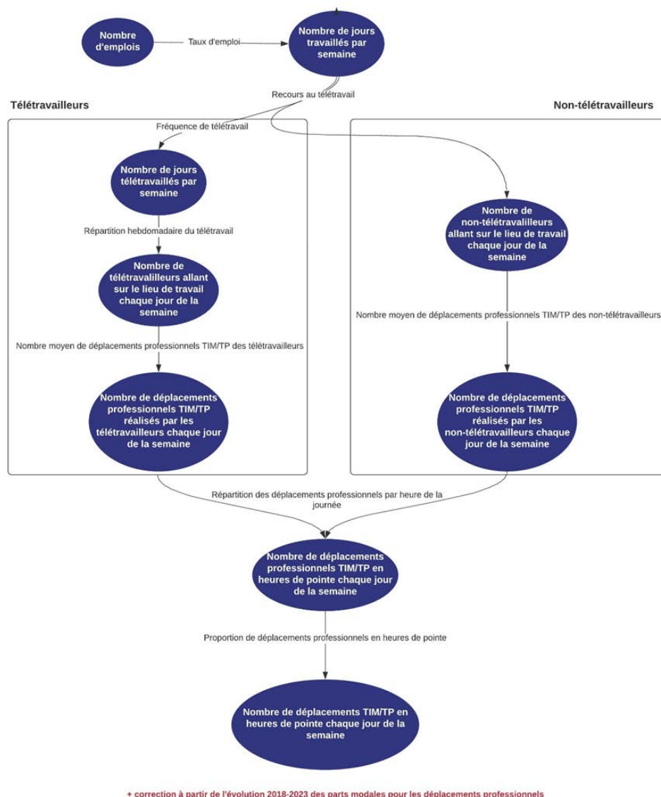
Figure 106: Schéma de la modélisation
