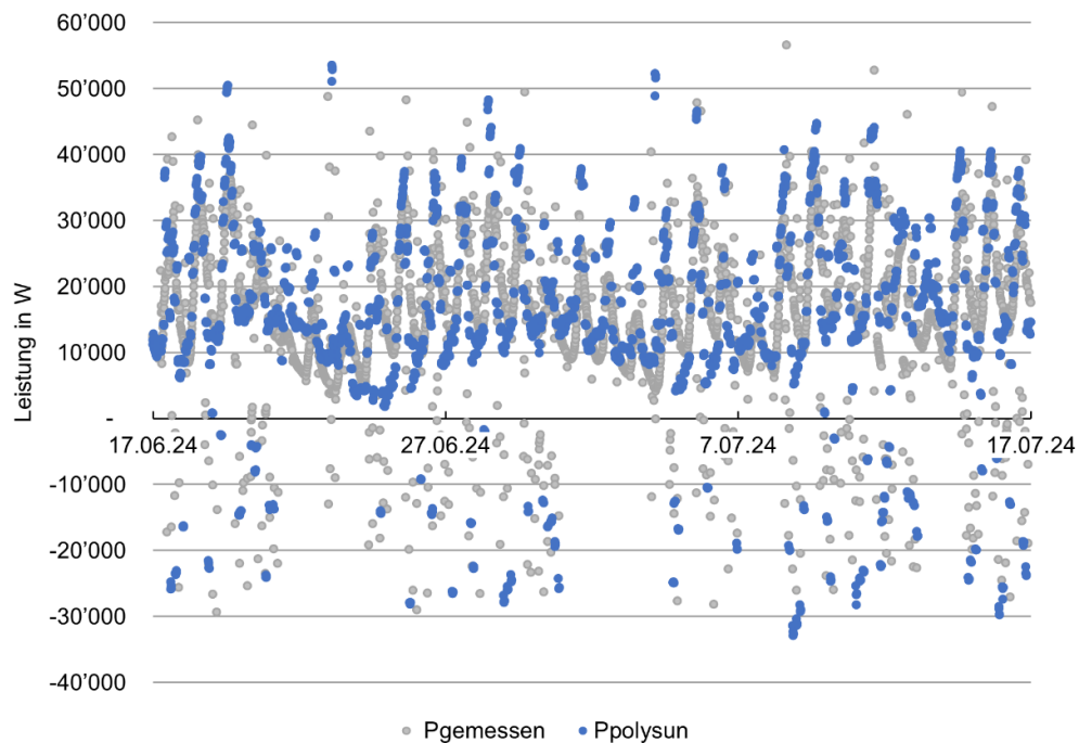
Abbildung 37: Vergleich von gemessener und in Polysun simulierter Leistung des Asphaltkollektors.
