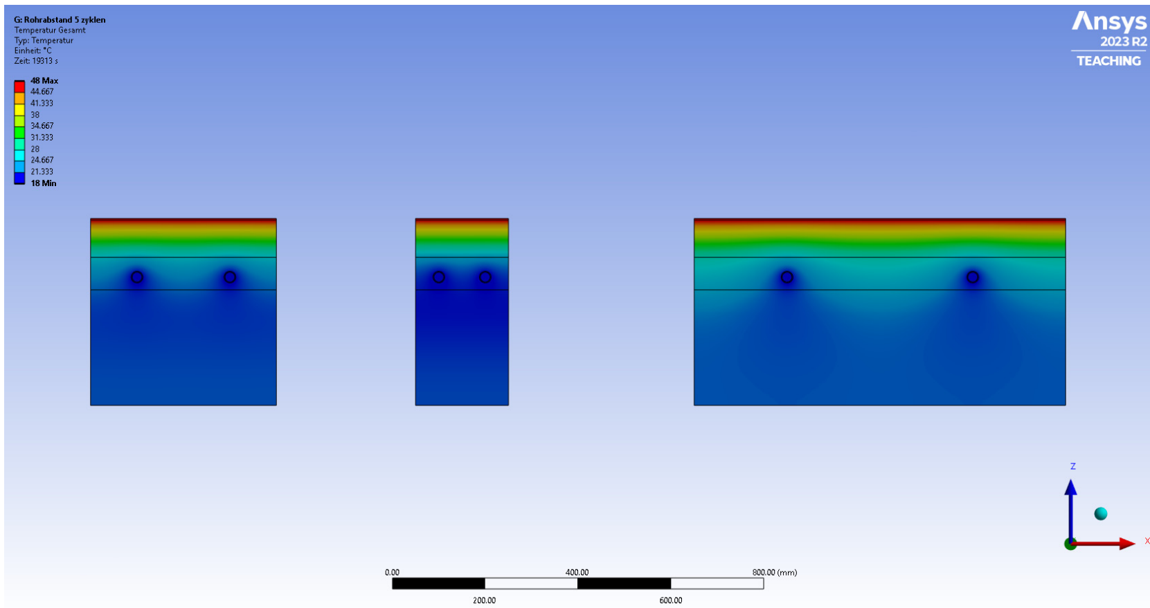
Abbildung 53: Momentaufnahme aus der thermischen Analyse, Asphaltkollektor mit unterschiedlichem Rohrabstand, Mittag
