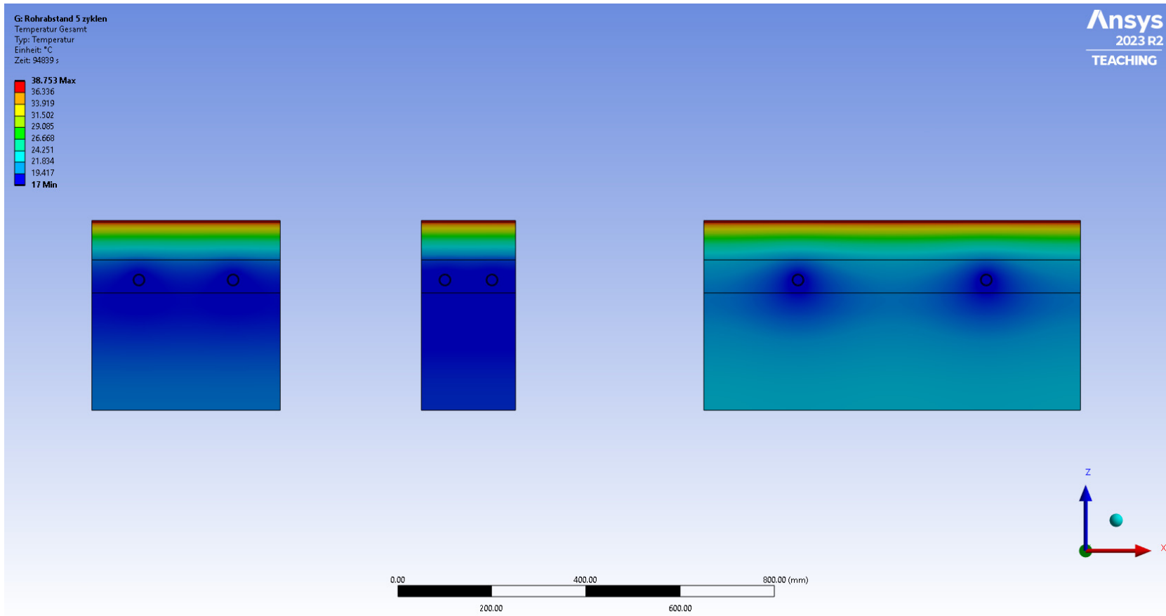
Abbildung 52: Momentaufnahme aus der thermischen Analyse, Asphaltkollektor mit unterschiedlichem Rohrabstand, Aufwärmphase
