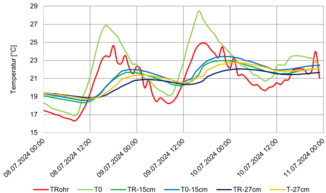
Abbildung 14: Temperaturen am Kollektorrohr, sowie 15 cm und 27 cm darunter sowie Temperatur zwischen zwei Kollektorrohren sowie 15 cm und 27 cm darunter.
