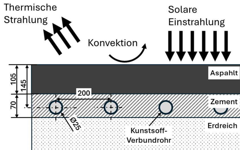
Abbildung 4: Prinzipschema und Schichtdicken Asphaltkollektor
