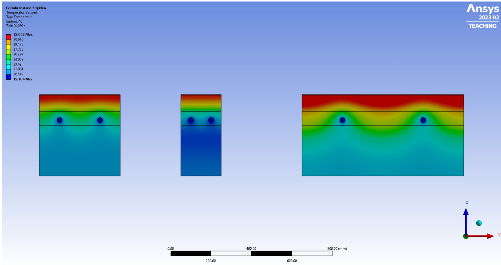
Abbildung 54: Momentaufnahme aus der thermischen Analyse, Asphaltkollektor mit unterschiedlichem Rohrabstand, Abkühlphase
