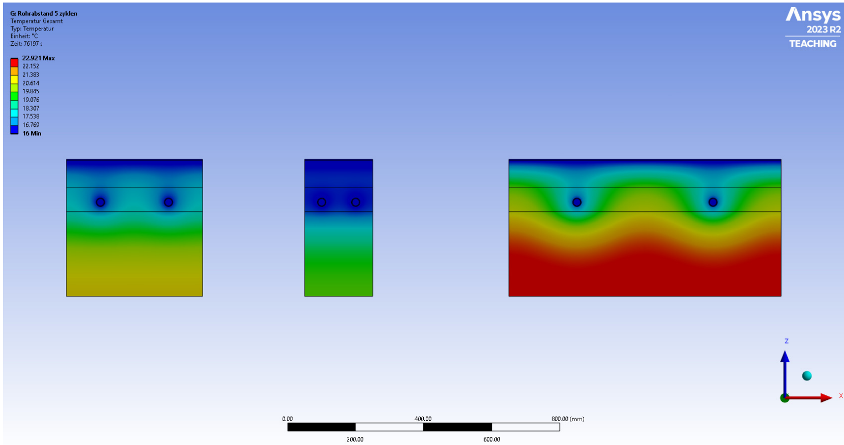
Abbildung 55: Momentaufnahme aus der thermischen Analyse, Asphaltkollektor mit unterschiedlichem Rohrabstand, Asphalt ausgekühlt
