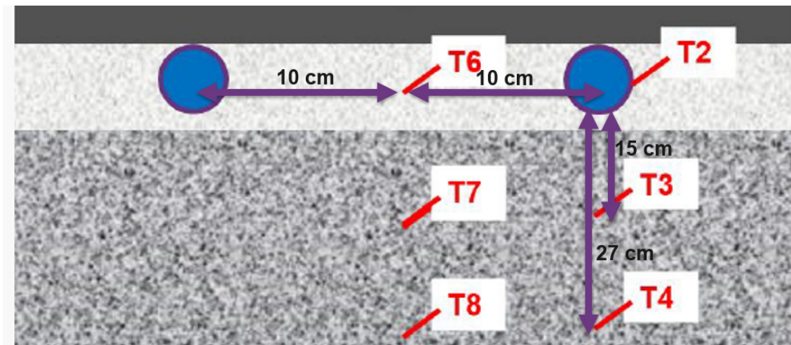
Abbildung 7: Verlegeposition und Abstand der Temperatursensoren in den drei Schichten (von oben nach unten) Asphalt, Zementmörtel und Erdreich/ungebundenen Kiesgemisch
