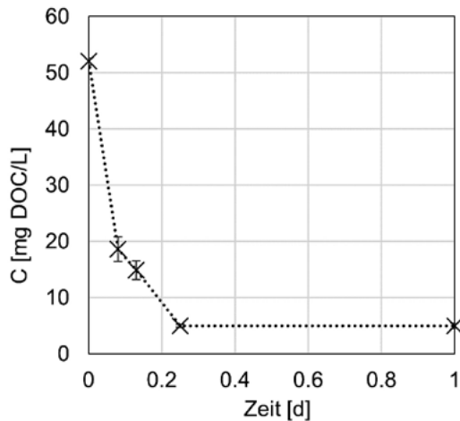
Fig. 4 DOC-Elimination für kommunales Abwasser (filtriert) im AIA-Test.
