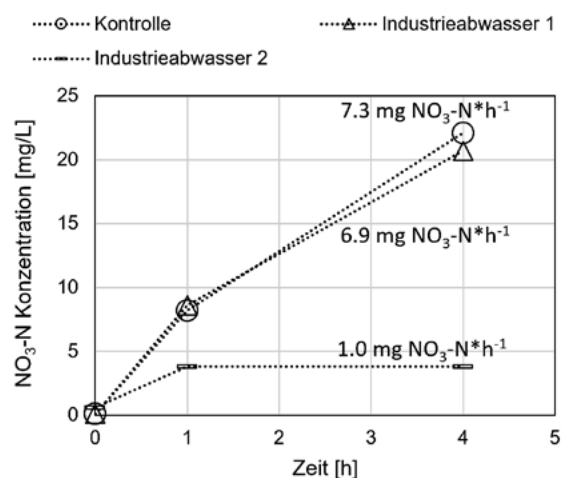
Fig. 6 Verlauf der Nitratkonzentration in der Kontrolle und in zwei Abwasserproben. Die Raten der Nitrifikation sind angegeben. Die Industrieabwasserprobe 2 hemmt die Nitrifikation.
