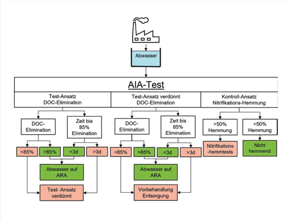
Fig. 7 Interpretation der Resultate aus dem AIA-Test für Abwasserströme, die in einer kommunalen ARA behandelt werden.
