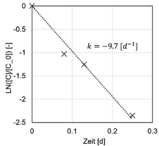
Fig. 5 Berechnete Abbauraten 1. Ordnung k [ \text{d}^{-1} ] für kommunales Abwasser (filtriert) im AIA-Test.
