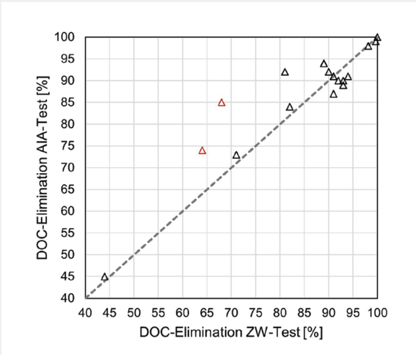
Fig. 2 DOC-Elimination für die Industrieabwasserproben bestimmt mit dem ZW-Test (X-Achse) und dem AIA-Test (Y-Achse). Für die rot markierten Abwasserproben war die DOC-Elimination nach 28 Tagen noch nicht konstant.
