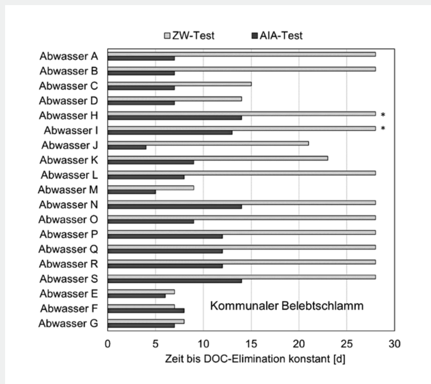
Fig. 3 Benötigte Zeit, um ein Plateau der DOC-Elimination (Abweichung \pm 2\% ) zu erreichen. Die Abwasserproben E, F und G wurden mit nicht adaptiertem Belebtschlamm einer kommunalen ARA getestet. * Für die Abwasserprobe H und I konnte im ZW-Test das Plateau der DOC-Elimination nicht erreicht werden.
