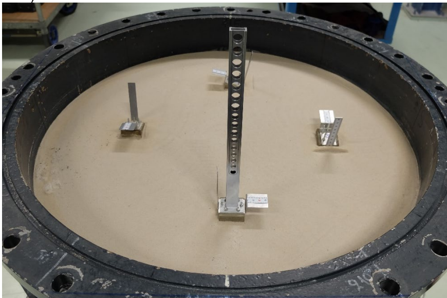
Abbildung unten: Fundament mit Mastaufbau und Laser-Erfassungs-Platten (Bilder HSLU & ETH)
