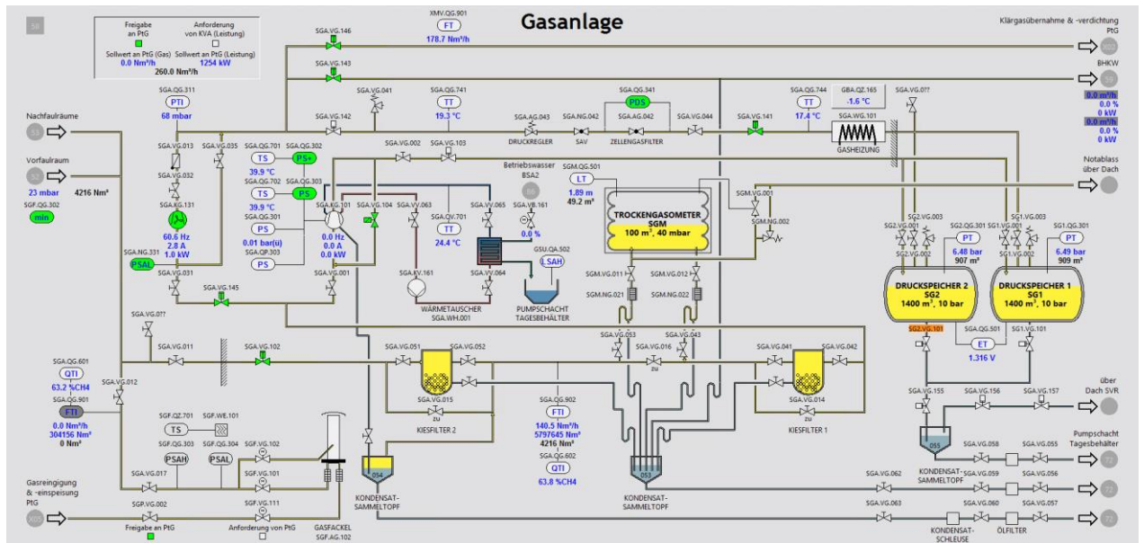
Abbildung 7: ARA-Prozessleitsystem (PLS): Gasanlagen
