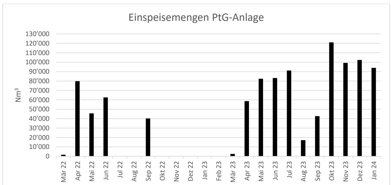
Abbildung 17: Einspeisemengen PtG-Anlage
