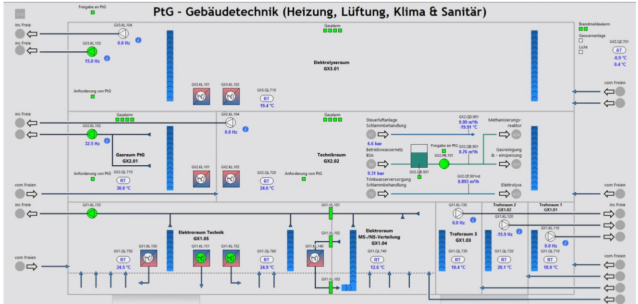
Abbildung 13: ARA-Prozessleitsystem (PLS): Gebäudetechnik PtG
