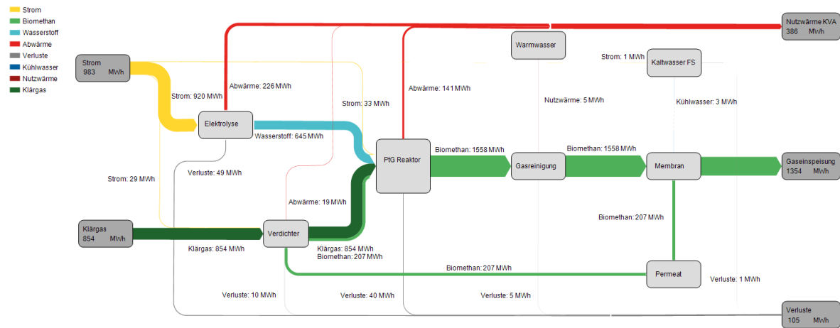
Abbildung 30: Sankeydiagramm Energiebilanz PtG-Anlage Oktober 2023
