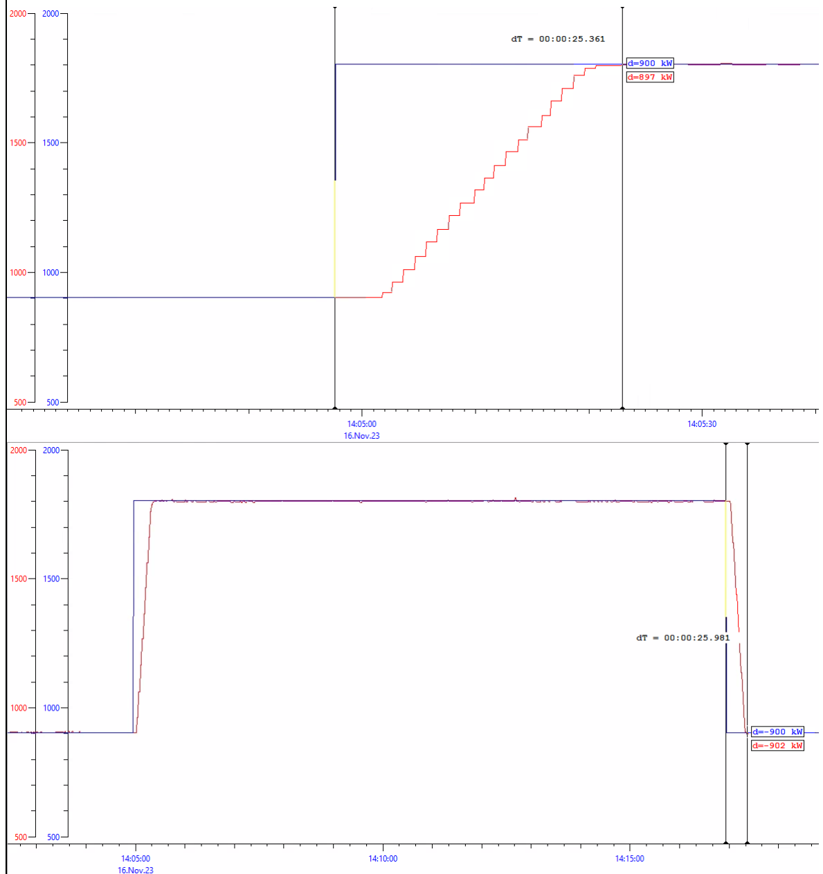
Abbildung 29: PLS-Trend Rampen
