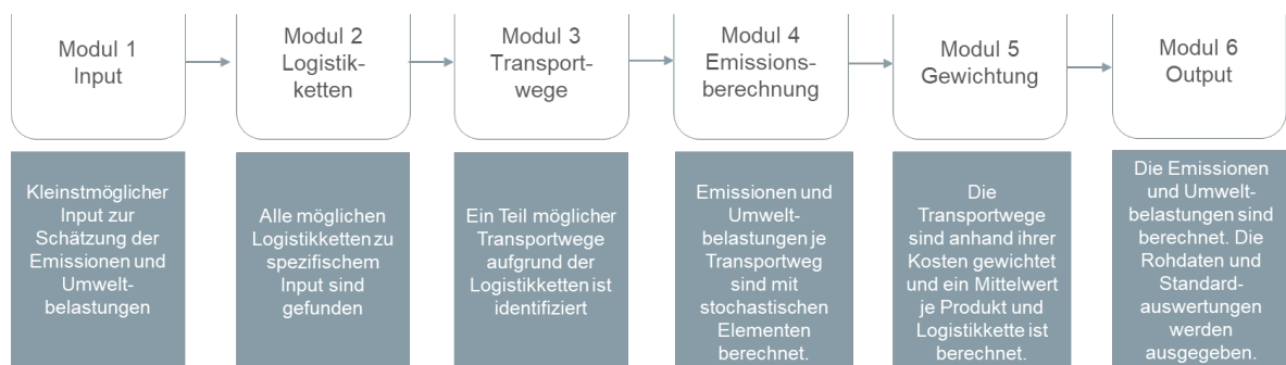
Abbildung 27: Modellstruktur
