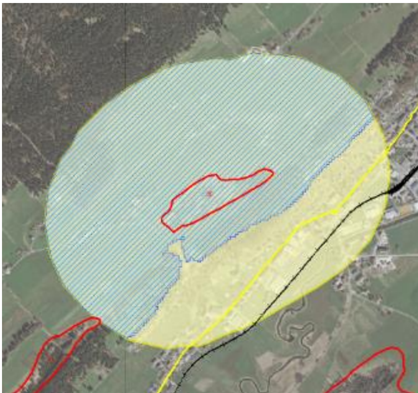
Abbildung 12. Beispiel für ein Objekt der Kategorie 5, wo der Verkehrsweg ausserhalb des hydrologischen Puffers liegt, aber innerhalb des Störungspuffers von <500m.
