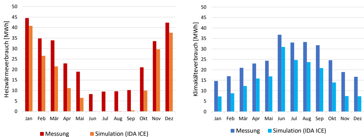
Abbildung 33: Monatliche Energiebilanz des OST-FZ im Vergleich zwischen Messung und Simulation in IDA ICE für die Messperiode Jan-Dez 2021. Es wurden bestmögliche Annahmen zur Nutzung für die Simulationen verwendet (Luftmengen, Raumsolltemperaturen, interne Lasten etc.).
