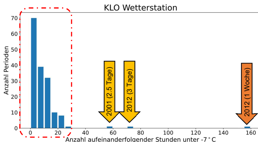
Abbildung 55: Anzahl Kälteperioden in Abhängigkeit der Anzahl Stunden bei welchen die Aussenlufttemperatur unter -7^{\circ}\text{C} fällt für die Klimastation Kloten für die Jahre 2000 – 2022.
