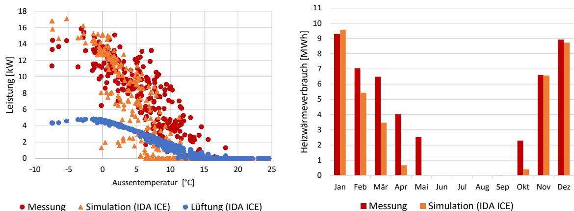
Abbildung 61: Tagesmittelwerte der Heizleistung (links) in Abhängigkeit von der Außenlufttemperatur und der monatliche Heizwärmeverbrauch (rechts) für den Messzeitraum 01.01.2021 bis 31.12.2021. Vergleich der dynamischen Gebäudesimulation (mit bestmöglichen Annahmen nur zur Nutzung) und der tatsächlich gemessenen Leistung und des monatlichen Heizwärmeverbrauchs für das MFH Plattenhof. In der linken Abbildung ist die simulierte Leistung der Luftvorwärmung separat dargestellt. Bei der monatlichen Auswertung (rechts) wurde die Luftvorwärmung nicht berücksichtigt.
