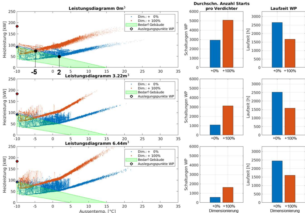
Abbildung 90: Leistungsdiagramm invertergeregelte WP1
