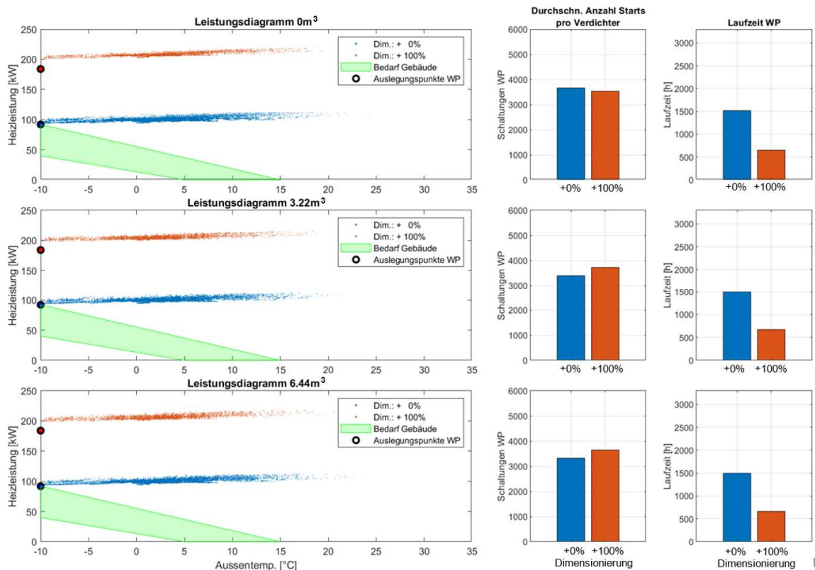
Abbildung 68: Leistungsdigramm WP mit fester Drehzahl und hoher Kapazität im Heizkreis (FBH, TABS).
