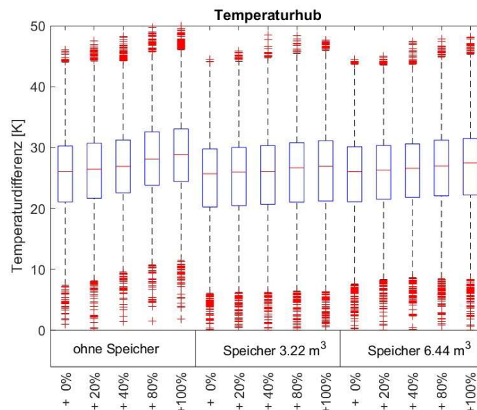
Abbildung 92: Temperaturhub zwischen Quellen- und Senkentemperatur der invertergeregelter WP 2 mit und ohne Speicherintegration.
