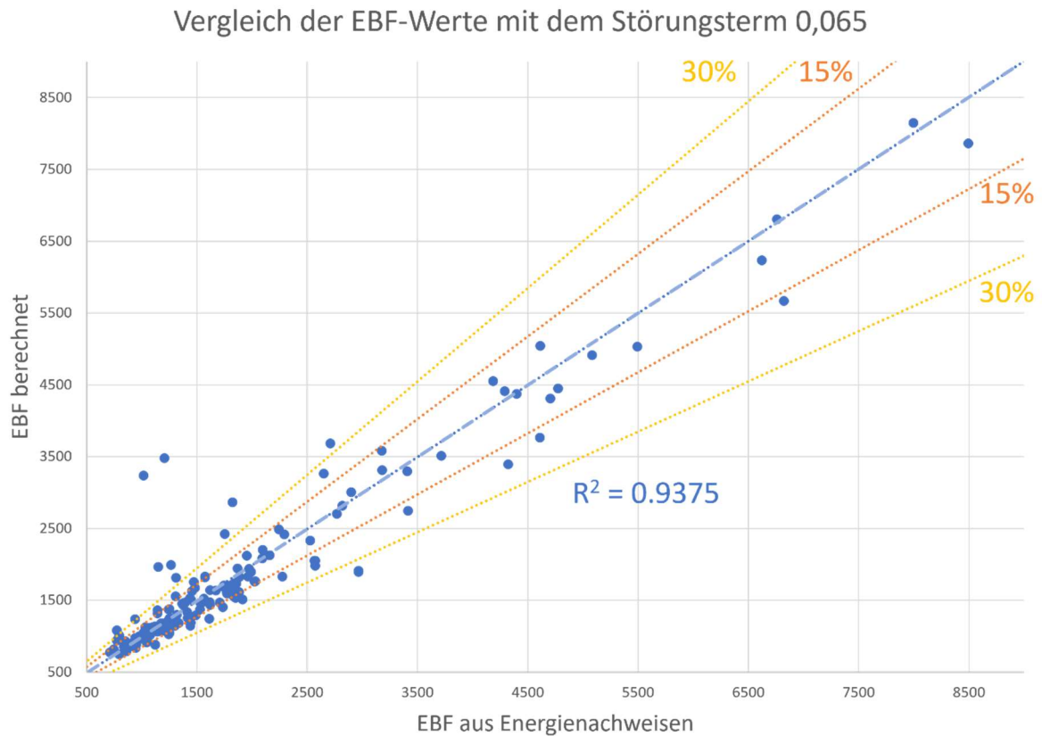
Abbildung 101: Vergleich der EBF-Werte mit dem Störungsterm 0.065, 15- und 30-prozentige Konfidenzintervalle sind eingezeichnet.
