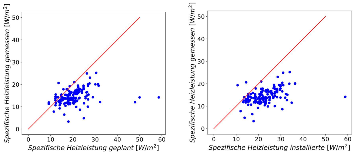
Abbildung 41: Vergleich der geplanten spez. Heizleistung (rechts) und der installierten spez. Heizleistung (links) mit der aus Messdaten ermittelten Heizleistung ( n=155 ). Die rote Linie ist die 1:1-Marke, bei welcher die gemessene und die geplante respektive installierte Leistung übereinstimmen.
