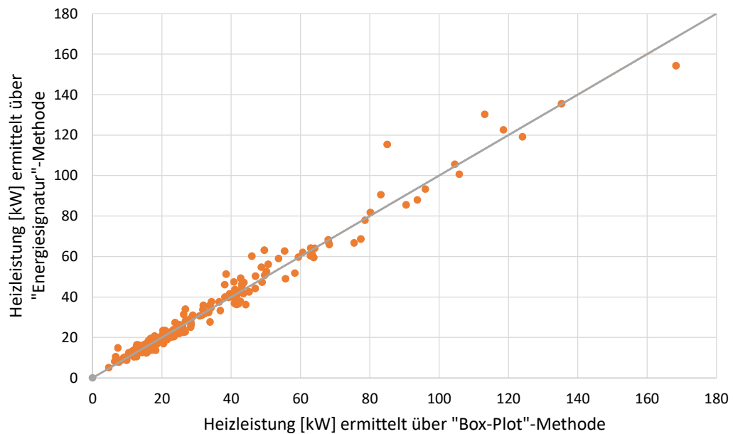
Abbildung 102: Vergleich der unterschiedlichen Methoden zur Ermittlung der Norm-Heizlast aus den EKZ-Messdaten für Stundenmittelwerte .
