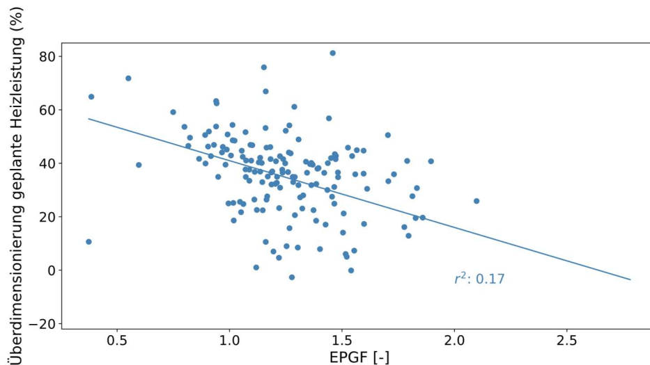
Abbildung 44: Relative Überdimensionierung der installierten Heizleistung in Abhängigkeit vom Energy Performance Gap Factor (n=155).
