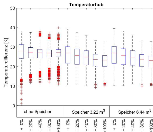
Abbildung 74: Temperaturhub zwischen Quellen- und Senkentemperatur mit und ohne Speicherintegration.
