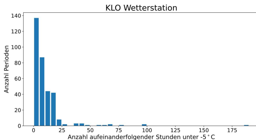
Abbildung 56: Anzahl Kälteperioden in Abhängigkeit der Anzahl Stunden bei welchen die Aussenlufttemperatur unter -5^{\circ}\text{C} fällt für die Klimastation Kloten für die Jahre 2000 – 2022.
