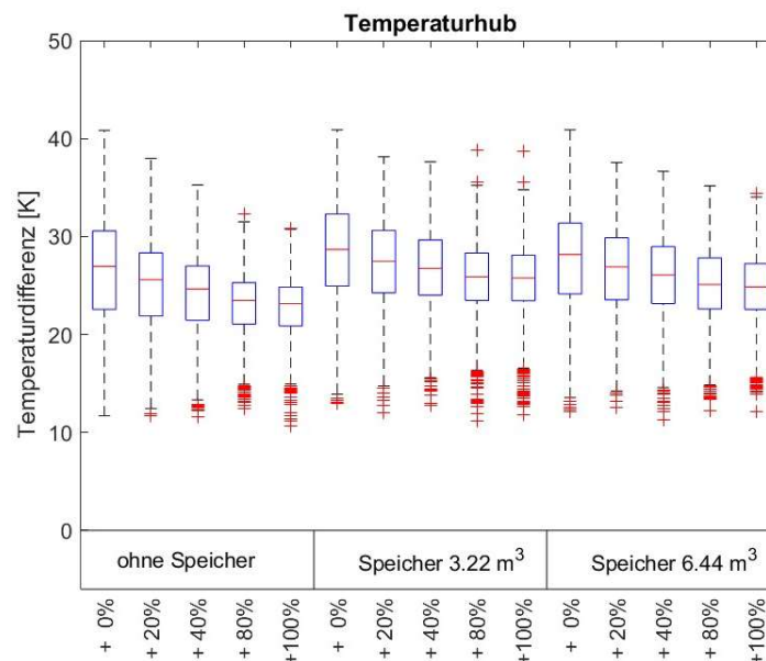
Abbildung 64: Temperaturhub zwischen Quellen- und Senkentemperatur mit und ohne Speicherintegration.
