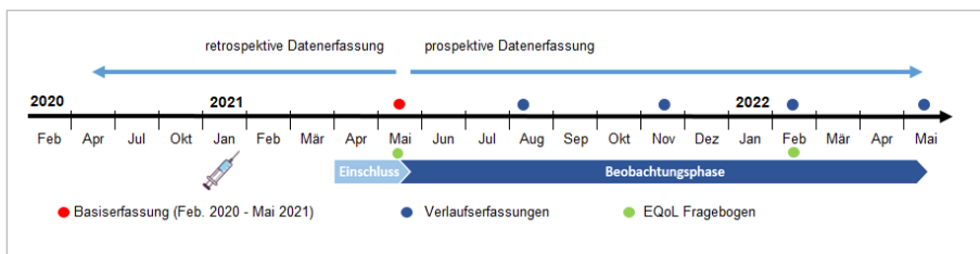
Abb 1: Studienablauf
