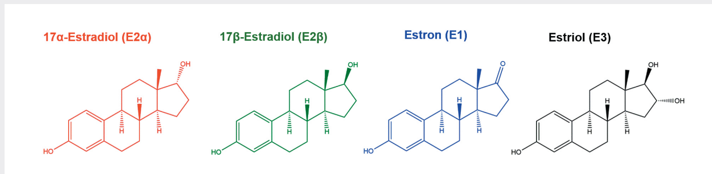
Fig. 1 Strukturformeln der untersuchten natürlichen Estrogene: 17 \alpha -Estradiol (E2 \alpha ; rot), 17 \beta -Estradiol (E2 \beta ; grün), Estron (E1; blau) und Estriol (E3; schwarz).
