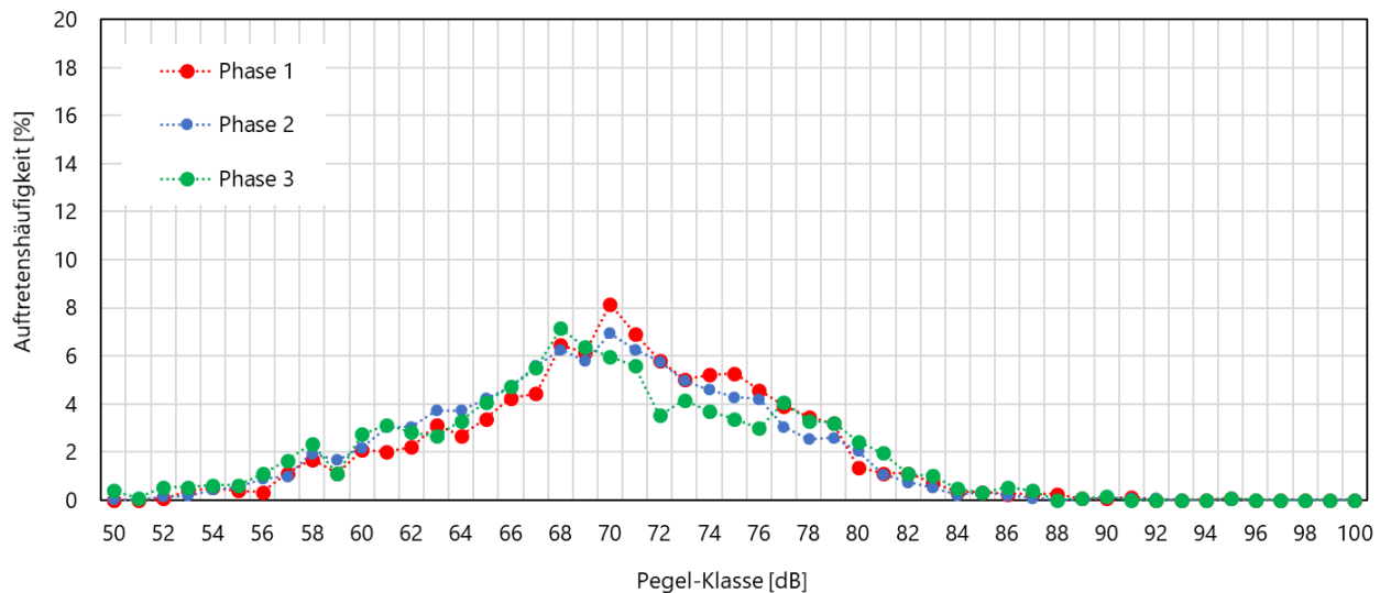
Abbildung 15: Phasenabhängige Pegelverteilung der Motorradereignisse am Messpunkt 1.
