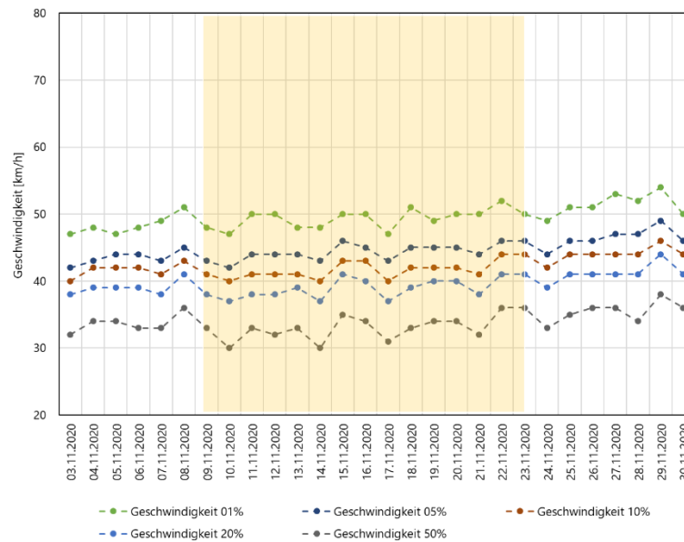
Abbildung 13: Tageweise ausgewertete Geschwindigkeitsperzentilwerte für die PW-Ereignisse am Messpunkt 2. Gelb unterlegt ist die Periode mit eingeschaltetem Display.
