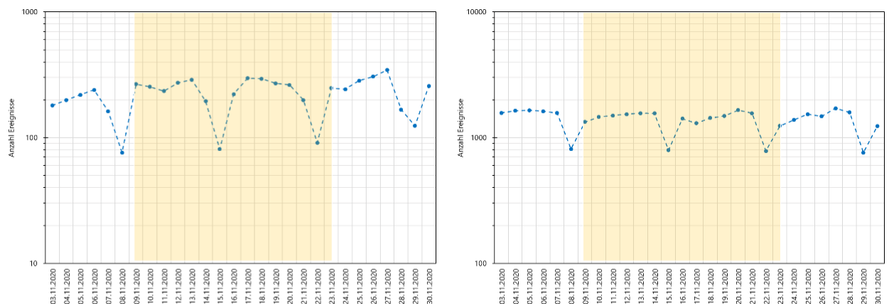
Abbildung 6: Erfasste Tages-Fahrzeugmengen am Messpunkt 2 (links: Motorräder, rechts: Personenwagen).
