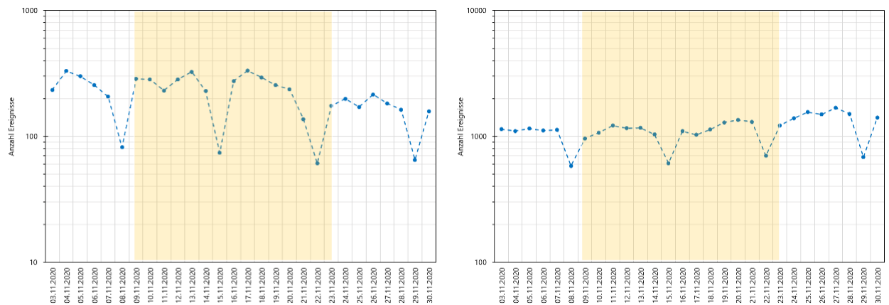
Abbildung 5: Erfasste Tages-Fahrzeugmengen am Messpunkt 1 (links: Motorräder, rechts: Personenwagen).
