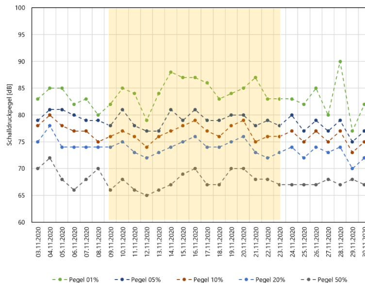
Abbildung 10: Tageweise ausgewertete Schalldruckpegelperzentilwerte für die Motorrad-Ereignisse am Messpunkt 2. Gelb unterlegt ist die Periode mit eingeschaltetem Display.
