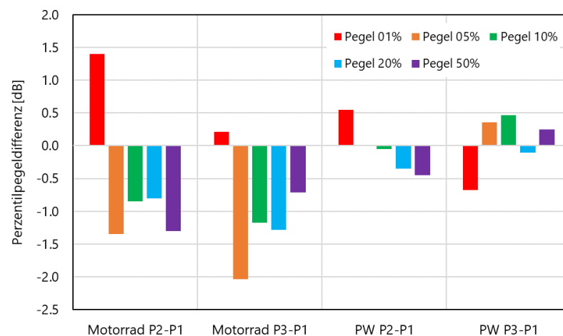
Abbildung 20: Perzentilpegeldifferenzen (1, 5, 10, 20, 50%) am Messpunkt 2 für die beiden Fahrzeugkategorien Motorräder und PW. P2-P1 steht für Phase 2 minus Phase 1, P3-P1 ist Phase 3 minus Phase 1.
