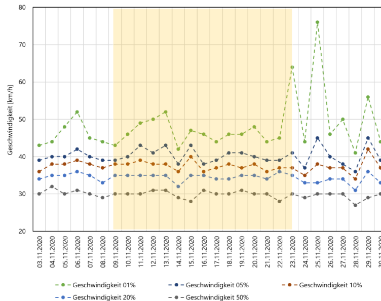
Abbildung 7: Tageweise ausgewertete Geschwindigkeitsperzentilwerte für die Motorrad-Ereignisse am Messpunkt 1. Gelb unterlegt ist die Periode mit eingeschaltetem Display. Lesebeispiel: am 13.11.2020 fuhren die langsamsten 50% der Motorräder höchstens 31 km/h, die 1% schnellsten sind mit mehr als 52 km/h unterwegs. Bei durchschnittlich rund 200 Motorrädern pro Tag wird das 1% Perzentil durch sehr wenige Fahrzeuge bestimmt, sodass hohe Spitzen entstehen können (25.11).
