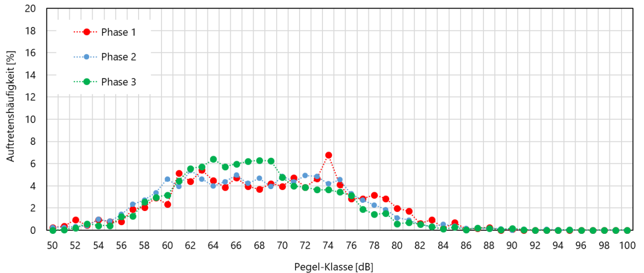
Abbildung 17: Phasenabhängige Pegelverteilung der Motorradereignisse am Messpunkt 2.
