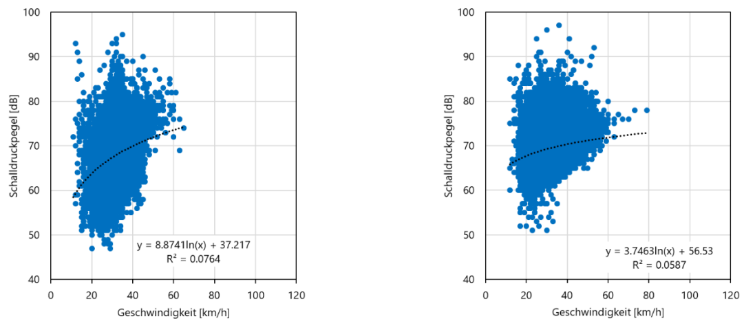
Abbildung 22: X-Y Darstellung der Geschwindigkeit/Schalldruckpegel-Paare am Messpunkt 2 für die Motorräder (links) und PW (rechts).
