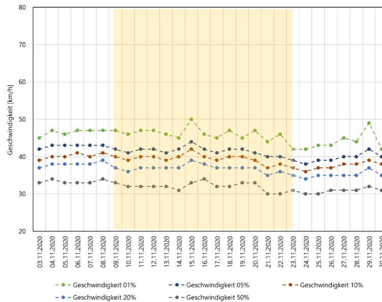
Abbildung 11: Tageweise ausgewertete Geschwindigkeitsperzentilwerte für die PW-Ereignisse am Messpunkt 1. Gelb unterlegt ist die Periode mit eingeschaltetem Display.
