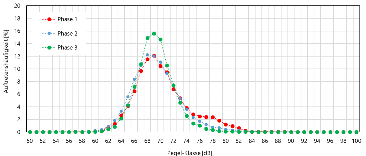
Abbildung 18: Phasenabhängige Pegelverteilung der PW-Ereignisse am Messpunkt 2.
