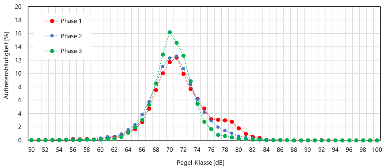
Abbildung 16: Phasenabhängige Pegelverteilung der PW-Ereignisse am Messpunkt 1.
