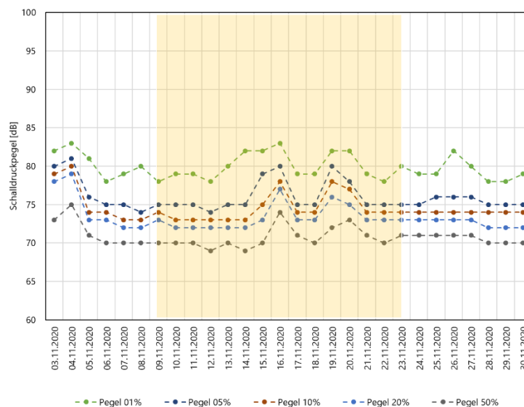
Abbildung 12: Tageweise ausgewertete Schalldruckpegelperzentilwerte für die PW-Ereignisse am Messpunkt 1. Gelb unterlegt ist die Periode mit eingeschaltetem Display.
