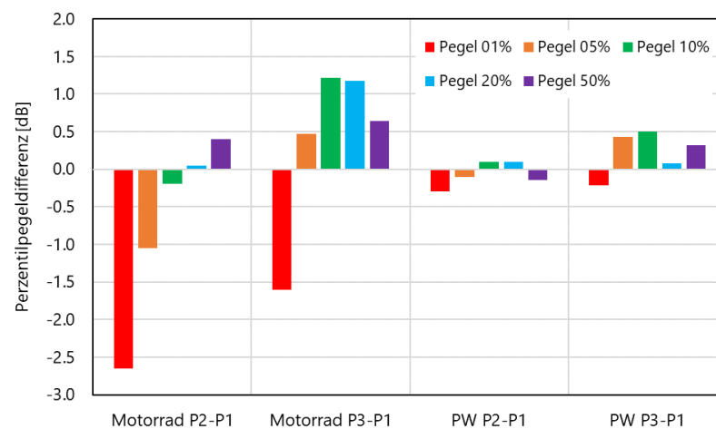
Abbildung 19: Perzentilpegeldifferenzen (1, 5, 10, 20, 50%) am Messpunkt 1 für die beiden Fahrzeugkategorien Motorräder und PW. P2-P1 steht für Phase 2 minus Phase 1, P3-P1 ist Phase 3 minus Phase 1.
