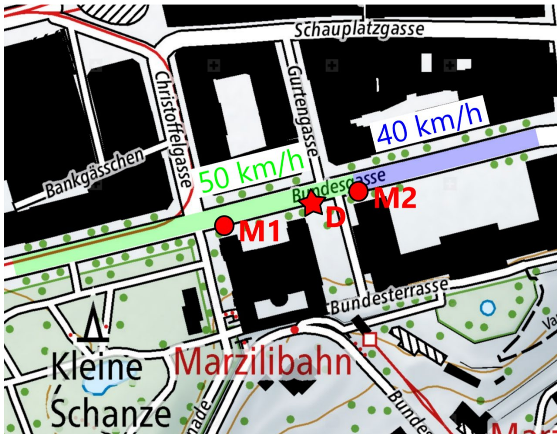
Abbildung 1: Situation der temporären Installation der Messpunkte M1 und M2 sowie des Lärmdisplays D in Bern. Der Messpunkt 1 liegt in einer Tempo 50 Zone, unmittelbar ab Messpunkt 2 ist Tempo 40 signalisiert. Karte: geodata © swisstopo
