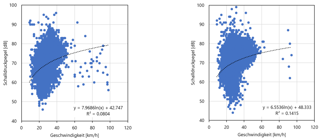
Abbildung 21: X-Y Darstellung der Geschwindigkeit/Schalldruckpegel-Paare am Messpunkt 1 für die Motorräder (links) und PW (rechts).
