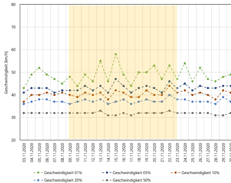
Abbildung 9: Tageweise ausgewertete Geschwindigkeitsperzentilwerte für die Motorrad-Ereignisse am Messpunkt 2. Gelb unterlegt ist die Periode mit eingeschaltetem Display.
