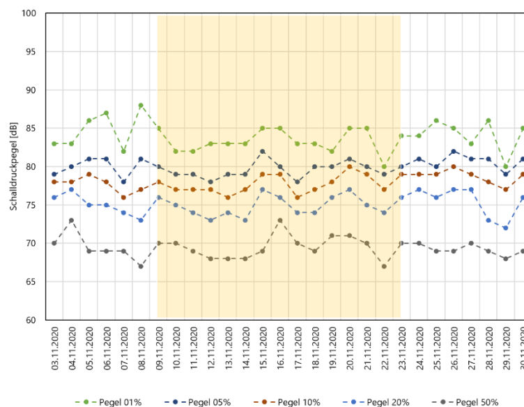
Abbildung 8: Tageweise ausgewertete Schalldruckpegelperzentilwerte für die Motorrad-Ereignisse am Messpunkt 1. Gelb unterlegt ist die Periode mit eingeschaltetem Display. Lesebeispiel: am 13.11.2020 erzeugten die leisesten 50% der Motorräder einen Schalldruckpegel von weniger als 68 dB, die 1% lautesten erzeugten mehr als 83 dB.
