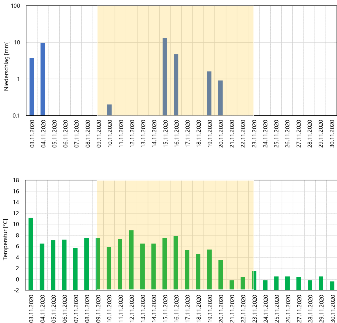
Abbildung 4: Auf jeweils 24 h bezogene Niederschlagsmenge (oben) und Lufttemperatur (unten) gemäss Daten von MeteoSchweiz für die Station Bern-Zollikofen. Gelb unterlegt ist die Periode mit eingeschaltetem Display.
