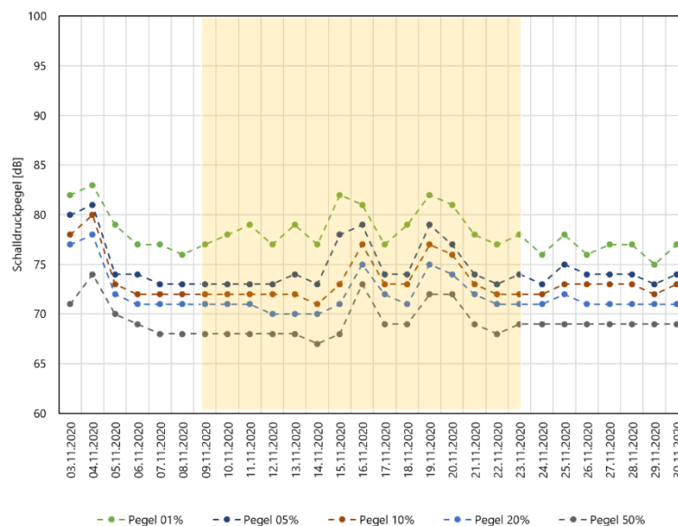
Abbildung 14: Tageweise ausgewertete Schalldruckpegelperzentilwerte für die PW-Ereignisse am Messpunkt 2. Gelb unterlegt ist die Periode mit eingeschaltetem Display.
