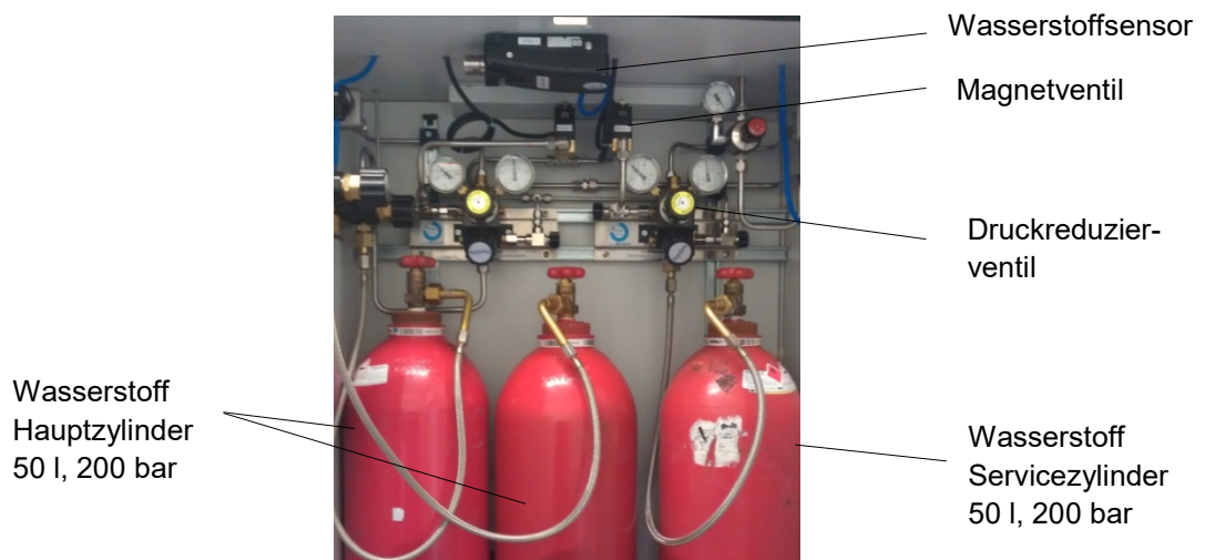
Bild 5: Wasserstoffverteilstation
