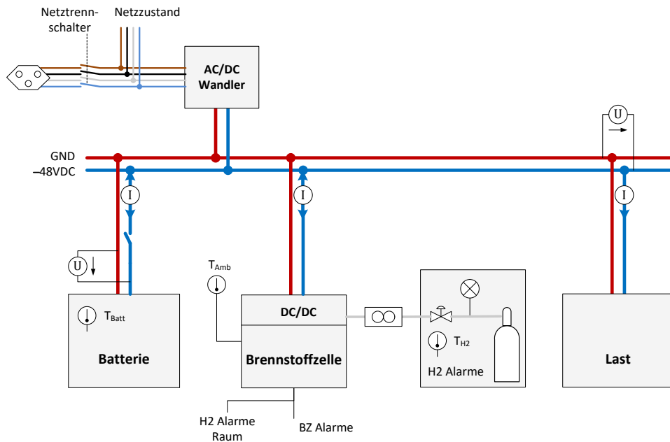
Bild 4: Anlagenschema
