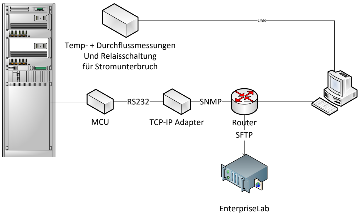
Bild 6: Kommunikationsschema
