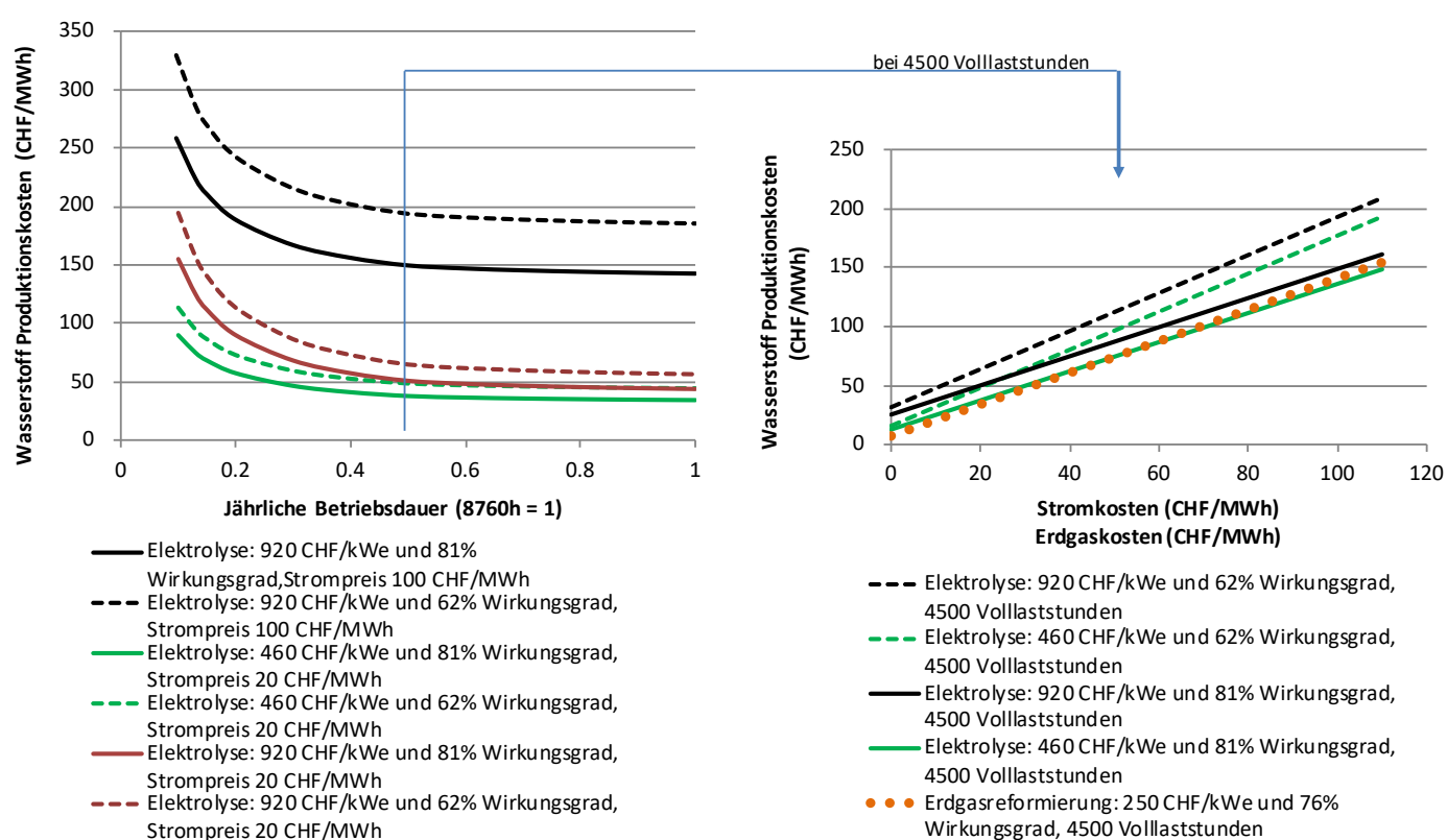
Abbildung 5.2: Wasserstoffproduktionskosten für verschiedene Elektrolyseurkonfigurationen (Investitionskosten, Effizienz) in Abhängigkeit von der jährlichen Elektrolyseurauslastung (linkes Feld) und in Abhängigkeit von den Kosten für die Stromversorgung (rechtes Feld). Zum Vergleich enthält die rechte Abbildung die Wasserstoffproduktionskosten für die Dampfmethanreformierung, die im Verhältnis zu den Kosten für die Erdgasversorgung dargestellt werden. Für alle Technologien zur Wasserstofferzeugung wird ein Zinssatz von 5% angenommen und maximal 90000 Gesamtbetriebsstunden.
