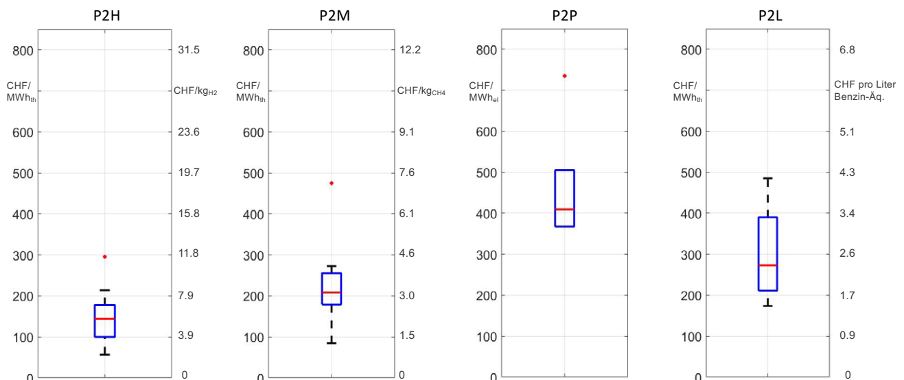
Abbildung 5.1: Verteilung der Kosten für die verschiedenen P2X-Pfade auf der Grundlage aktueller Kosten- und Leistungsdaten (repräsentativ für das Jahr 2015, basierend auf der in dieser Studie verwendeten Literaturquellen, wie im Ergänzungsbericht aufgeführt). Die Boxplots beinhalten den Median (mittleres Quartil innerhalb der Box), 25. und 75. Perzentile. Die Whisker-Plots reichen bis zu den äussersten Datenpunkten ohne Berücksichtigung von Ausreissern; die Ausreisser werden einzeln mit dem Symbol «•» dargestellt. Für die Pfade, die Gas produzieren, basieren die Daten auf Brennwerten; für die P2L-Route stellt die Einheit «CHF pro Liter Benzin-Äquivalent» ein energiebezogenes Mass mit eingeschränkter Vergleichbarkeit zu den Kraftstoffpreisen im Einzelhandel dar, da diese eine erhebliche Steuerkomponente beinhalten.
