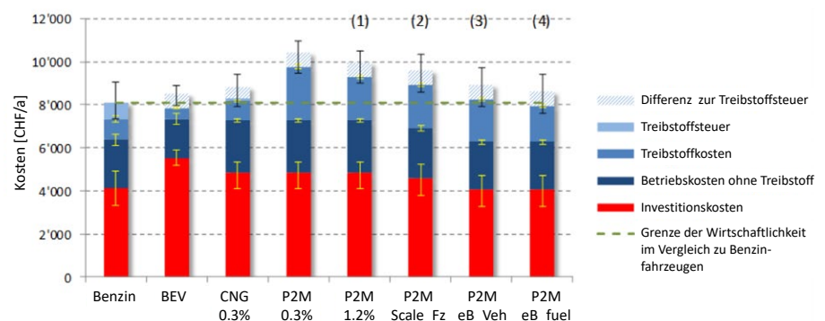
Abbildung 9.2: Berechnung der Gesamtbetriebskosten («total costs of ownership», TCO) für einen benzinbetriebenen Pkw als Referenz, ein BEV und Fahrzeuge mit CNG oder SNG (P2M), beide mit einer Marktdurchdringung von 0.3%. Die P2M-Fahrzeugkosten werden ebenfalls unter Berücksichtigung der folgenden Kostensenkungseffekte berechnet: (1) erhöhte Marktdurchdringung von CNG-Fahrzeugen von 0.3% auf 1.2%; (2) reduzierte Fahrzeugkosten aufgrund gesteigerter Produktionsmengen; (3) Berücksichtigung des Umweltnutzens des Fahrzeugs; (4) Berücksichtigung des Umweltnutzens des synthetischen Kraftstoffs.
