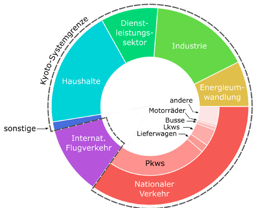
Abbildung 3.1: CO 2 Emissionen in der Schweiz (2015) nach Sektoren [9].
