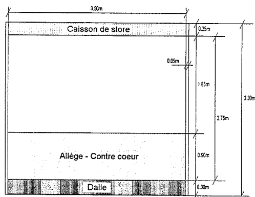
Coupe de la façade double-peau avec contre-cœur
