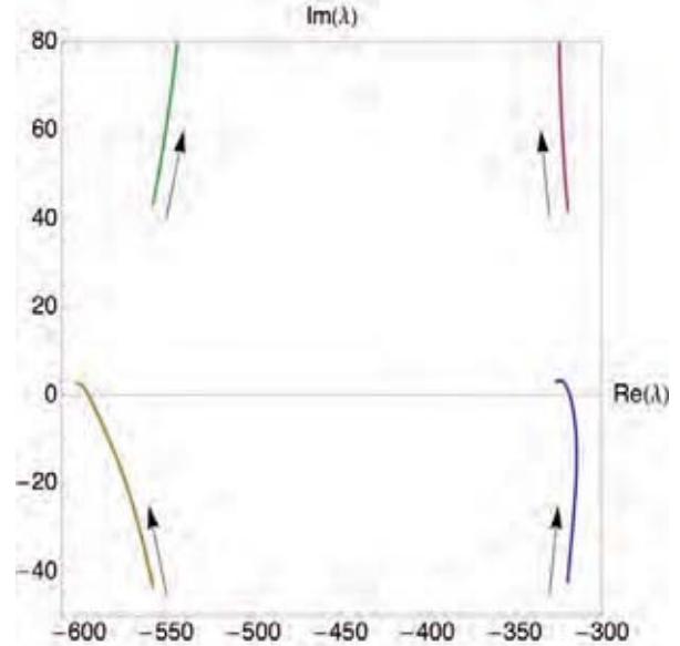
Figur 4 Die Trajektorie der beiden niedrigsten komplexen Eigenwerte als Funktion einer von -6.5 bis -6.556 variierenden Permeabilität t . Die Pfeile geben die Richtung des steigenden Imaginärteils der Permeabilität t an.
