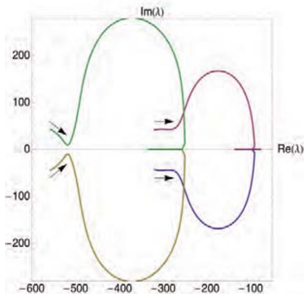
Figur 3 Die Trajektorie der beiden niedrigsten komplexen Eigenwerte als Funktion einer von -6.5 bis -4.5 variierenden Permeabilität t . Die Pfeile geben die Richtung der steigenden Permeabilität t an.
