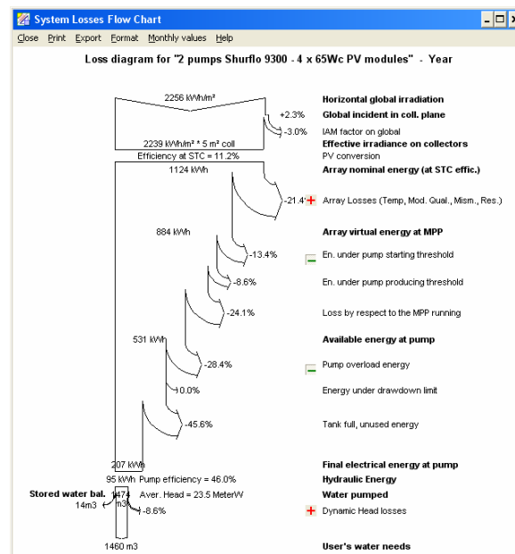
Fig 7. : Simulation détaillée: diagramme des pertes
