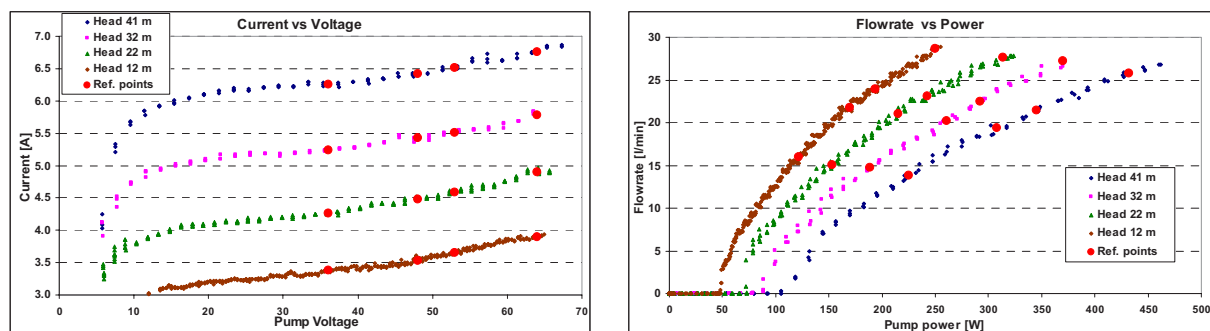
Fig 2.: Mesures de la pompe Watermax BU, avec points de référence à tensions fixes.
