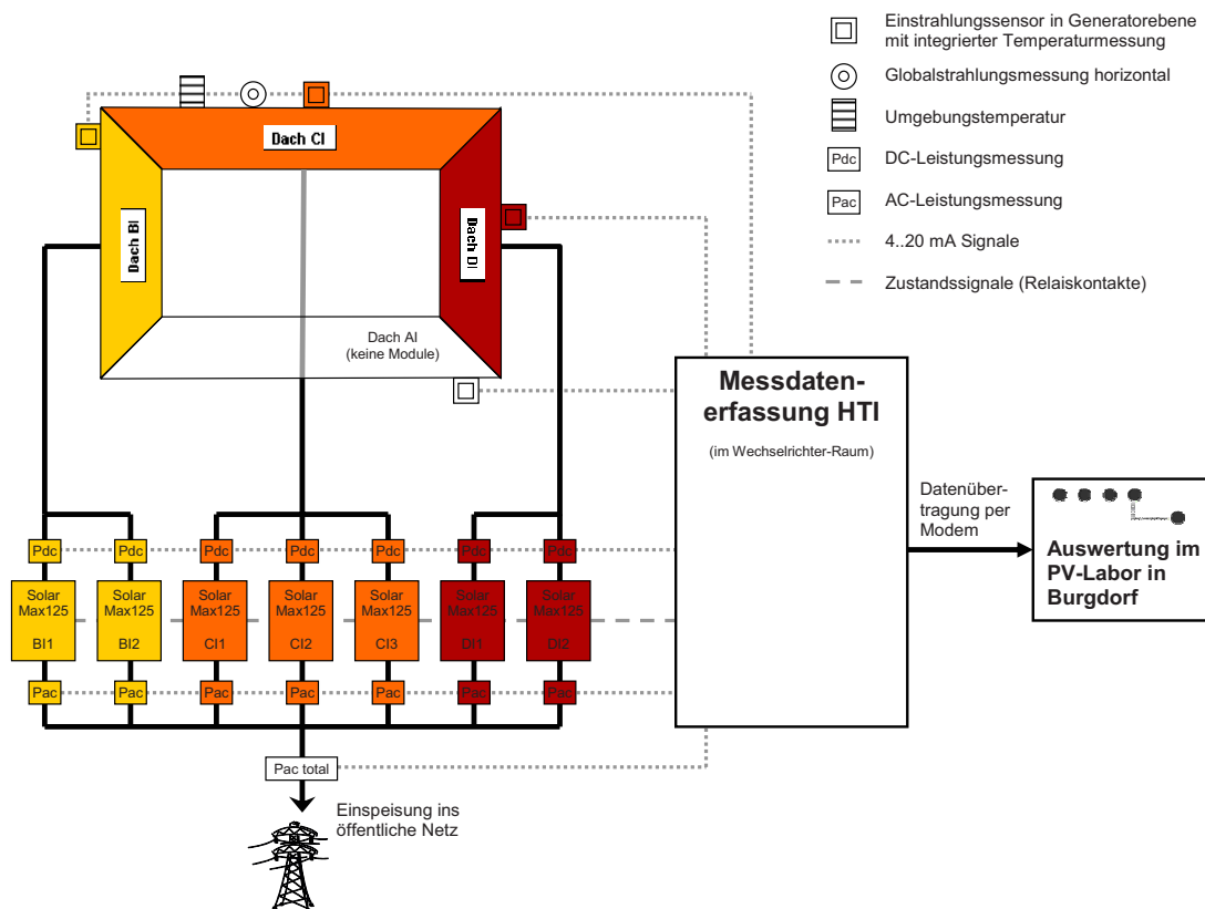
Bild 4: Blockschaltbild der Datenerfassung der PV-Anlage Wankdorf (Stade de Suisse)
