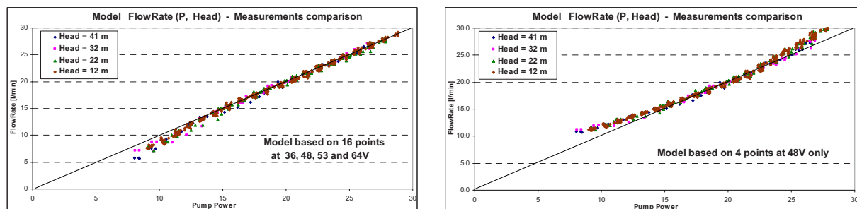
Fig 3.: Comparaison du débit simulé avec les valeurs mesurées, pour les données ci-dessus
