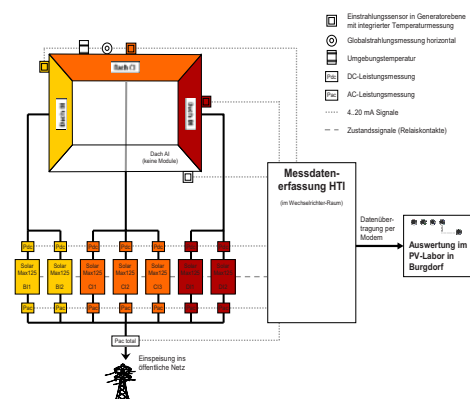
Figur 3: Blockschaftscheina Stade de Suisse (Bildquelle HTI Burgdorf)
