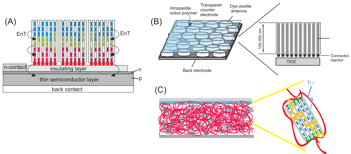
Figur 4) Prinzip der Dünnschicht-Antennen-Solarzellen. (A) sensibilisierte Festkörper-Solarzelle, (B) sensibilisierte Farbstoff-Solarzelle und (C) sensibilisierte Plastik-Solarzelle.
