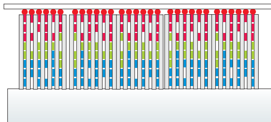
Figur 5) Arbeitsschritte zum Aufbau einer sensibilisierten Festkörper-Antennen-Solarzelle. Dazu gibt es einen Patentanspruch [16].
