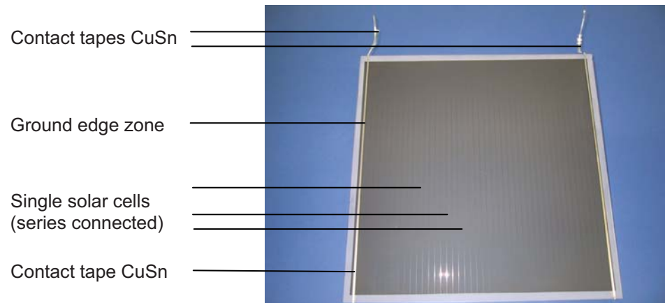
Fig. 1 CIGS solar module 30 x 30 cm 2
