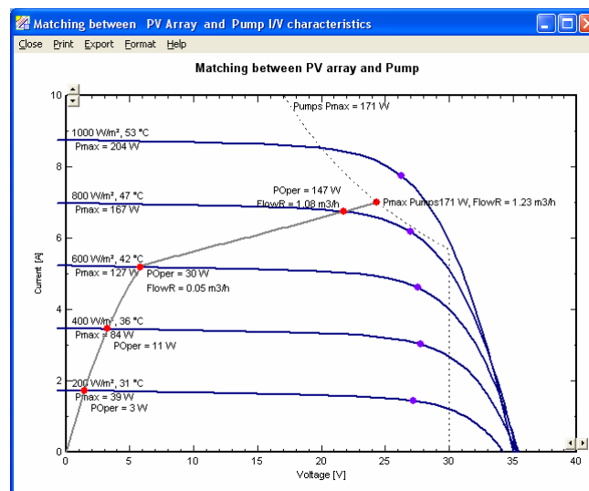
Fig 6.: Aide au dimensionnement électrique pour les systèmes à couplage direct
