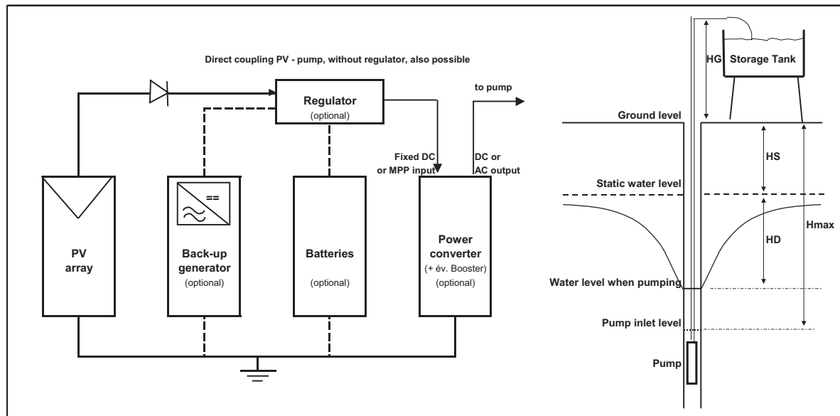
Fig 1.: Schéma global d'un système de pompage – Avec quelques options possibles pour la simulation
