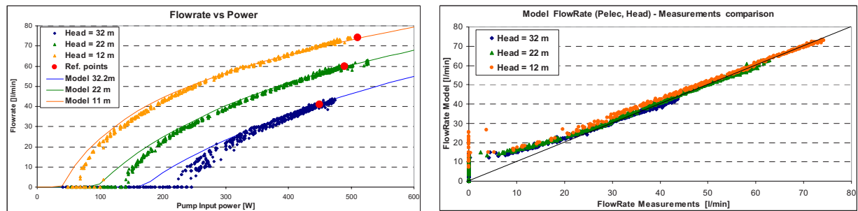
Fig 4.: Pompe centrifuge: modélisation selon 3 points de fonctionnement (Puissance, Débit, Pression) à tension nominale (78V).
