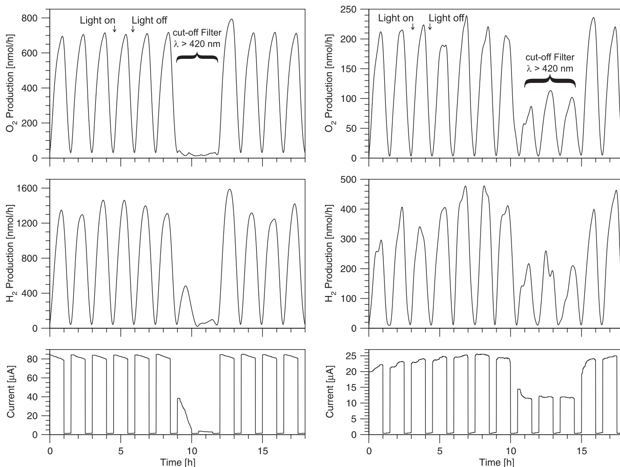
Figur 1) O 2 und H 2 Produktion zusammen mit dem Photostrom für eine Schicht aus TiO 2 Nanoröhren als Photoanode in Kombination mit einer Pt Katode und einer Solarzelle aus amorphem Silizium.
