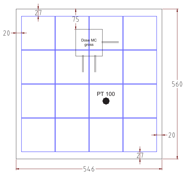
Abbildung 1: Modul layout
