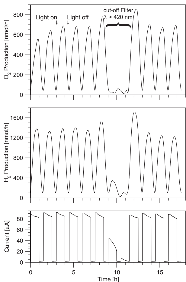
Figur 3) O 2 und H 2 Produktion zusammen mit dem Photostrom für eine Schicht aus TiO 2 Nanoröhren beladen mit Ag/AgCl als Photoanode in Kombination mit einer Pt Katode und einer Solarzelle aus amorphem Silizium.
