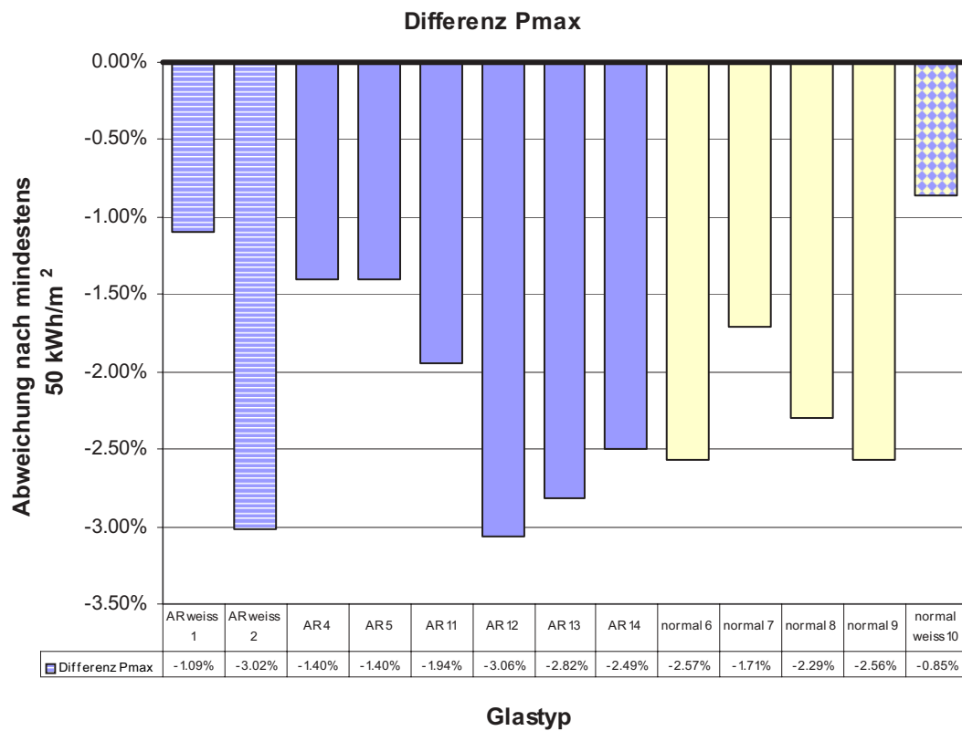
Abbildung 3 : relative Leistungsabnahme nach mindestens 50kWh/m 2 Exposition im Freiland
