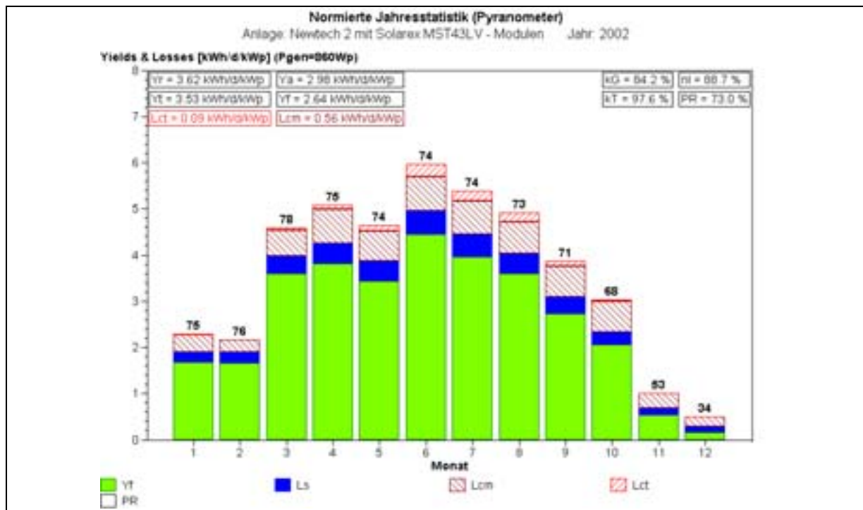
Bild 4: Normierte Jahresstatistik 2002 der a-Si-Tandem-Anlage Newtech 2 mit BP Solarix MST43LV.
