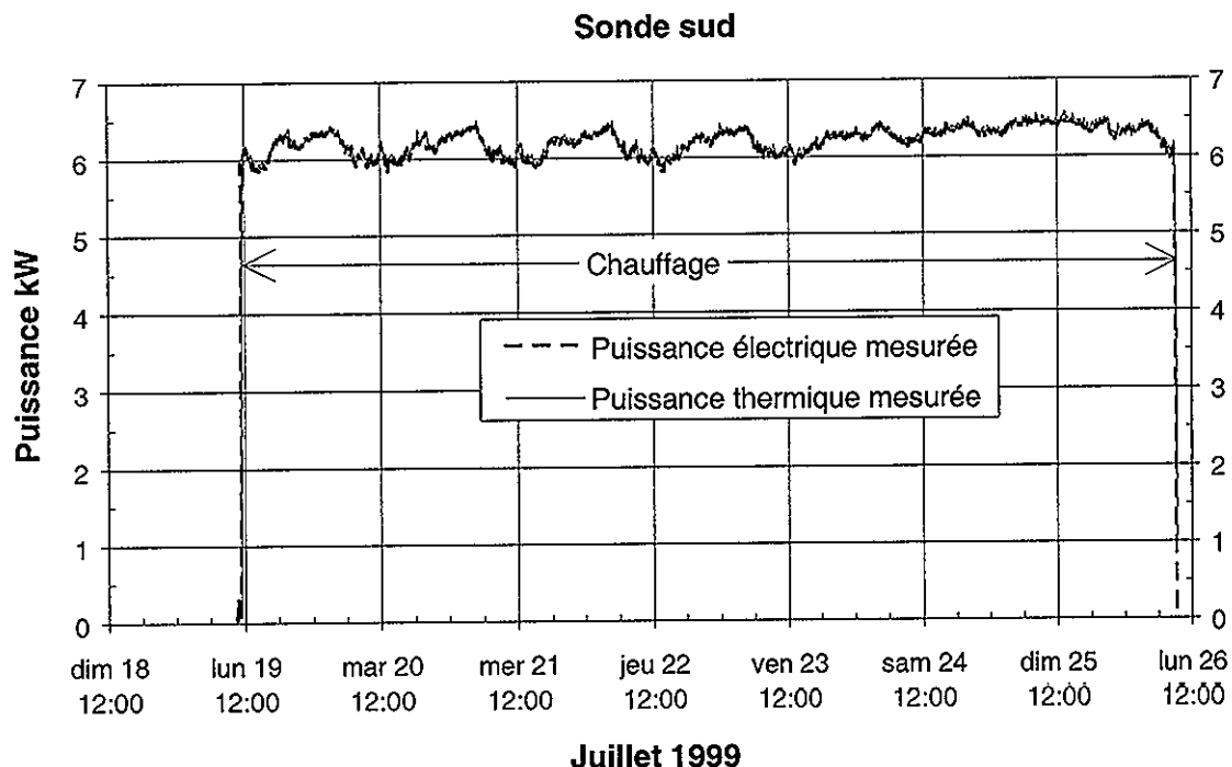
Fig. 2.8 Evolution des puissances thermique et électrique mesurées lors du test de la sonde sud.
