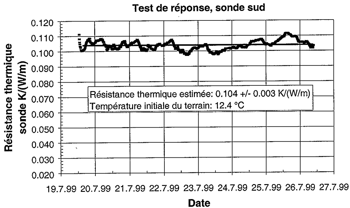
Fig. 2.10 Estimation de la résistance thermique effective de la sonde géothermique sud.
