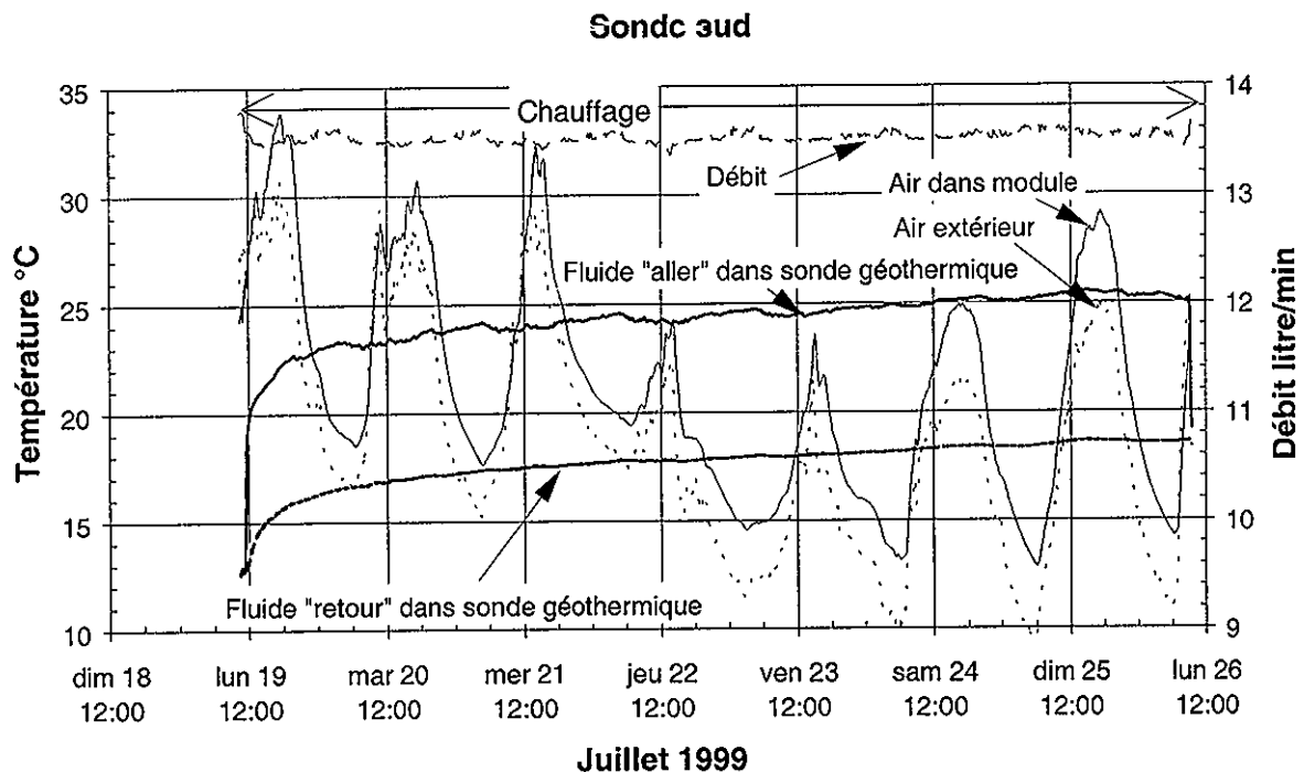
Fig. 2.7 Evolution des températures mesurées de l'eau circulant dans la sonde sud (aller et retour), de l'air dans la boîte contenant le module de chauffage, de l'air extérieur et du débit mesuré.
