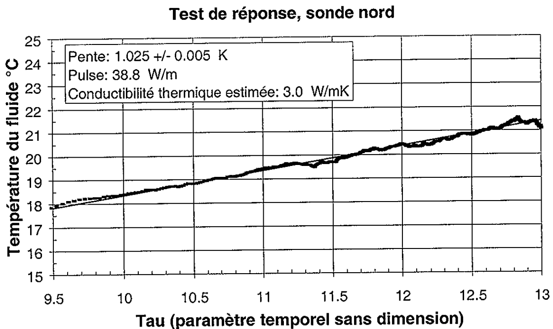
Fig. 2.5 Estimation de la conductibilité thermique moyenne du terrain avec les mesures de la sonde nord.
