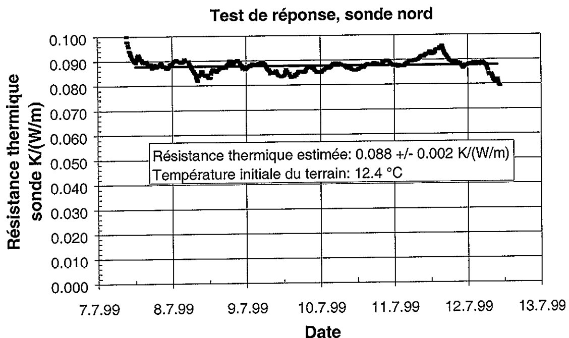
Fig. 2.6 Estimation de la résistance thermique effective de la sonde géothermique nord.
