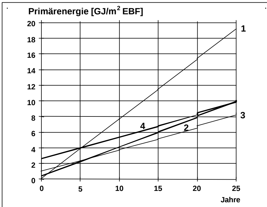
Figur 17: Aufsummierter Primärenergiebedarf für Heizung, Warmwasser, Haushaltstrom und graue Energie für verschiedene Erneuerungsvarianten für ein 24-Familienhaus aus den fünfziger Jahren. Dargestellt sind auch die periodischen Unterhaltsarbeiten mit ihrem Grauenergieeinsatz (Treppenstufen).
