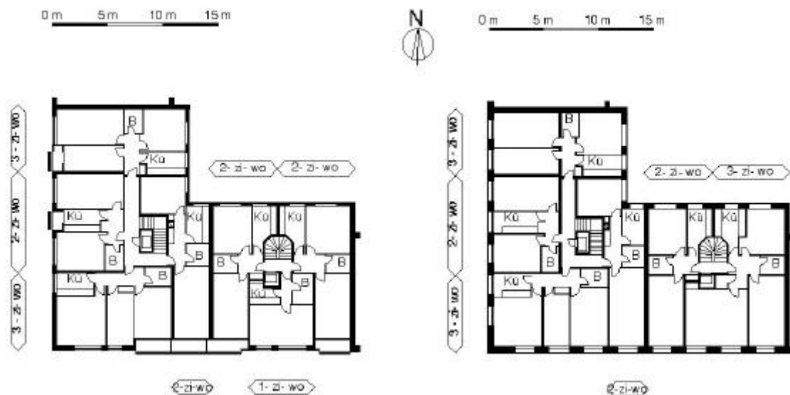
Grundriss Normalgeschoss vor und nach dem Eingriff.
