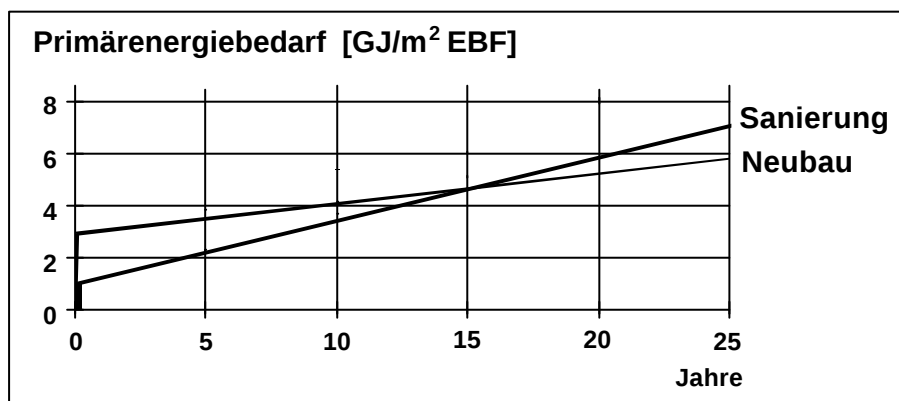
Figur 16: MINERGIE-Sanierung und MINERGIE-Ersatzneubau im Vergleich. Aufsummierter Primärenergieverbrauch für die Sanierung bzw. für Abbruch und Erstellung (graue Energie) sowie für die Beheizung der beiden Erneuerungsvarianten.
