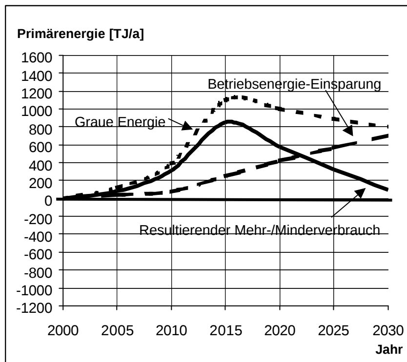
Figur 20: Resultierender Mehr- bzw. Minderverbrauch bei erhöhter Ersatzneubautätigkeit mit einem über den Betrachtungszeitraum konstanten durchschnittlichen Heizenergiebedarf der Neubauten von 220 \text{ MJ}/(\text{m}^2\text{a}) .
