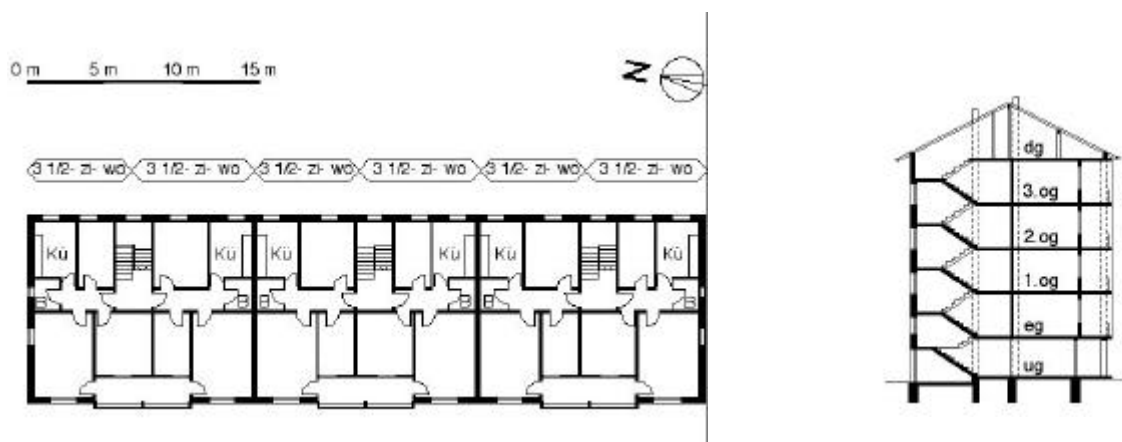
Grundriss Normalgeschoss und Querschnitt.
