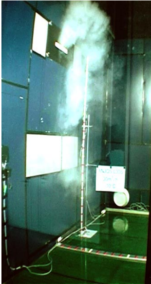
Figur 4-12: F-SH-O, Fussbodenheizung, Zulufttemperatur 2 °C
