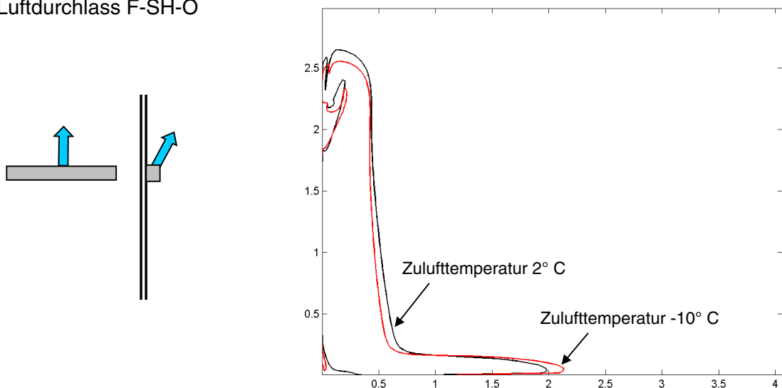
Figur 4-17: Vergleich der 20%-Isolinie für das Zugluftisiko in der Symmetrieachse bei einer Zulufttemperatur von 2°C (schwarz) gegenüber einer Zulufttemperatur von -10 °C (rot bzw. grau) mit FBH (CFD-Rechnung)
