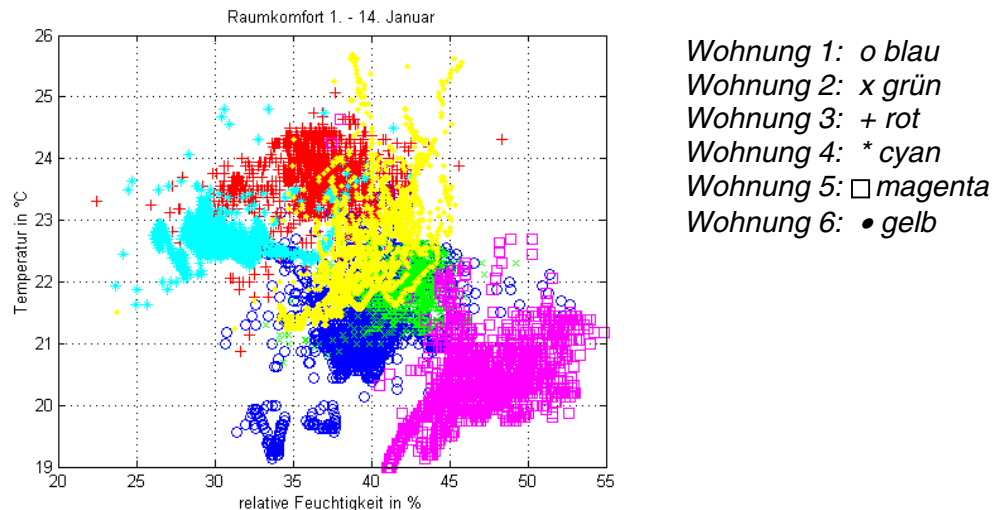
Figur 5-4: Darstellung Feuchte/Temperatur im Referenzpunkt jeder Wohnung (Januar)
