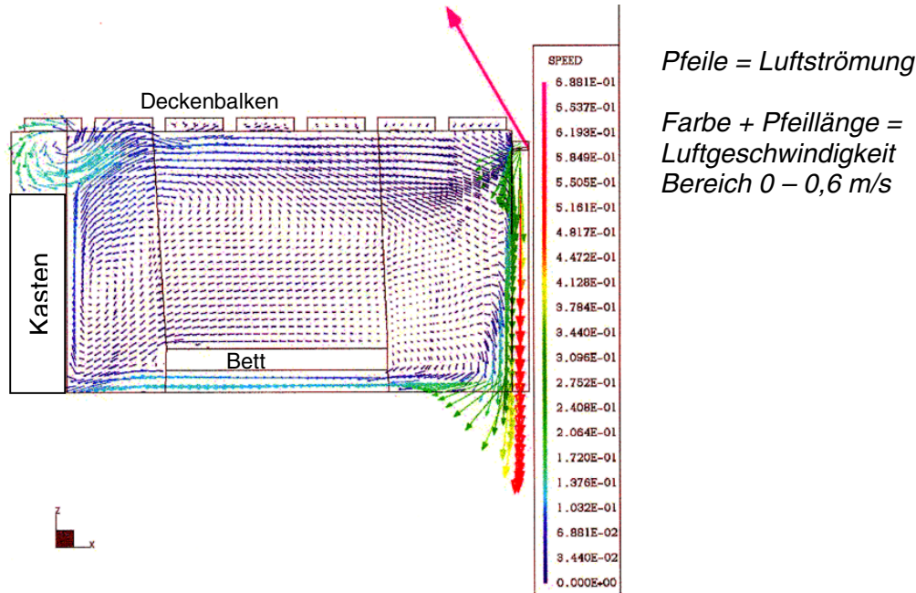
Figur 5-3: Strömungsdarstellung in Mittelebene des Raumes für Aussentemperatur von -8\text{ }^{\circ}\text{C} und realistisch modellierte Innenoberflächentemperaturen, z.B. Glas innen 16,5\text{ }^{\circ}\text{C} ; Lufteintritt durch ALD oberhalb Fenster schräg nach oben (Pfeil) [Fluck, 2000].
