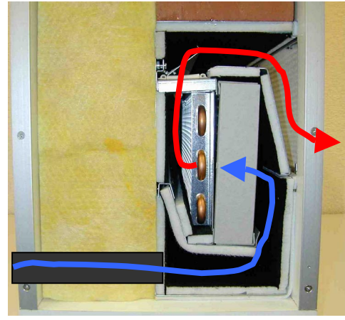
Figur 6-4: Schnitt durch die Lüftungsboxe mit Heizregister, mit skizzierten Luftpfad
