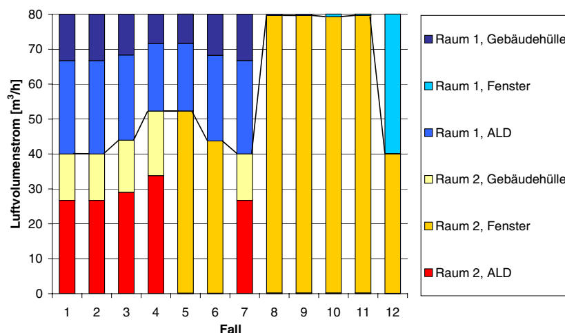
Figur 3-2: Luftvolumenströme für die untersuchten Fälle 1 bis 12. Dabei wurde nach der Herkunft der Zuluft (Gebäudeleckage, Fenster oder ALD) unterschieden.
