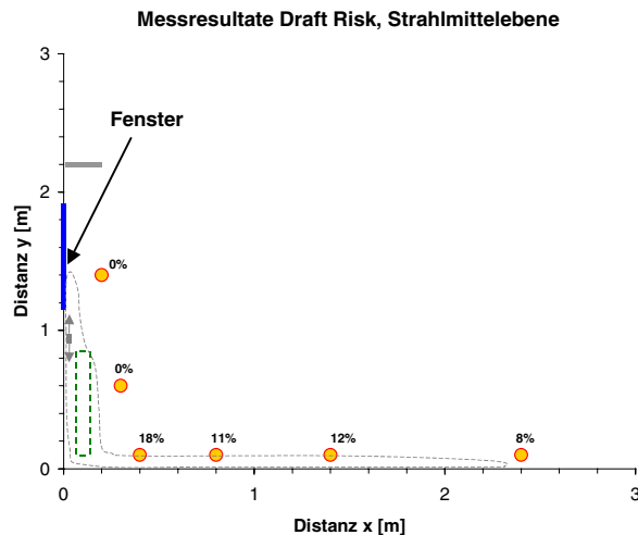
Figur 4-9: Die Eindringtiefe der Diskomfortzone wird bei der Anordnung „unten“ etwas kleiner, jedoch ist das Zugluftrisiko entlang dem Boden etwas grösser, Wärmequelle: FBH, Heizkörper ausgeschaltet.
