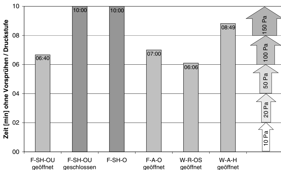
Figur 4-19: Schlagregendichtheit der untersuchten Aussenluftdurchlässe, Zeit (ohne Vorsprühen) bis Wassereintritt, und die entsprechenden Druckstufen
