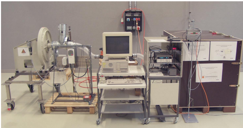
Figur 4-1: Versuchsaufbau für die Untersuchung der strömungstechnischen Eigenschaften
