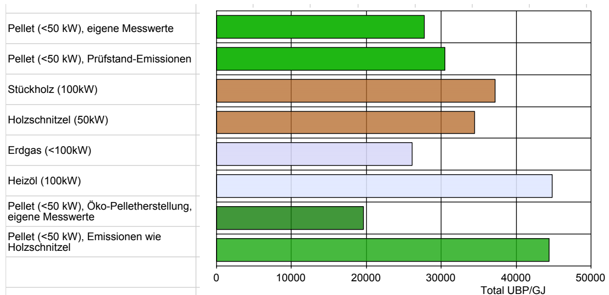
Abbildung 10.1: Total der UBP für Öl-, Gas-, Holz- und Holzpellettheizungen. Bei den Pellets wurde einmal mit den eigenen Messwerten und einmal mit den Prüfstands-Messungen gerechnet. Zur Beurteilung des ökologischen Verbesserungspotentials von Pellets wurden zusätzlich die UBP bei Verwendung eines holzbefeuerten Direktrockners mit Gewebefilter und Abwärmenutzung dargestellt (Öko-Pelletherstellung). Weiter ist der theoretische Fall, dass bei der Pelletverbrennung gleichviel Schadstoffemissionen entstehen wie bei der Holzschnitzelverbrennung angegeben.
