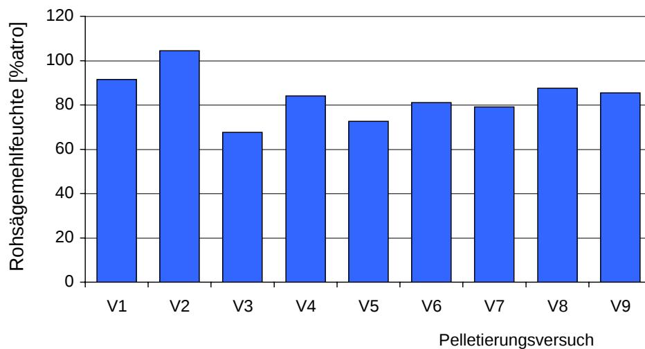
Abbildung 7.1: Feuchtegehalte des Rohsägemehls nach Anlieferung
