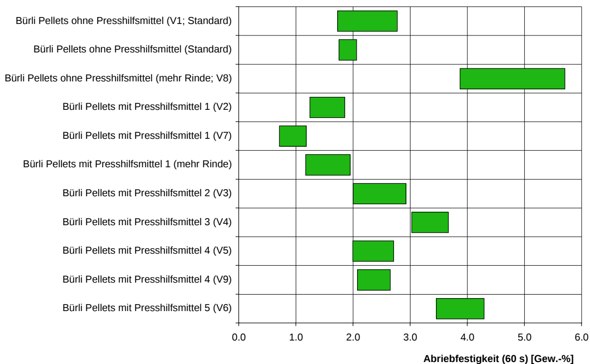
Abbildung 7.8: Vergleich des Abriebverhaltens beim Zusatz von Presshilfsmitteln
