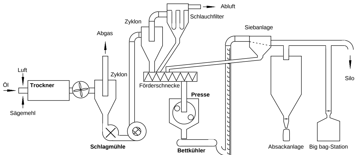
Abbildung 6.1: Verfahrensfließbild der untersuchten Holzpelletieranlage
