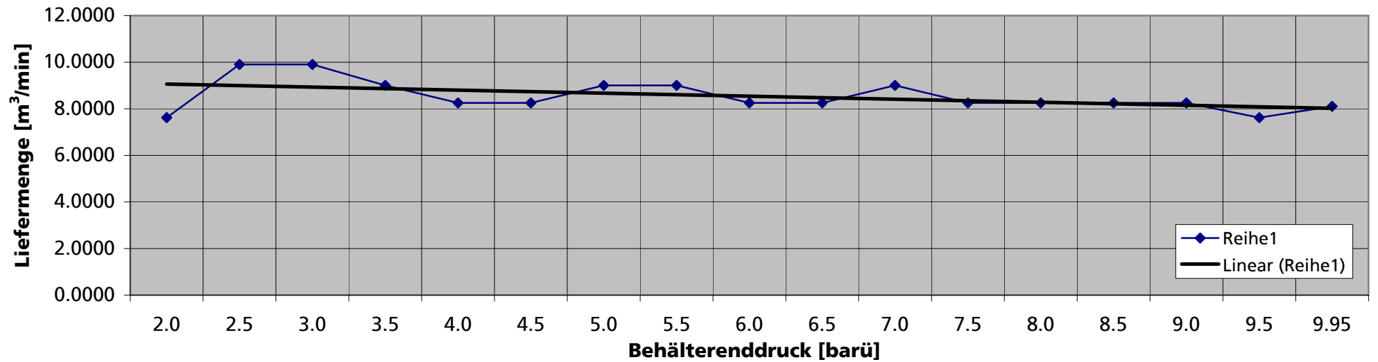
Liefermenge Kompressor 1
