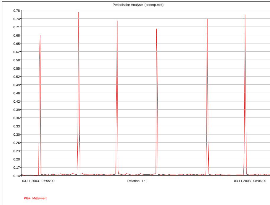
Abbildung 3.17: Leistungsfaktor (als Mittelwert) der beiden Fräsmotoren während eines Produktionszyklus. Die beiden Motoren wurden gemeinsam gemessen. Leistungsfaktor bei Leerlauf ca. 0.14. Bei Last während ca. 3-4 Sekunden ca. 0.6 bis 0.7 Last nur während ca. 3-4 Sekunden.
