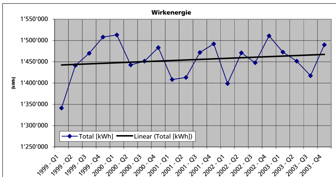
Abbildung 3.20: Wirkenergieverbrauch pro Quartal für die Jahre 1999 bis 2003
