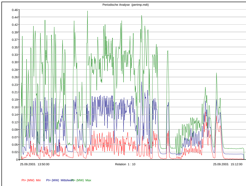
Abbildung 3.12: Minimum, Maximum und Mittelwert der Wirkleistung der Aussenhackanlage am 25.09.2003 von 13:50 bis 15:12 Uhr. Die Minimum-, Maximum- und Mittelwerte sind die Werte, welche in der am Messgerät eingestellten Integrationsperiode erfasst wurden. In dieser Aufzeichnung ist als Integrationszeit 1 Sekunde eingestellt.
