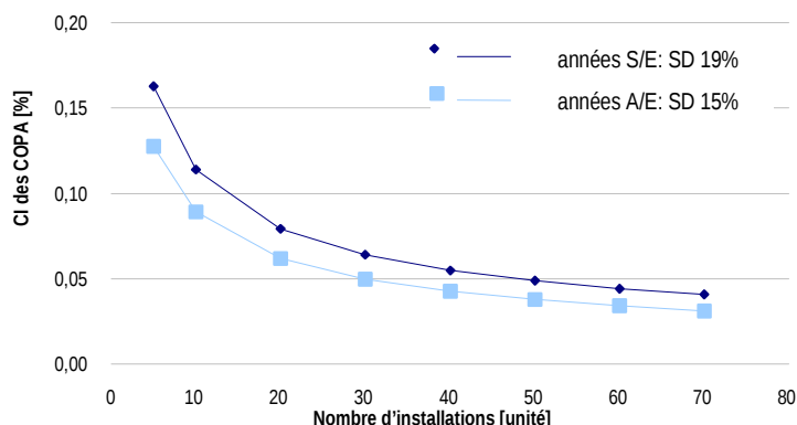
Taille des échantillons versus intervalle de confiance COPA
