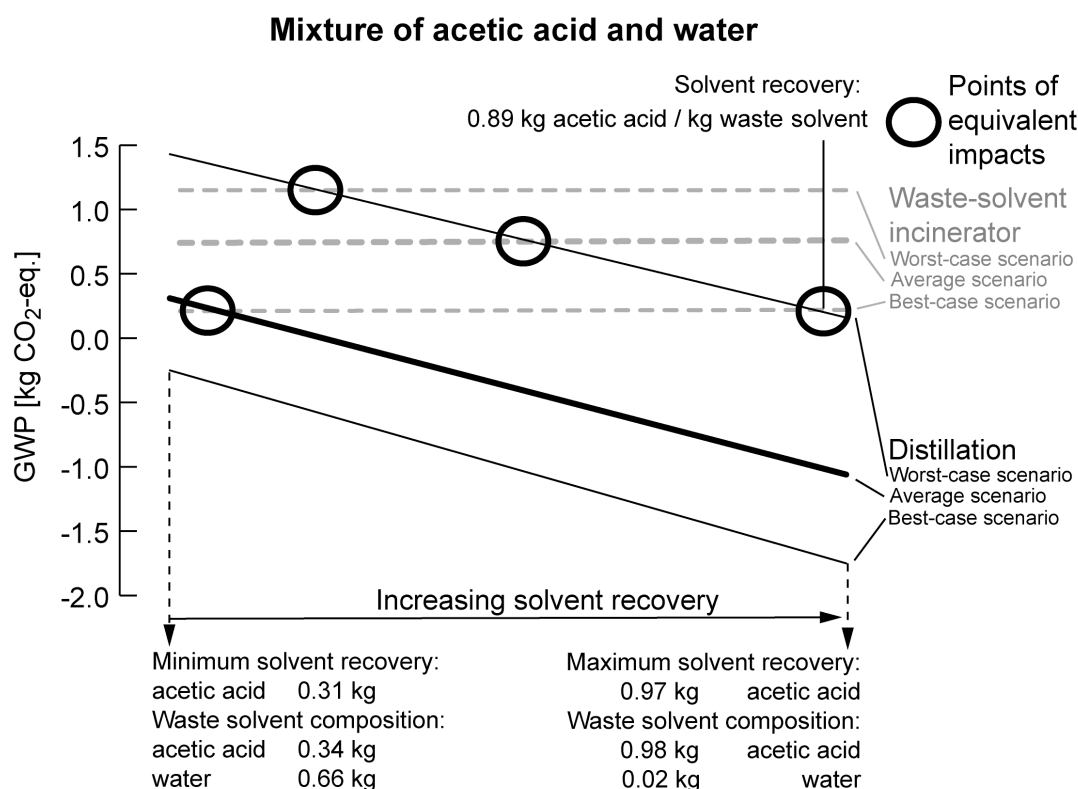
Abbildung 2: Bestimmung allgemeiner Daumenregeln für spezifische ALM. Das Beispiel von Essigsäure und Wasser zeigt, dass ab einer Lösungsmittelrückgewinnung von 0.89 kg pro kg ALM die Destillation grundsätzlich die aus Umweltsicht zu bevorzugende Technologie ist.
