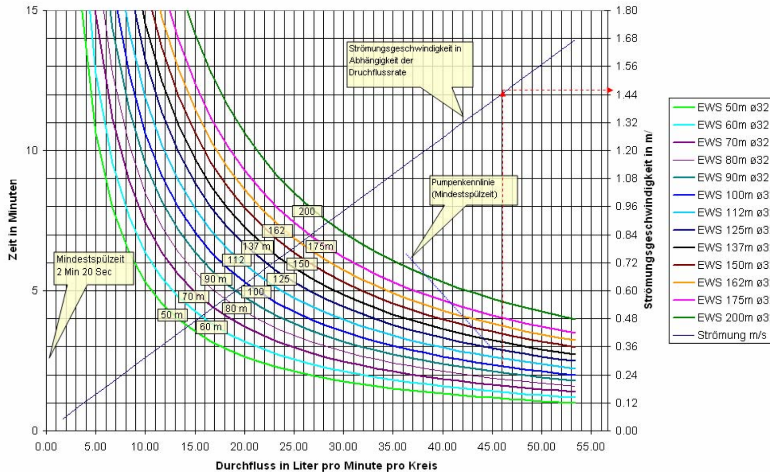
Mindestspüldauer für einen Umgang bei ø32mm EWS pro Kreis
