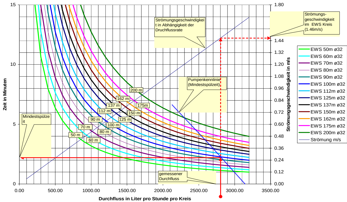
Figur 15: Mindestspüldauer für \varnothing 32\text{mm} Erdwärmesonden verschiedener Tiefe (pro Kreis). Ist bereits eine Y-Verbindung an der Sonde angeschlossen, muss die Spüldauer mindestens verdoppelt werden.
