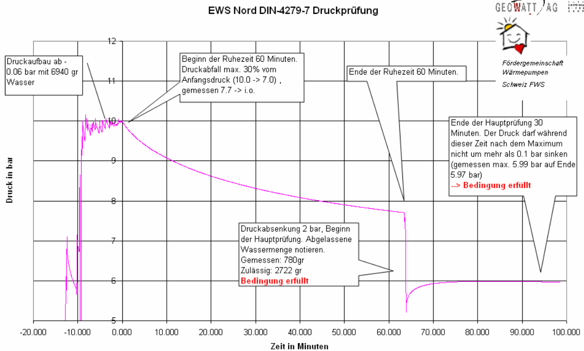
Figur 20: Druckprüfung in Anlehnung an die DIN V 4279-7 zeigt für die getestete Erdwärmesonde keine Leckage.
