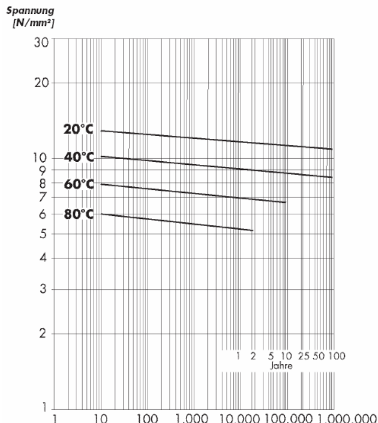
Zeitstand-Innendruck-Diagramm für Polyethylen PE 100
