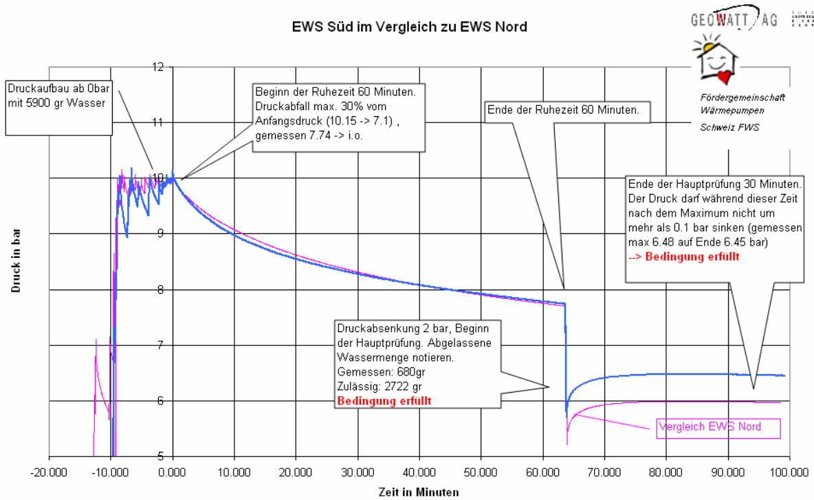
Figur 22: Vergleich der beiden EWS (Nord Magenta leak, Süd blau dicht)
