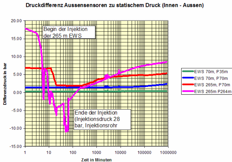
Figur 3: Druckverhältnisse in einer 70 m und einer 265 m tiefen Erdwärmesonde jeweils am Sondenfuss und auf 35 m respektive 70 m Sondentiefe (Rohner et al., 2000).
