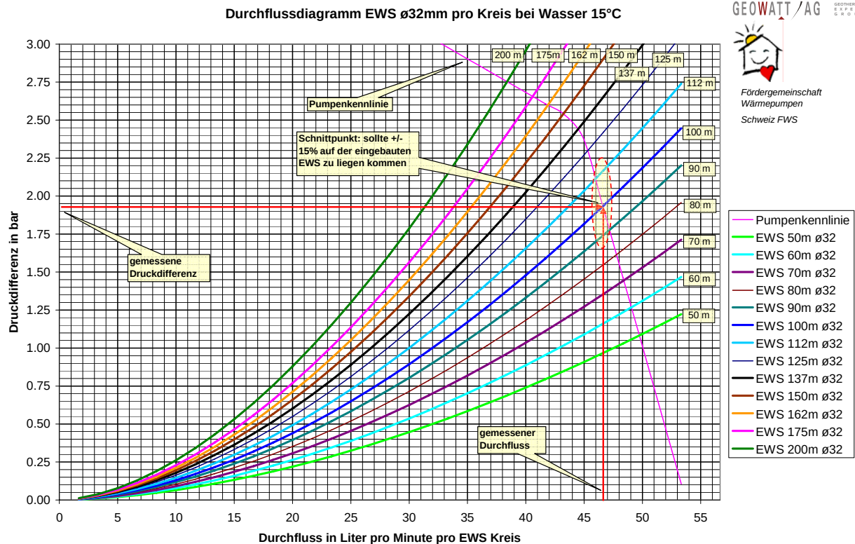
Figur 17: Durchflussdiagramm für eine Erdwärmesonde mit 32 mm Rohrdurchmesser
