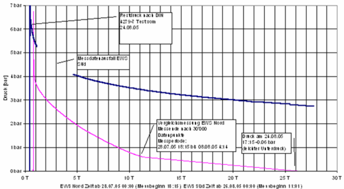
Figur 22: Vergleich der beiden EWS (Nord Magenta leak, Süd blau dicht)
