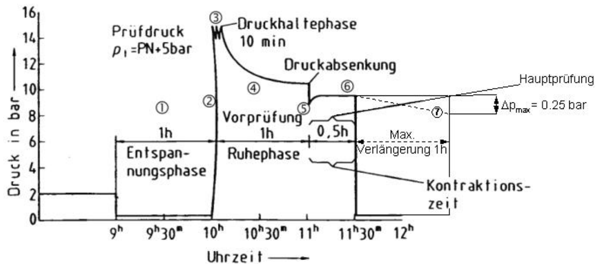
Figur 2: Druckverlauf während der Prüfung. Die Bildlegende ist der nachfolgenden Tabelle zu entnehmen.
