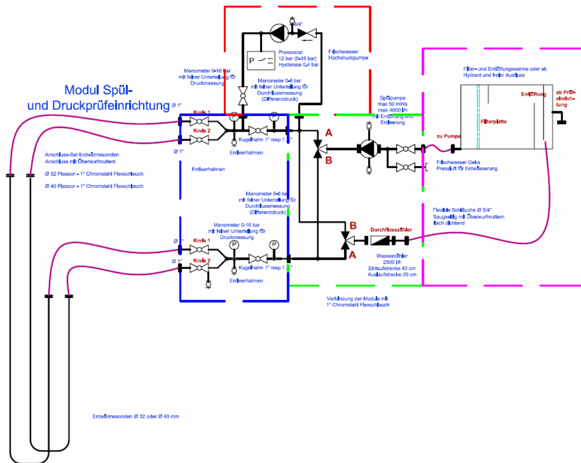
Figur 10: Modulare Druck- und Durchflussprüfeinrichtung
