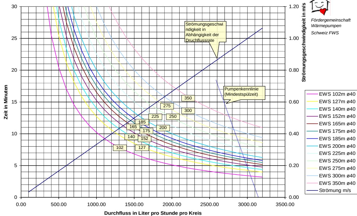
Figur 16: Mindestspüldauer für \varnothing 40\text{mm} Erdwärmesonden verschiedener Tiefe (pro Kreis). Ist bereits eine Y-Verbindung an der Sonde angeschlossen, muss die Spüldauer mindestens verdoppelt werden.
