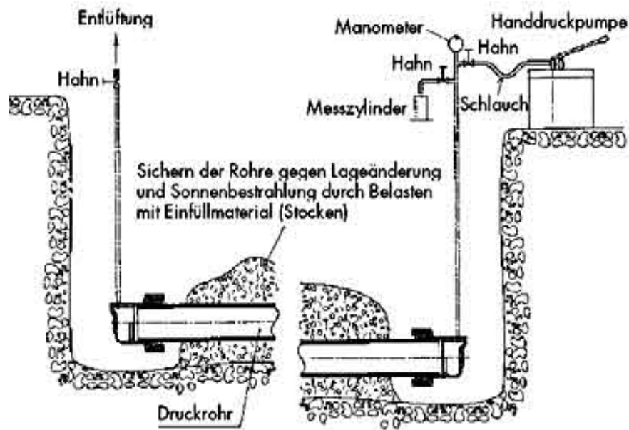
Figur 1: Aufbau Prüfeinrichtung für horizontale Rohre.
