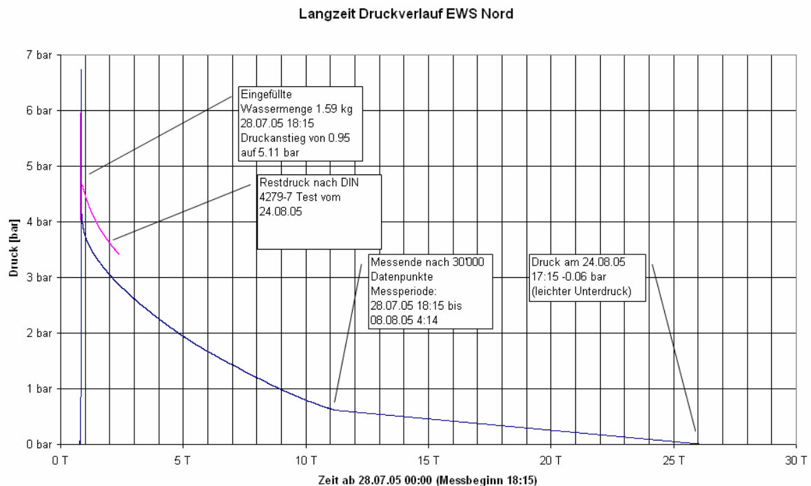
Figur 21: Langzeitdruckmessung in der Erdwärmesonde zeigt deutlich eine Leckage.
