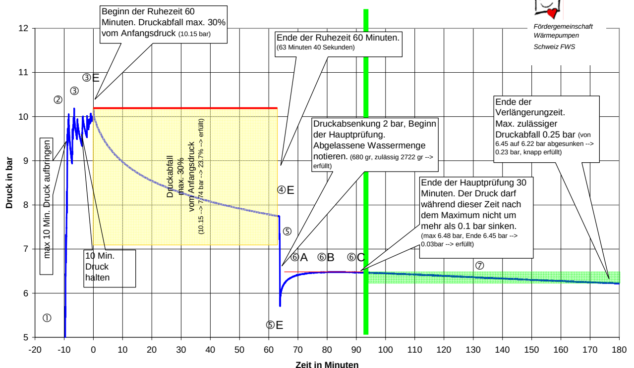
Figur 5: Druckprüfung in Anlehnung an DIN V 4279-7. Die dargestellte Druckkurve wurde mit dem später in Kapitel 3.1 vorgestellten Prüfgerät während dem Test einer dichten, 290 m Erdwärmesonde aufgenommen. Die effektiv Werte sind eingetragen.
