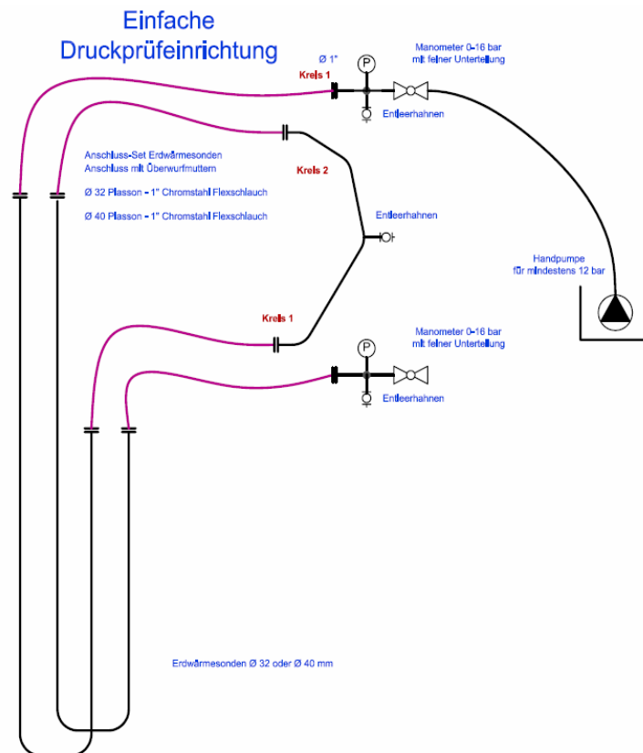
Figur 6: Schema einfache Druckprüfeinrichtung
