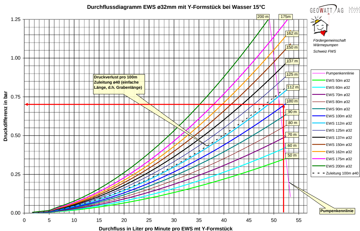
Figur 18: Durchflussdiagramm für eine Erdwärmesonde mit 32 mm Rohrdurchmesser und angeschlossenem Y-Formstück.
