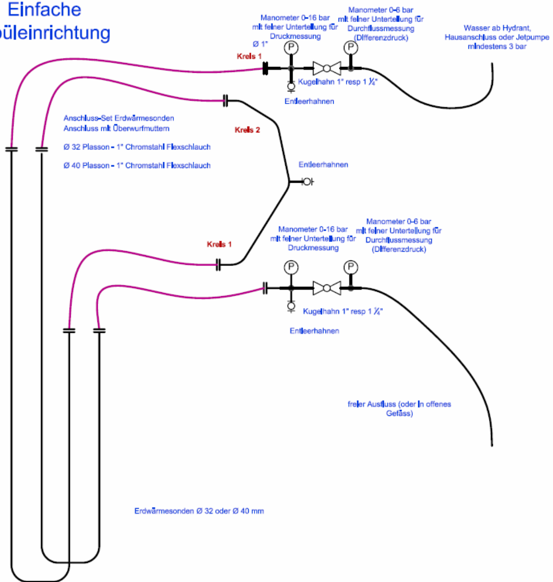
Figur 9: Schema einfache Druckprüfeinrichtung mit Spüleinrichtung.
