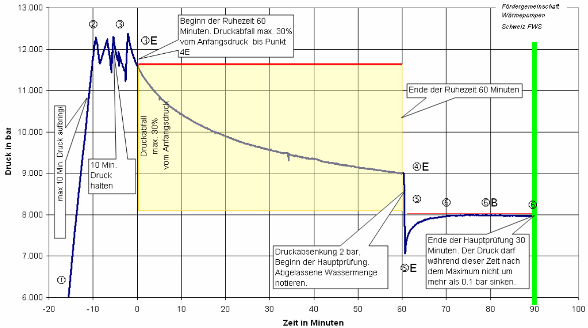
Figur 19: Beispiel für die Auswertung einer Druckprüfung
