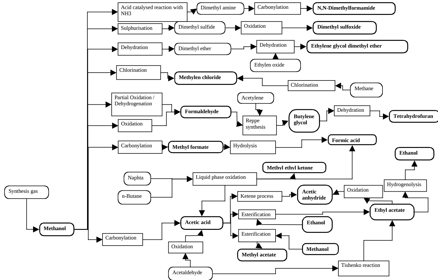
Abbildung 2: Methanol-Route
