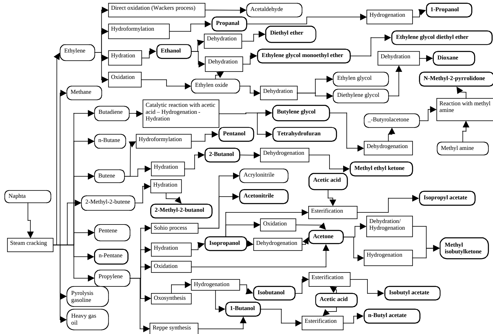
Abbildung 3: Dampfcracker-Route
