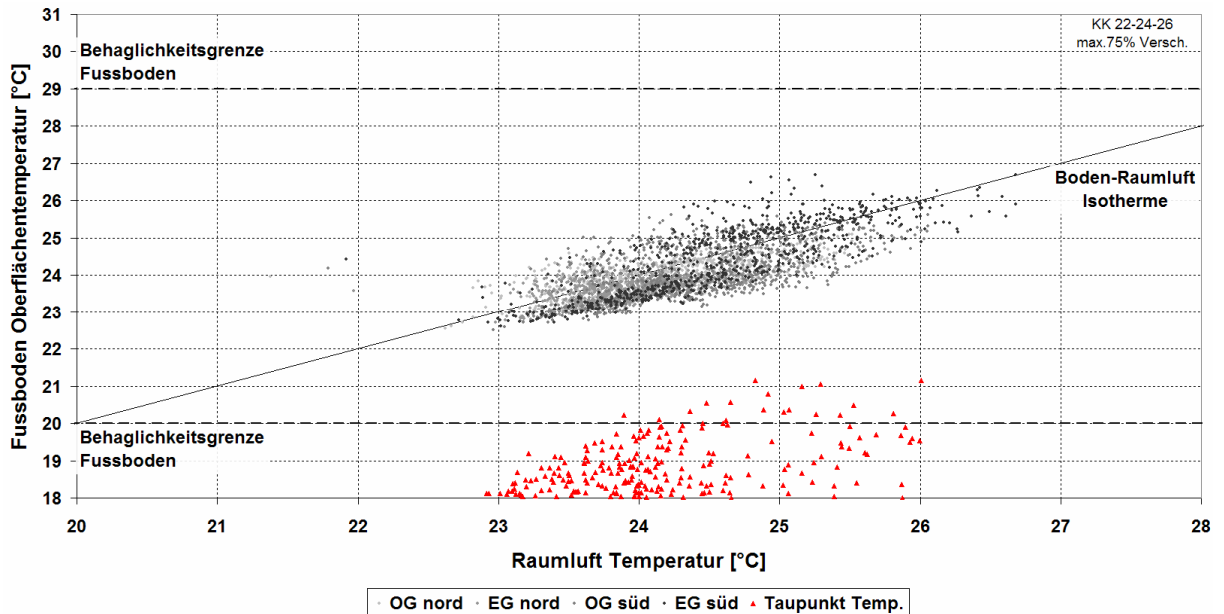
Abb. 3.13: Darstellung der Fussboden – Oberflächentemperaturen und Taupunkttemperaturen gegenüber der Raumlufttemperatur für die Variante H+K 1 mit Kühllkurve KK 22-24-26
