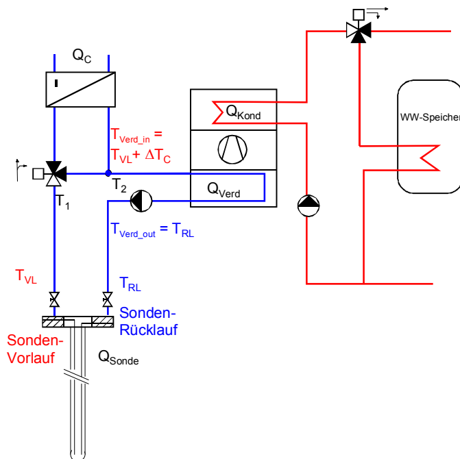
Abb. 3.4: Warmwasserproduktion im parallelen Kühlbetrieb, Erdwärmesonde zwischen Wärmetauscher und Verdampfer geschaltet: Empfohlene hydraulische Schaltung (besserer COP)
