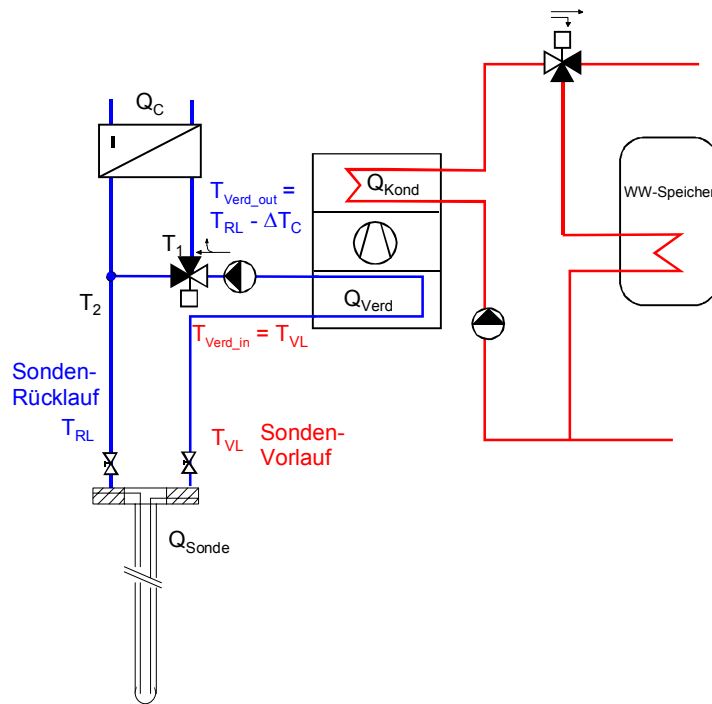
Abb. 3.3: Warmwasserproduktion im parallelen Kühlbetrieb, Wärmetauscher direkt nach Verdampfer: Hydraulische Schaltung nicht empfohlen (Frostgefahr Wärmetauscher, schlechterer COP)
