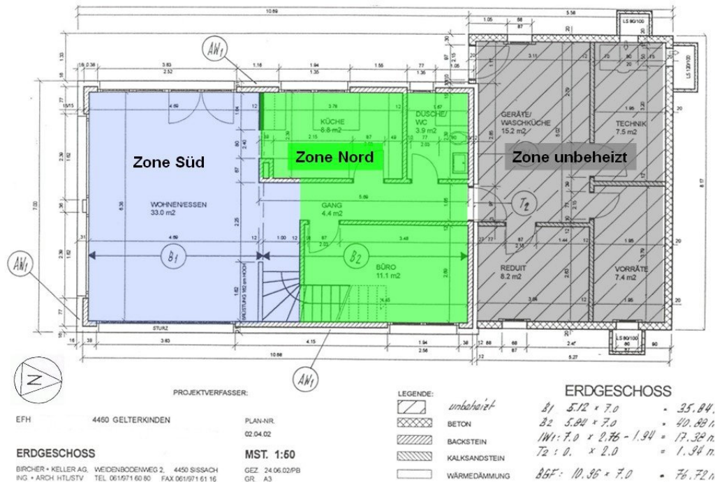
Abb. 2.9: Zonierung Erdgeschoss
