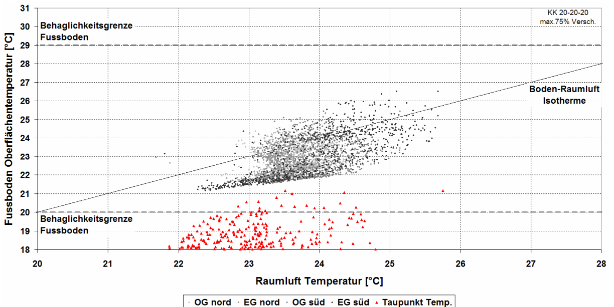
Abb. 3.14: Darstellung der Fussboden – Oberflächentemperaturen und Taupunkttemperaturen gegenüber der Raumlufttemperatur für die Variante H+K 7 mit Kühllkurve KK 20-20-20
