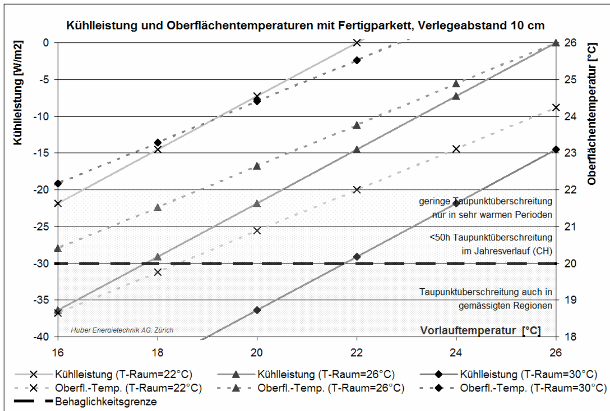
Abb. 6.17: Kühllastkurven mit Fertigparkett, bei einem Verlegeabstand Fussbodenheizungsrohre von 10cm, Fussbodenheizungsrohren von d_a=16\text{mm} / d_i=12\text{mm} und einem Durchsatz von 0.025 kg/s
