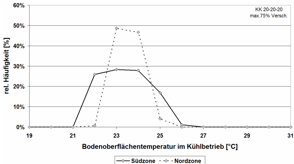
Abb. 3.7 Häufigkeitsverteilung der Fussbodenoberflächentemperaturen im Kühlfall
