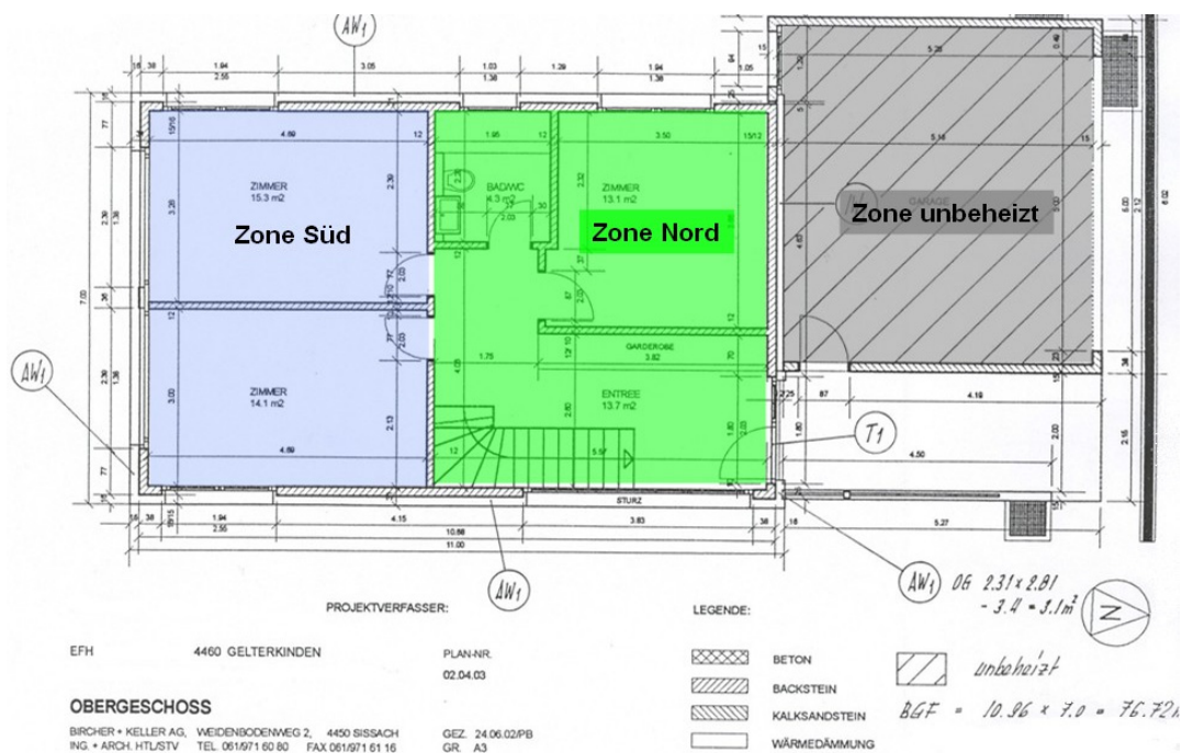
Abb. 2.10: Zonierung Obergeschoss
