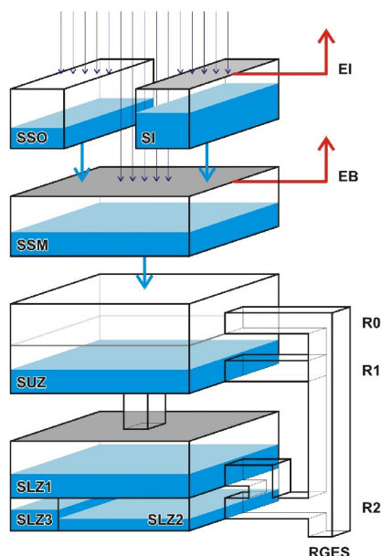
Abbildung 4: Prinzip der kaskadierenden Linearspeicher im hydrologischen Modellsystem PREVAH (aus Vivioli et al. 2007)
