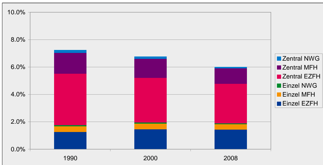
Abbildung 5: Anteil der Wohnungen mit Elektroheizungen am Gesamtbestand beheizter Wohnungen, unterteilt nach Heizungssystem und Gebäudetyp.
