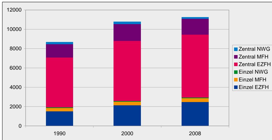
Abbildung 7: Endenergieverbrauch durch elektrische Widerstandsheizungen, nach Heizungssystem und Gebäudetyp (in TJ).
