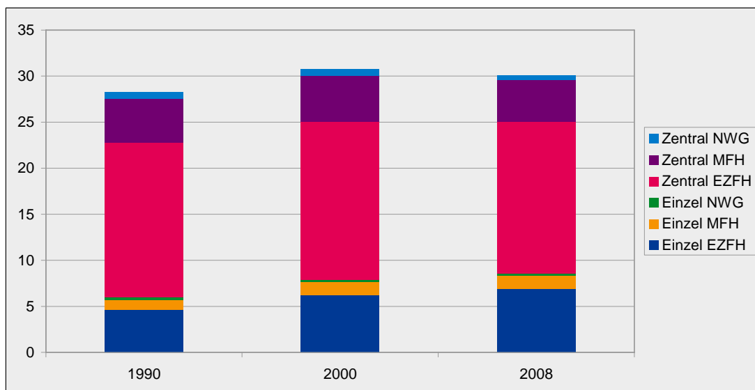
Abbildung 6: Energiebezugsfläche der mit Elektroheizungen beheizten Wohnungen, nach Heizungssystem und Gebäudetyp (in Mio.m 2 ).
