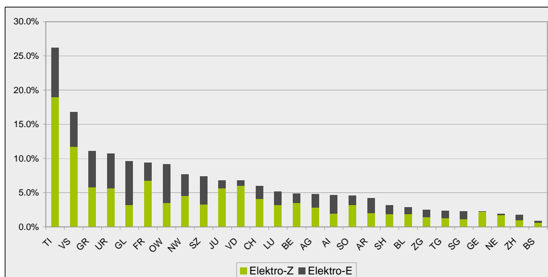
Abbildung 8: Anteil der Wohnungen mit elektrischen Widerstandsheizungen am Gesamtbestand an beheizten Wohnungen im Jahre 2008, nach Kantonen sowie getrennt nach Einzel – und Zentralheizungen.
