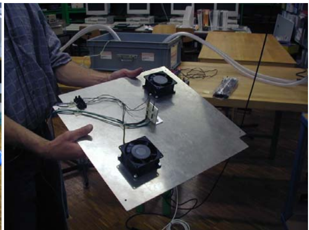
Figure 3 : échangeur industriel et fond avec ventilateurs de brassage
