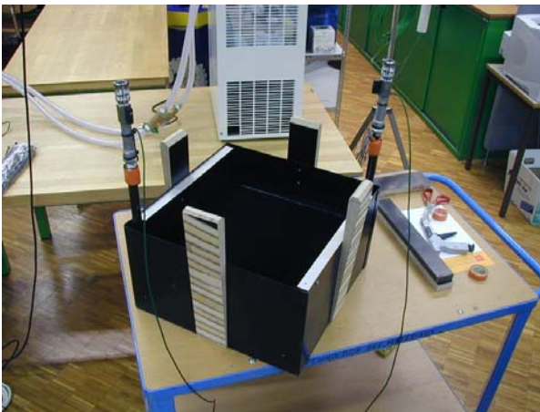
Figure 3 : échangeur industriel et fond avec ventilateurs de brassage
