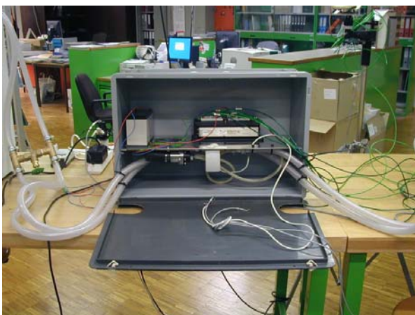
Figure 6 : caisse contenant l'acquisiteur et la régulation
