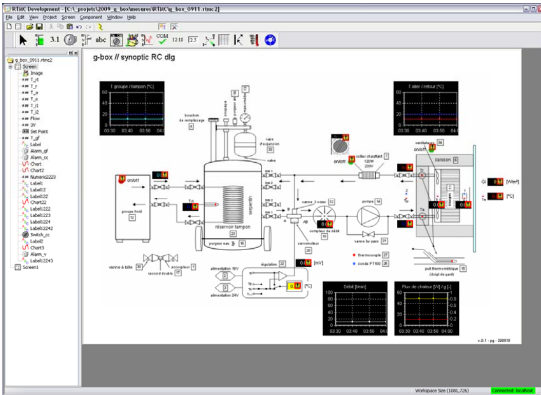
Figure 1: interface graphique d'exploitation du g-box (via Internet)
