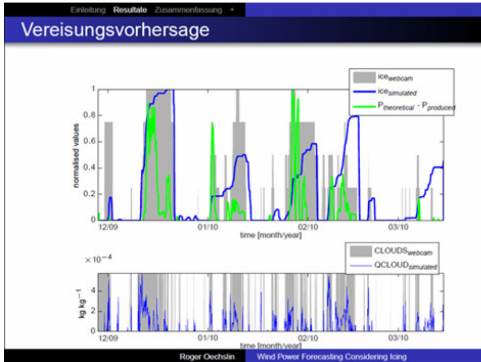
Abb. 51: Abhängigkeit des Produktionsverlusts einer Windkraftanlage (grün) in Abhängigkeit von der Eislast (blau). Grau markiert sind Bereiche mit instrumenteller Vereisung.
