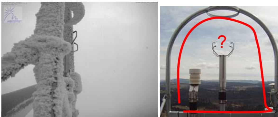
Abb. 34: Links: Eisansatz am Blitzschutz während eines starken Vereisungsereignisses. Rechts: Schematische Darstellung einer möglichen Beeinflussung der Windmessung durch starken Eisansatz am Blitzschutz.
