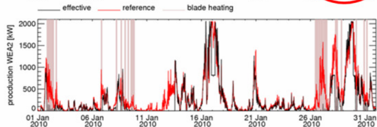
Abb. 27: Verlauf der Produktion an WEA 1 (oben) und WEA 2 (unten).
