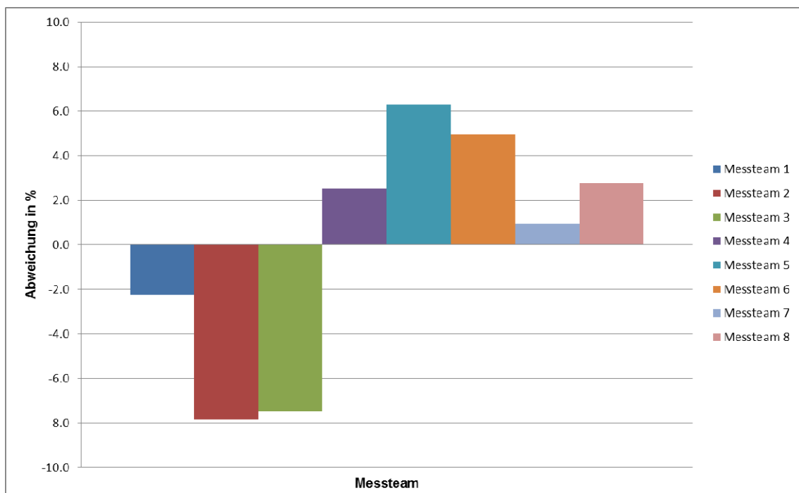
Abbildung 9: Abweichungen des Volumenstrom Unterdruck der einzelnen Messungen in % vom Mittelwert
