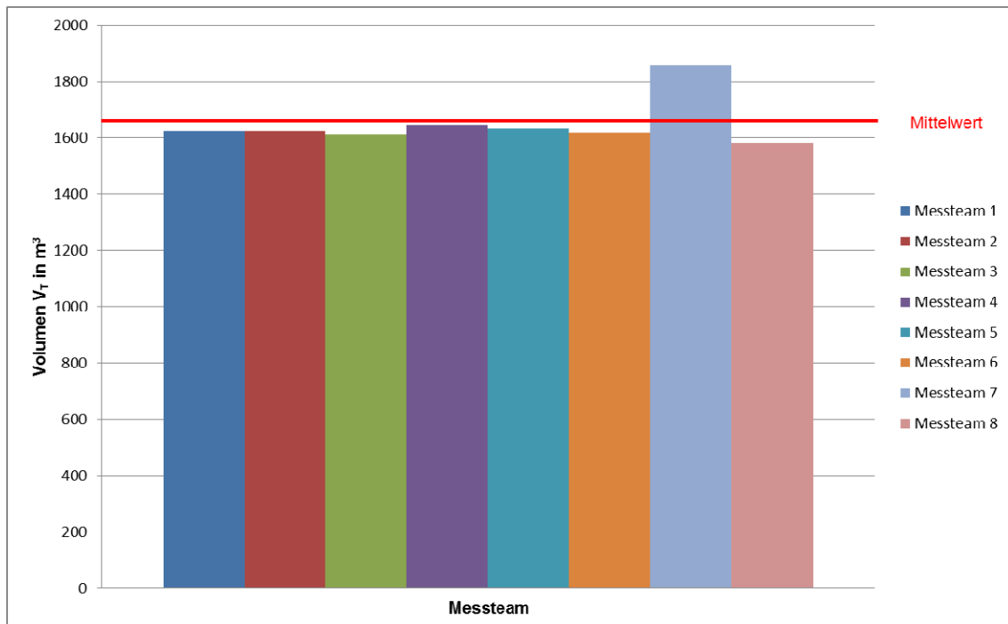
Abbildung 6: Ermittelte Volumen im \text{m}^3 der Messungen 1 bis 8; Mittelwert = 1'650 \text{m}^2
