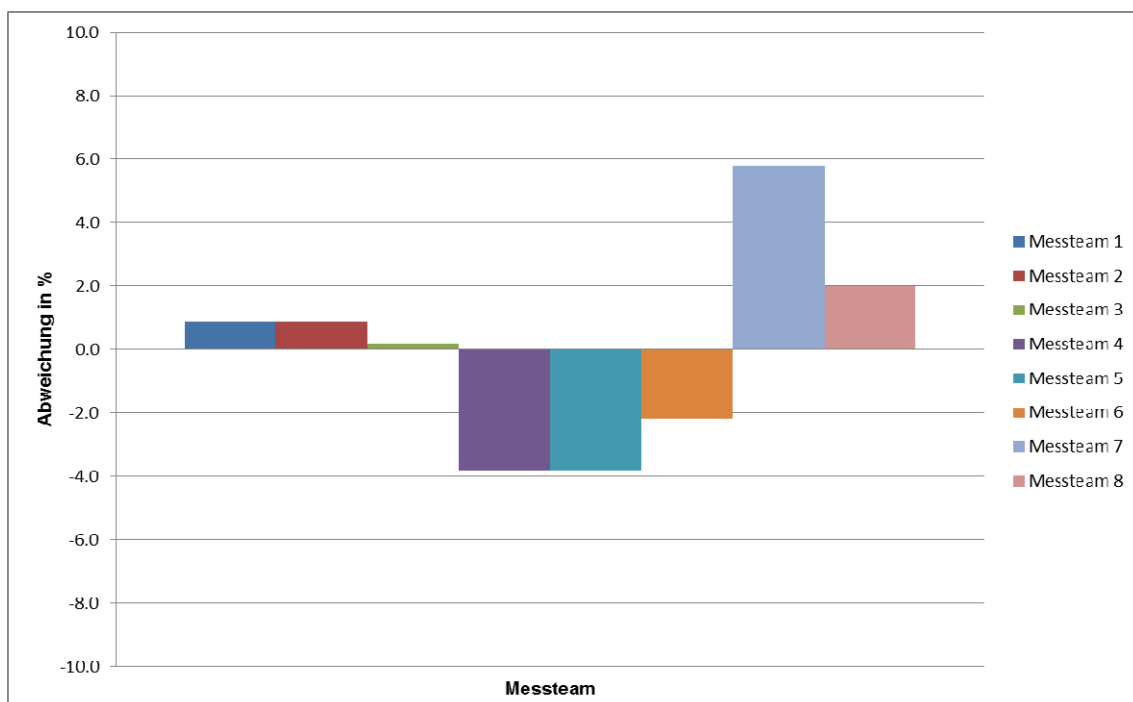
Abbildung 5: Abweichungen der Hüllflächen der einzelnen Messungen in % vom Mittelwert
