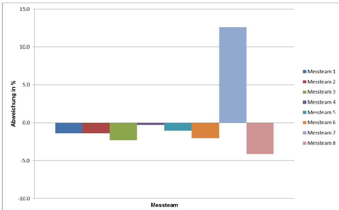
Abbildung 7: Abweichungen der Volumen der einzelnen Messungen in % vom Mittelwert
