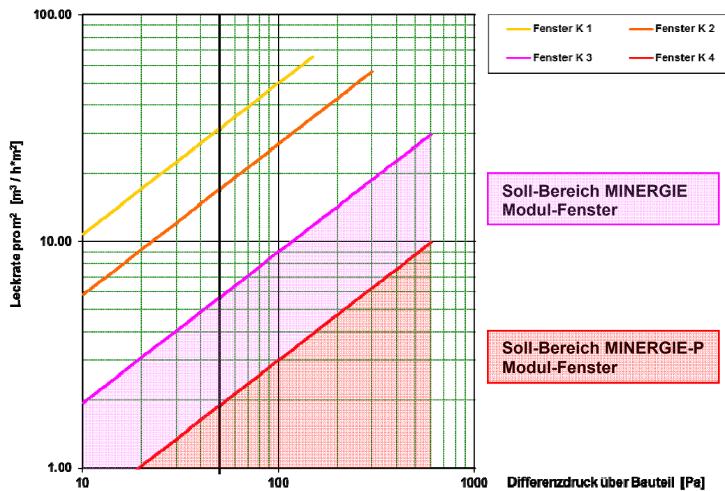
Abbildung 24: Graphische Darstellung der Anforderungen nach SN EN 12207
