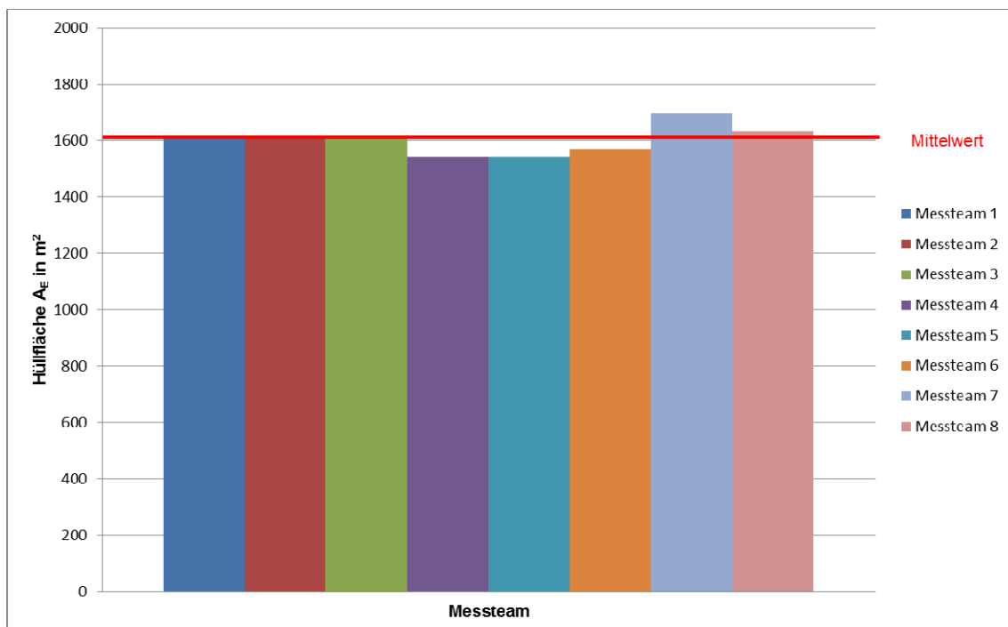
Abbildung 4: Ermittelte Hüllflächen in m 2 der Messungen 1 bis 8; Mittelwert = 1'603 m 2
