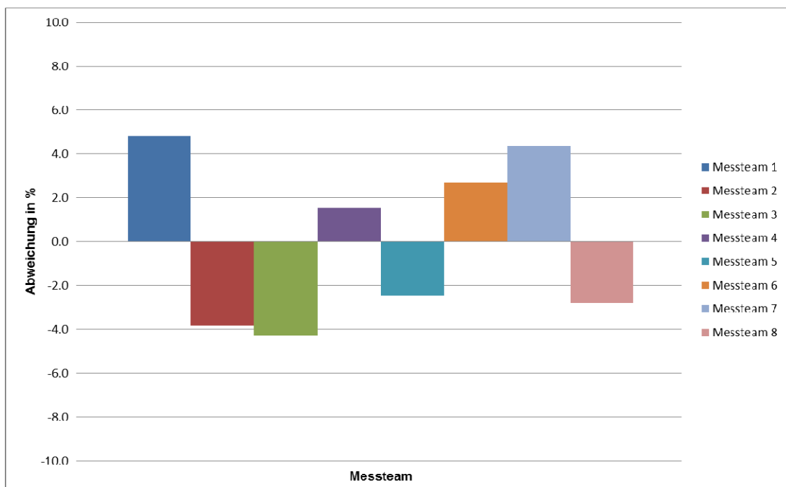
Abbildung 11: Abweichungen des Volumenstrom Überdruck der einzelnen Messungen in % vom Mittelwert
