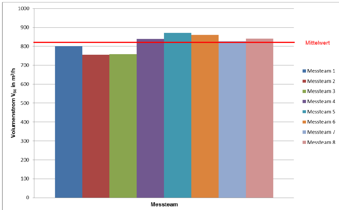
Abbildung 8: Ermittelte Volumenströme der Messungen 1 bis 8 bei Unterdruck in \text{m}^3/\text{h} ; Mittelwert = 819 \text{ m}^3/\text{h}
