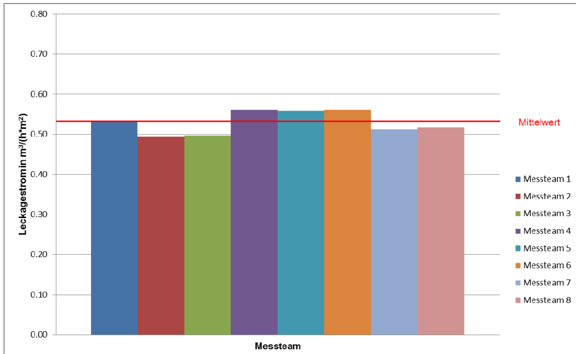
Abbildung 12: Ermittelte q_{50} -Werte der Messungen 1 bis 8 als Mittelwert aus Unter- und Überdruck in \text{m}^3/(\text{h} \cdot \text{m}^2)
