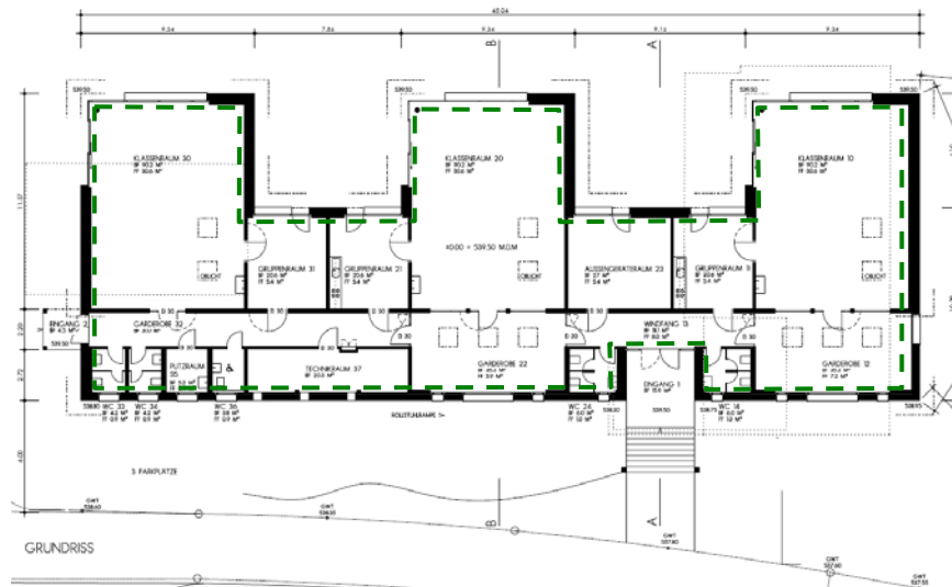
Abbildung 2: Grundriss mit eingetragener Luftdichtigkeitsebene
