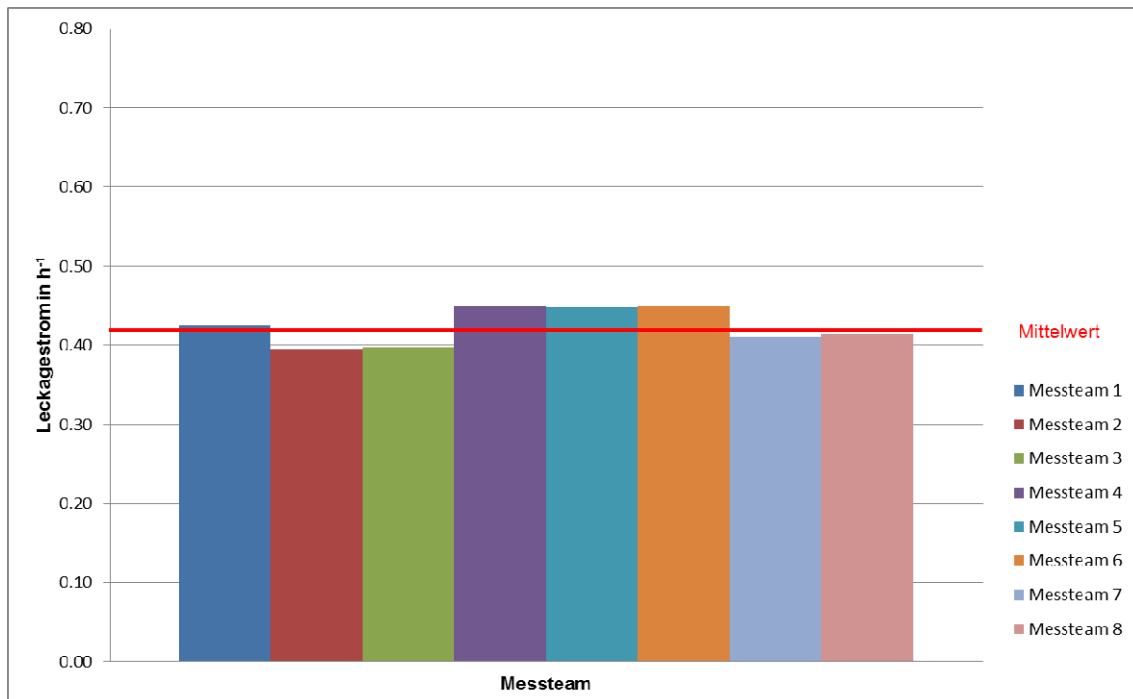
Abbildung 14: Ermittelte n_{50,st} -Werte der Messungen 1 bis 8 als Mittelwert aus Unter- und Überdruck in h^{-1}
