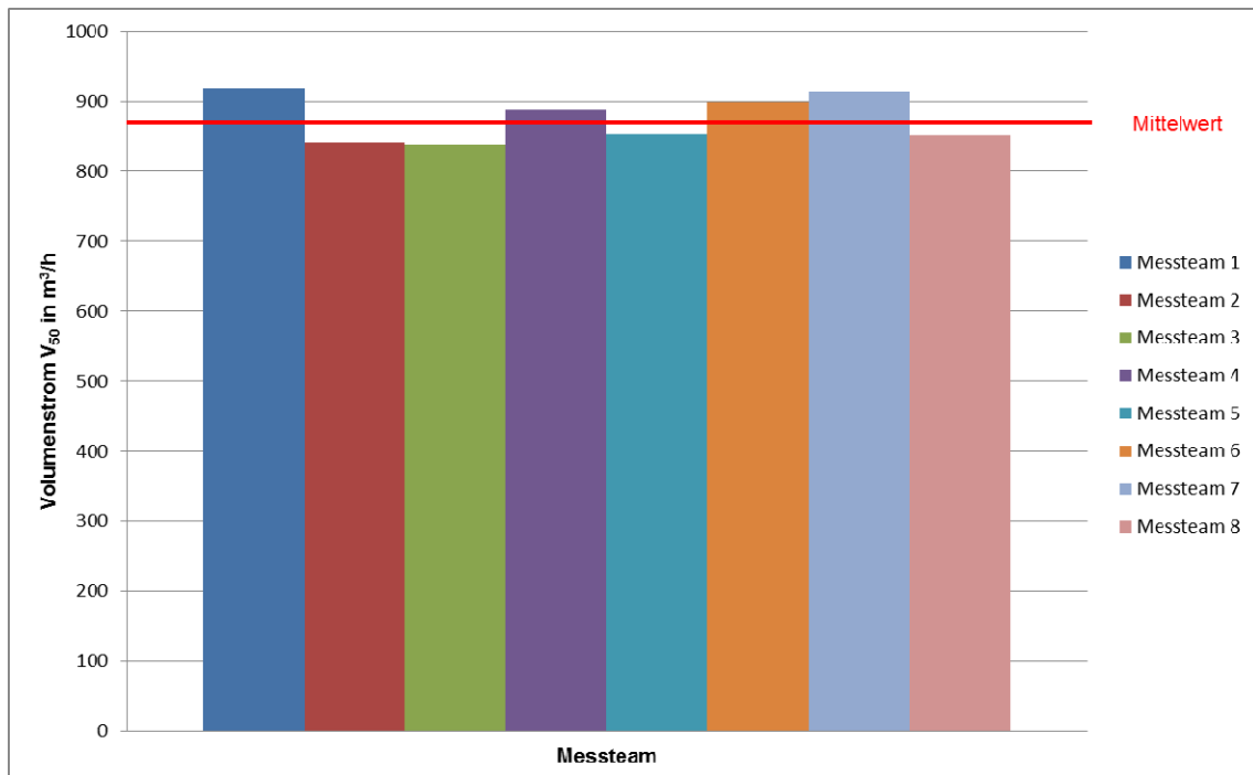
Abbildung 10: Ermittelte Volumenströme der Messungen 1 bis 8 bei Unterdruck in \text{m}^3/\text{h} ; Mittelwert = 876 \text{m}^3/\text{h}
