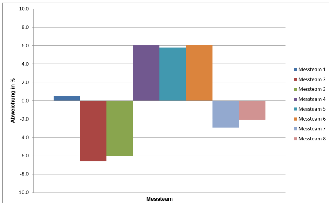
Abbildung 13: Abweichungen der Kennwerte q_{50} der einzelnen Messteams in % vom Mittelwert
