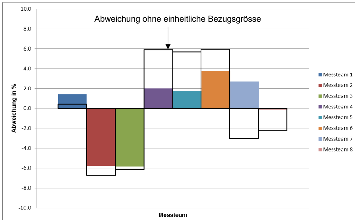
Abbildung 16: Abweichungen der Kennwerte q_{50} und n_{50, \text{st}} der einzelnen Messteams in % bezogen auf die mittlere Hüllfläche von 1603 \text{ m}^2
