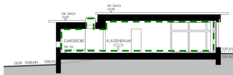
Abbildung 3: Querschnitt mit eingetragener Luftdichtigkeitsebene
