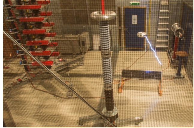
Figur 7: Hochspannungslabor an der BFH in Burgdorf (© 2014 Daniel Forster / NET Ltd.)
