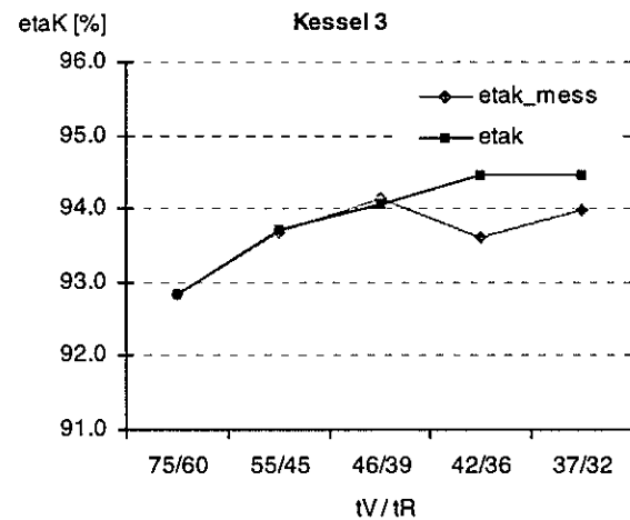
Abbildung 7.5 Vergleich Messung Rechnung: Umrechnung vom gegebenen t_V/t_R -Paar 75/60°C auf andere t_V/t_R -Paare (Vollast)
