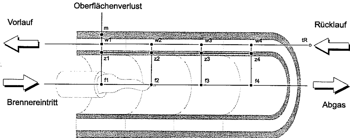
Abbildung 5.3 Rechengitter für das Heizkesselmodell.
