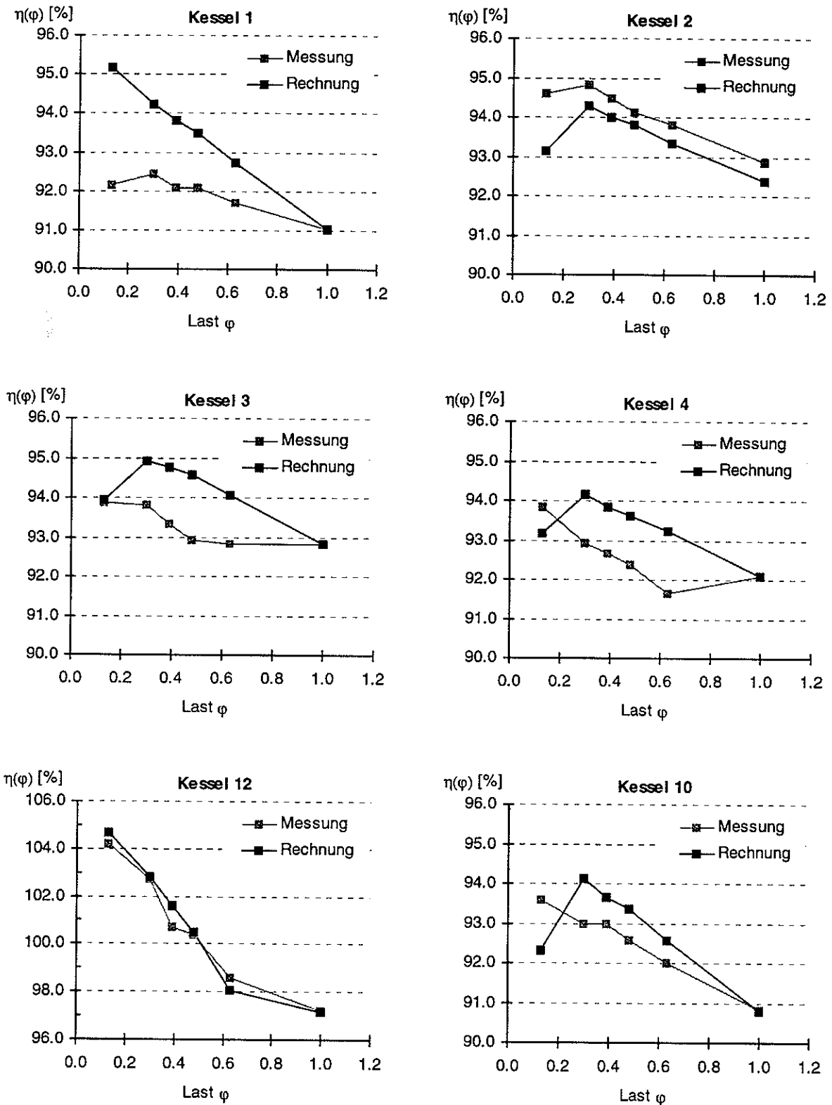
Abbildung 7.2 Vergleich Messung und Rechnung der Nutzungsgrade bei den fünf Laststufen des Normnutzungsgrades. Last = 1.0 entspricht dem Volllastwirkungsgrad.
