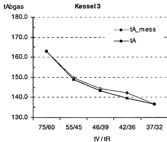
Abbildung 7.5 Vergleich Messung Rechnung: Umrechnung vom gegebenen t_V/t_R -Paar 75/60°C auf andere t_V/t_R -Paare (Vollast)
