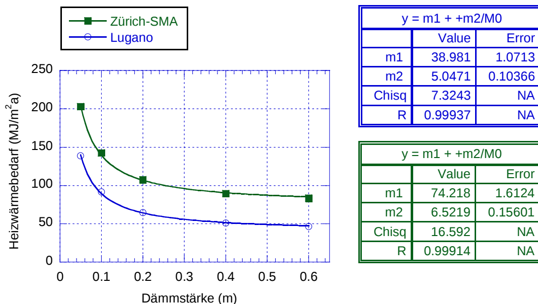
Fig. 3: Beispiele für Simulationsergebnisse (Punkte) und Fits (Linien) bei einem Mehrfamilienhaus in Zürich-SMA und Lugano
