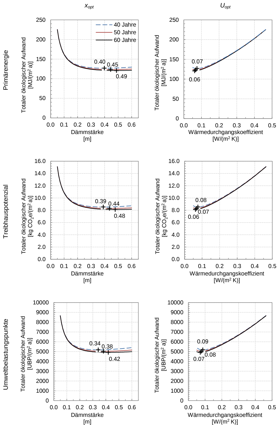
Fig. 28: Einfluss der Lebensdauer der Wärmedämmung (Referenzfall Altbau, Ölkessel)
