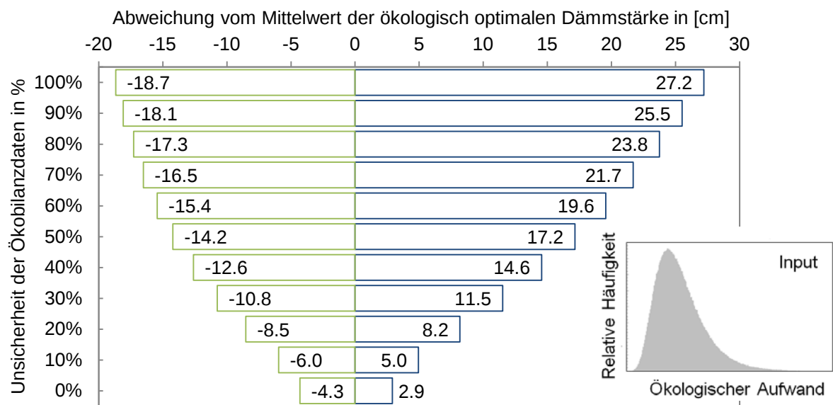
Fig. 8: Unsicherheit der ökologisch optimalen Dämmstärke (Konfidenzniveau 95%) in Abhängigkeit der Unsicherheit der Ökobilanzdaten [WvG14] (Indikator: UBP)
