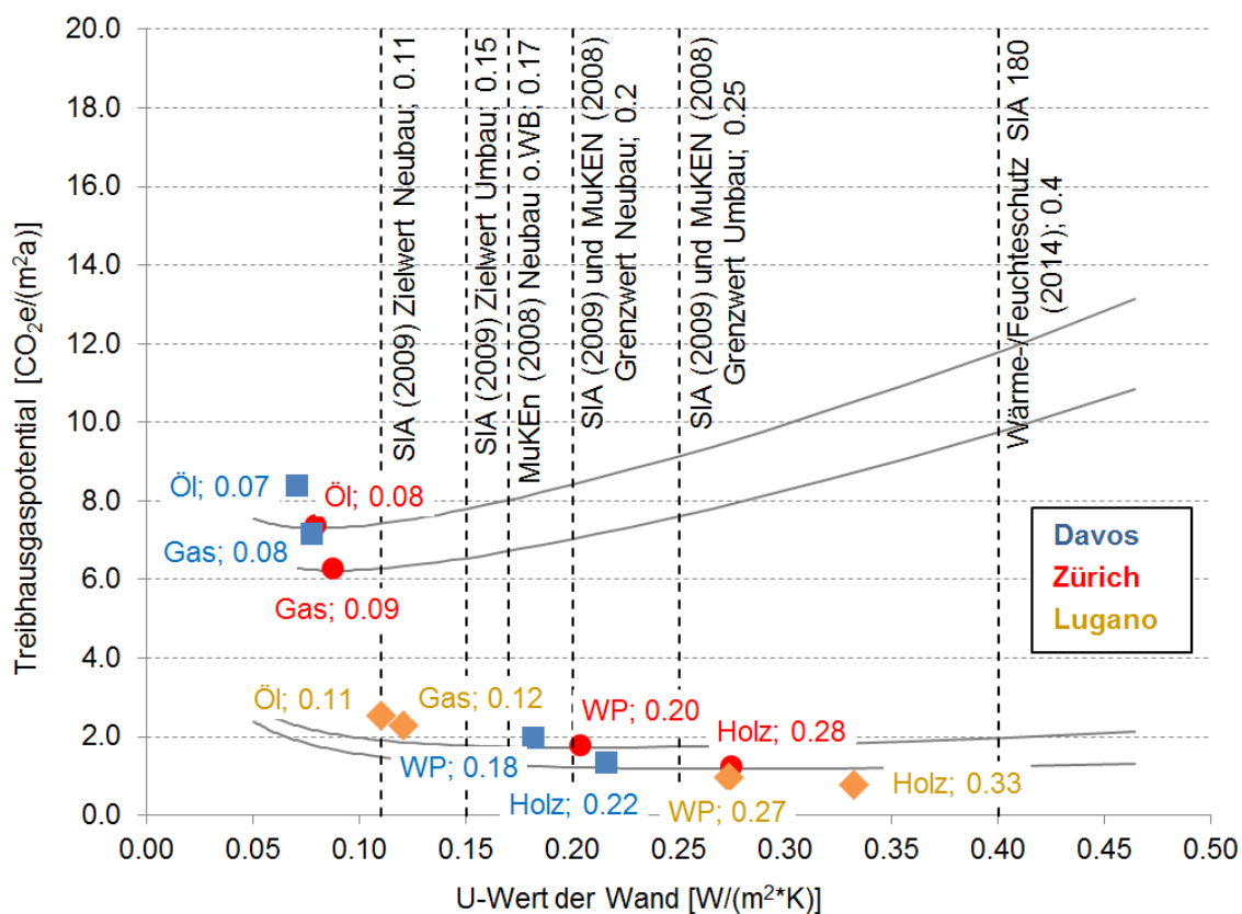
Fig. 31: Vergleich der optimalen Dämmstärken bezüglich des Umweltindikators Treibhausgaspotential mit normativen bzw. behördlichen Vorgaben
