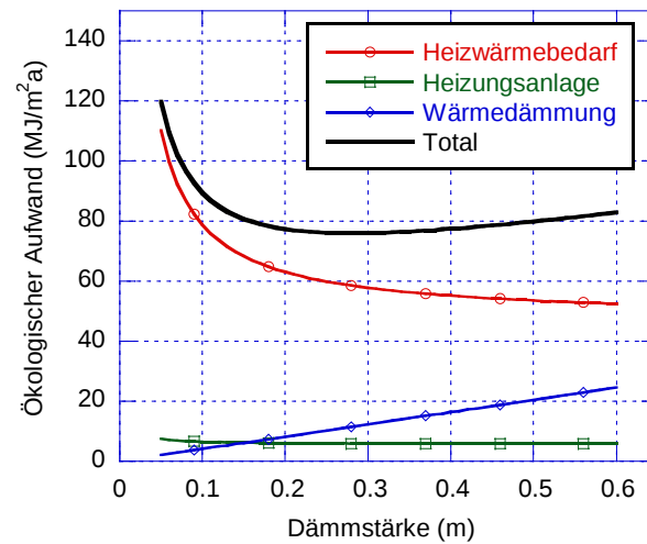
Fig. 9: Ökologischer Aufwand (Primärenergie) in Funktion der Dämmstärke, aufgeteilt nach Komponenten (Referenzfall Neubau)
