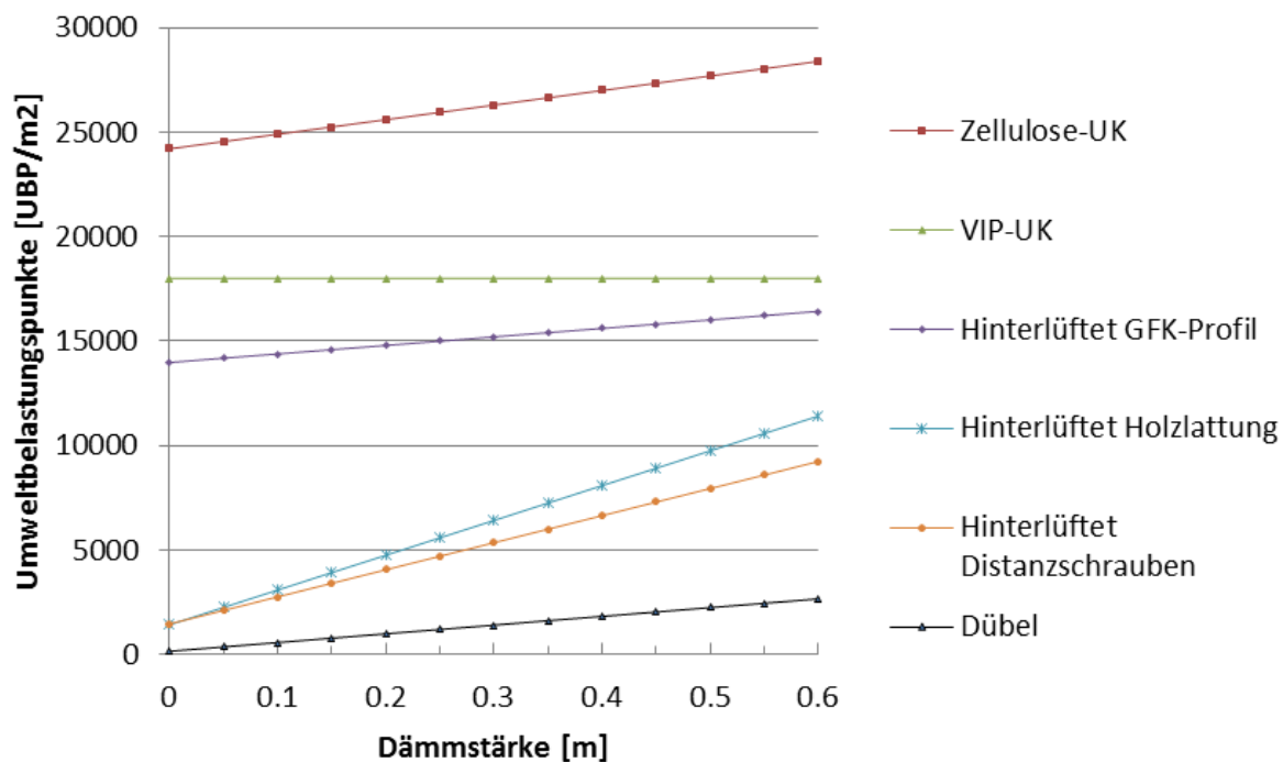
Ökologischer Aufwand (Umweltbelastungspunkte) von drei Unterkonstruktionen von hinterlüfteten Fassaden im Vergleich mit Unterkonstruktionen gemäss Kap. 2.6.1
