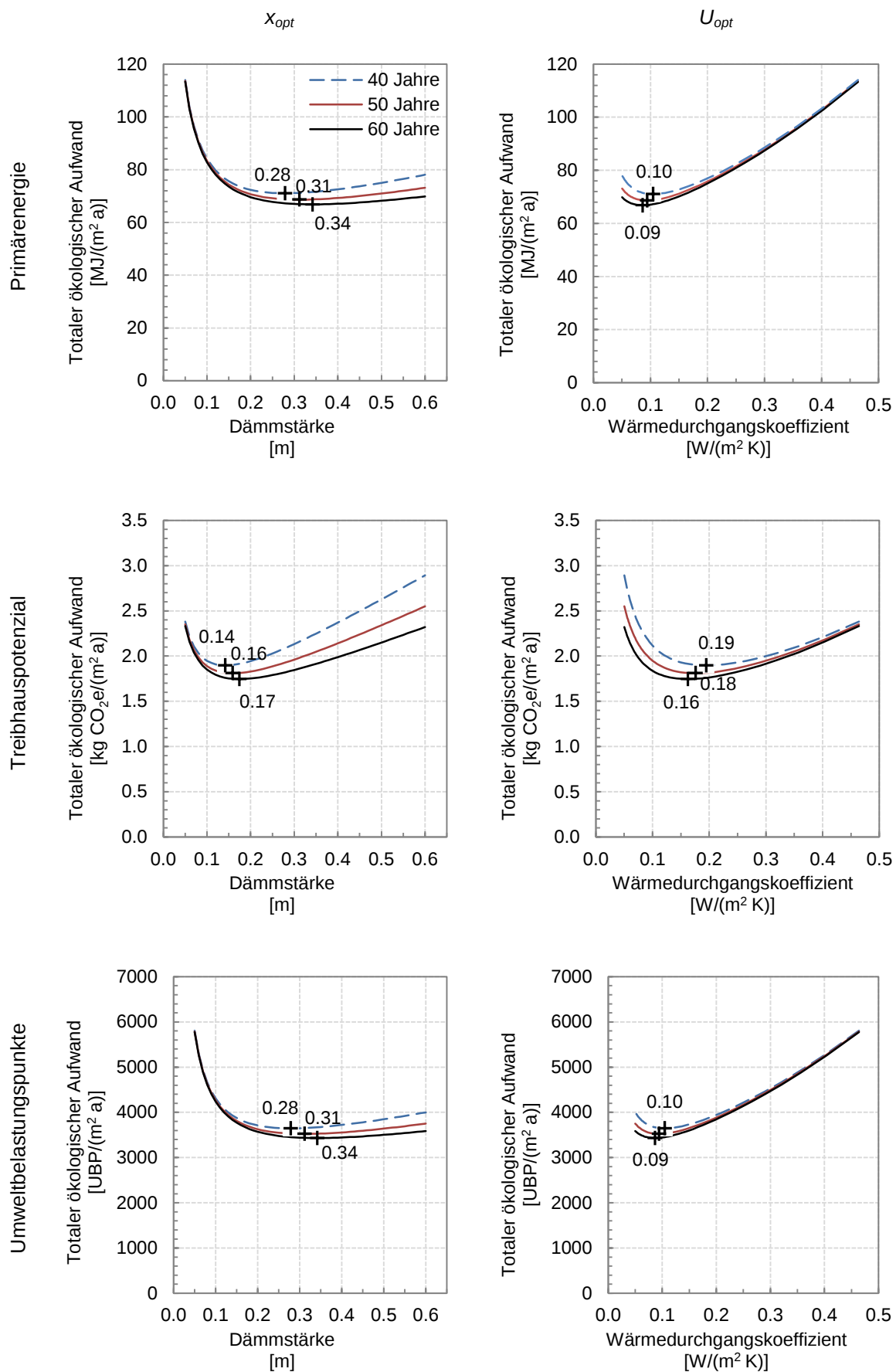
Fig. 20: Einfluss der Lebensdauer der Wärmedämmung (Referenzfall Neubau, WP JAZ=3.9)
