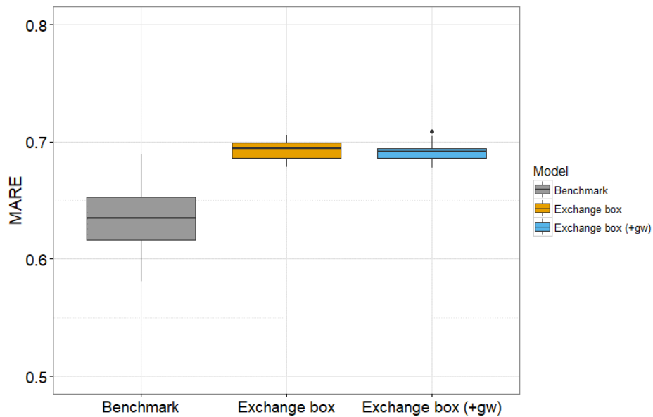
Abbildung 15 Das Gütemass F_{MARE} für die Kalibrierungsperiode für Bezugsmodell (benchmark) und das HBV_{exchange} -Modell mit Einbezug von nur Abfluss (Exchange box) sowie Grundwasser und Abfluss (Exchange box+gw).
