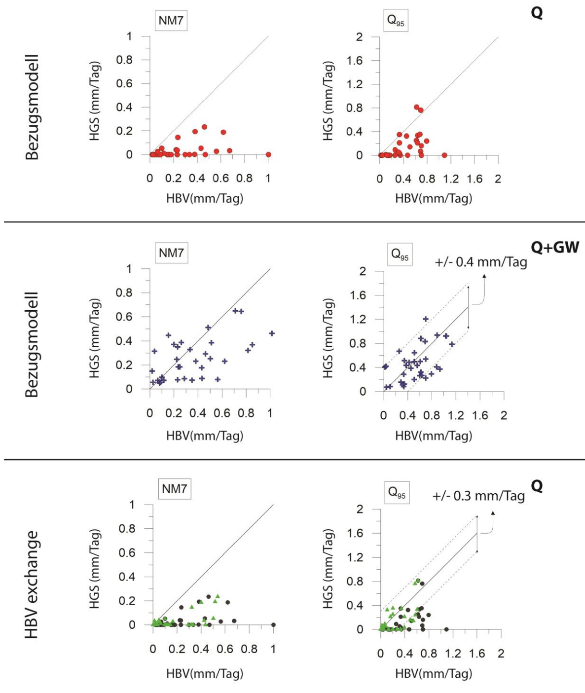
Abbildung 14 Auszug aus einer Reihe von Niedrigwasserkennwerten - hier NM7Q und Q 95 - um die Nachsimulierung des HGS Röthenbach-Modells und seinen Variationen mit HBV zu bewerten und Unsicherheiten abzuleiten. In der ersten Zeile wurde das Bezugsmodell nur mit Q (Oberflächen Abfluss) kalibriert. In der zweiten Zeile wurde das Benchmark
