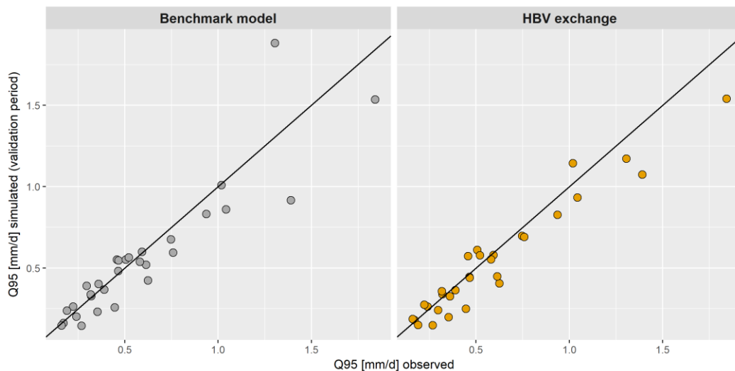
Abbildung 18 Vergleich der Simulationen des HBV_{exchange} -Modells mit dem Bezugsmodell hinsichtlich des Niedrigwasserkennwerts Q_{95} für die Validationsperiode (2002-2013).
