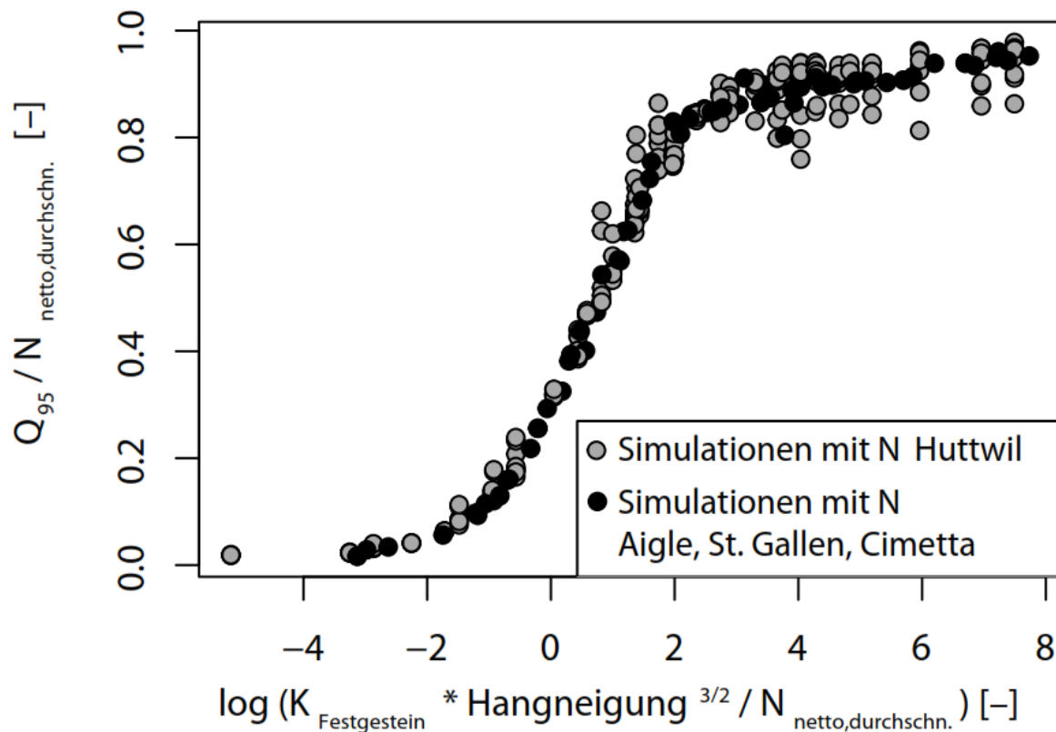
Abbildung 7 Das Verhältnis zwischen Q_{95} und dem durchschnittlichen Netto-Niederschlag N_{\text{netto,durchschn.}} ist gegen BPI geplottet. Jeder Punkt repräsentiert eine Modellkonfiguration. Nur Modelle ohne alluviale Grundwasserleiter, d.h. ausschliesslich mit Festgestein, sind eingeschlossen. Dafür beinhalten die gezeigten Daten zusätzliche Simulationen, in denen das Querschnittsverhältnis (aspect-ratio), die Porosität, und der Niederschlagsinput (in grau/schwarz) variiert wurden. Korrelation der linearisierten Beziehung: R^2 = 0.82 , p < 2.2e-16 .
