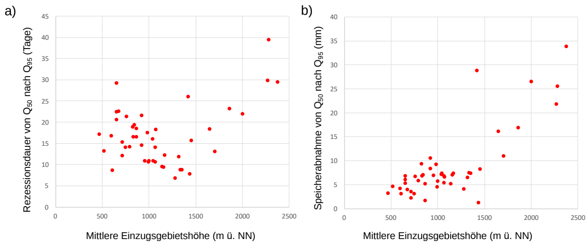
Abbildung 3 Rezessionsdauer (a) und Gebietsspeicherabnahme (b) von Q_{50} nach Q_{95} in Abhängigkeit der mittleren Einzugsgebietshöhe für 48 Einzugsgebiete in der Schweiz.
