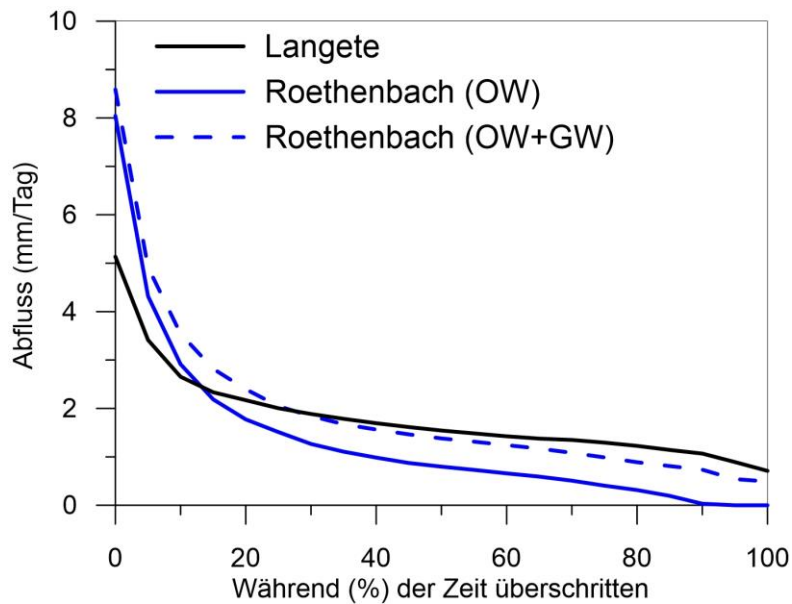
Abbildung 11 Simulierte Dauercurven des Röthenbachs und der Langeten. Für den Röthenbach wurde wie für die Langeten die Dauerkurve für den Oberflächenabfluss (OW) erstellt, sowie die Dauerkurve für die Summe von Oberflächenabfluss und Grundwasserabfluss (OW+GW).
