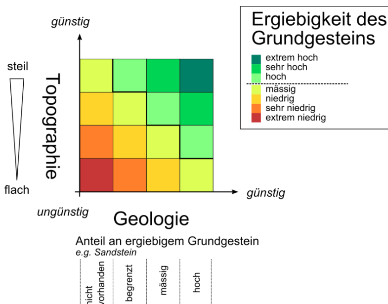
Abbildung 22 Schematische Darstellung der Beziehung zwischen der Ergiebigkeit des Festgesteins zu der Geologie und dem Gefälle (nicht maßstabgetreu).
