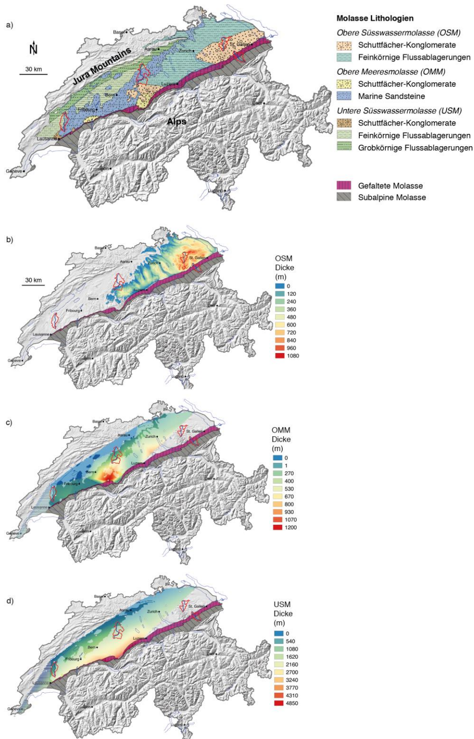
Abbildung 20 Überblick der (a) Molasselithologien basierend auf paläo-sedimentologischen Modellen (Trümpy, 1980) und der Mächtigkeit der (b) Oberen Süsswassermolasse OSM (Gander, 2004), der (c) Oberen Meeresmolasse OMM und der (d) Unteren Süsswassermolasse USM (graue Punkte = verwendete Tiefbohrungen; zusammenfassende Referenz: (Sommaruga et al., 2012) Dunkle Farben in (b) bis (d) zeigen, wo die entsprechende Molasseeinheit an der Oberfläche oder unter quartären Ablagerungen vorhanden ist. Die horizontal schraffierte Fläche nordwestlich von Lausanne zeigt ein Gebiet mit erhöhter Unsicherheit der Mächtigkeiten aufgrund tektonischer Brüche. In rot: Fünf detailliert untersuchte Einzugsgebiete mit dem Verlauf des Hauptflusses in blau ausgewählt aufgrund ihrer grossen Spannweite des Q_{95}/Q_{50} Kennwerts und gut positionierten hydrologischen Messstationen (auf Festgestein). Die Einzugsgebiete mit einem hohen Anteil marinen Sandsteins als Festgestein zeigen die höchsten Q_{95}/Q_{50} Werte (Langete-Rotbach, Huttwil; Murg, Murgenthal).
