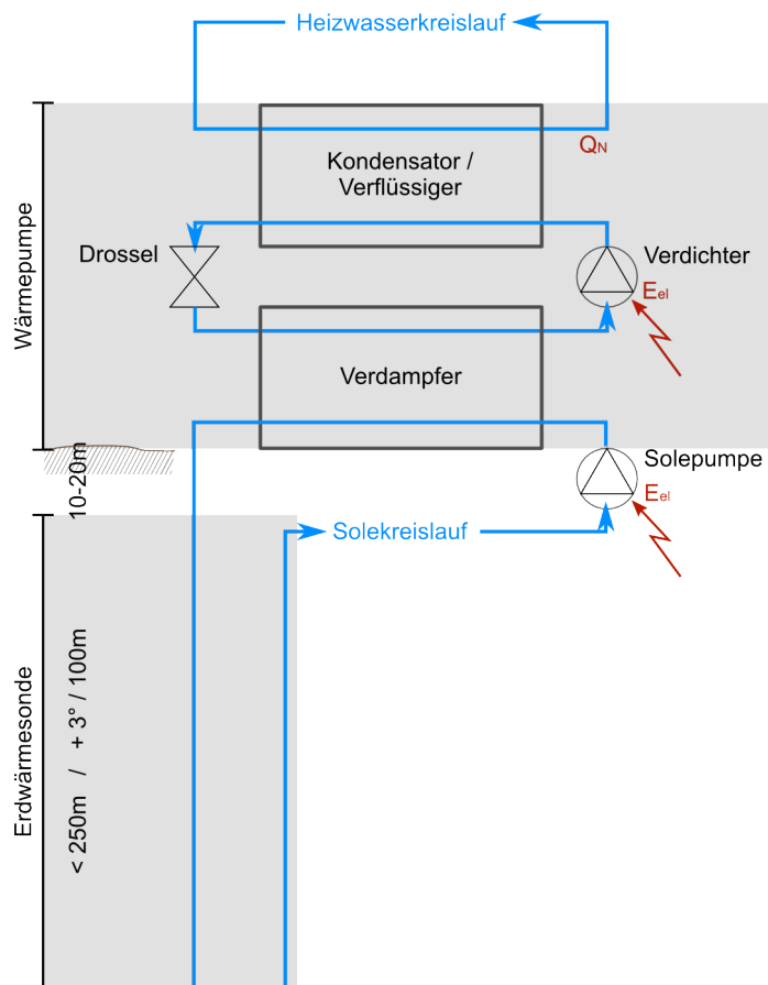
Abbildung 91: Systemkomponenten Sole-Wasser-Wärmepumpe
