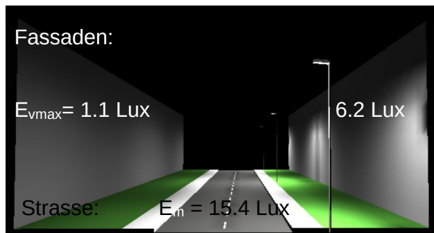
Bild 3: Visualisierung einer Strassenbeleuchtung mit Fassaden
