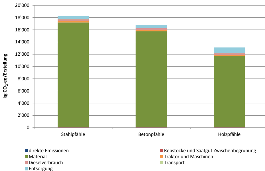
Abbildung 5-7: Treibhauspotenzial [kg CO 2 -eq] der Neuerstellung einer Hektare Rebanlage mit Stahlpfählen, Betonpfählen und Holzpfählen
