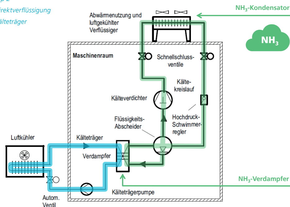
Abbildung 4: Die Kälteabgabe erfolgt über einen sekundären Kälte-träger-Kreislauf.
