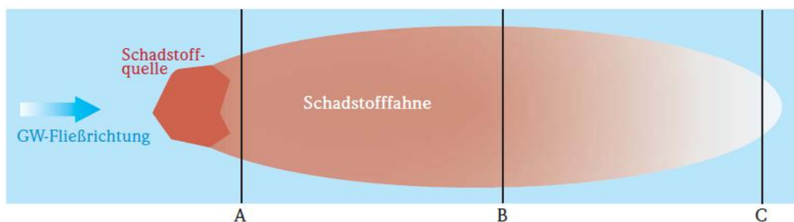
Abbildung 8 Darstellung von Transekten (Quelle: Handbuch Altlasten, Bundesland Hessen)
