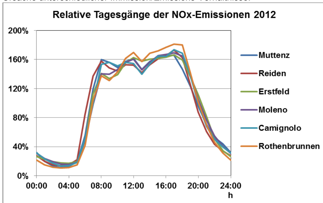
Abbildung 3.1: Relative Tagesgänge der NOx-Emissionen 2012 der A2 bzw. A13 an den sechs MfMU-Standorten. 100% = Jahresmittel je Standort.
