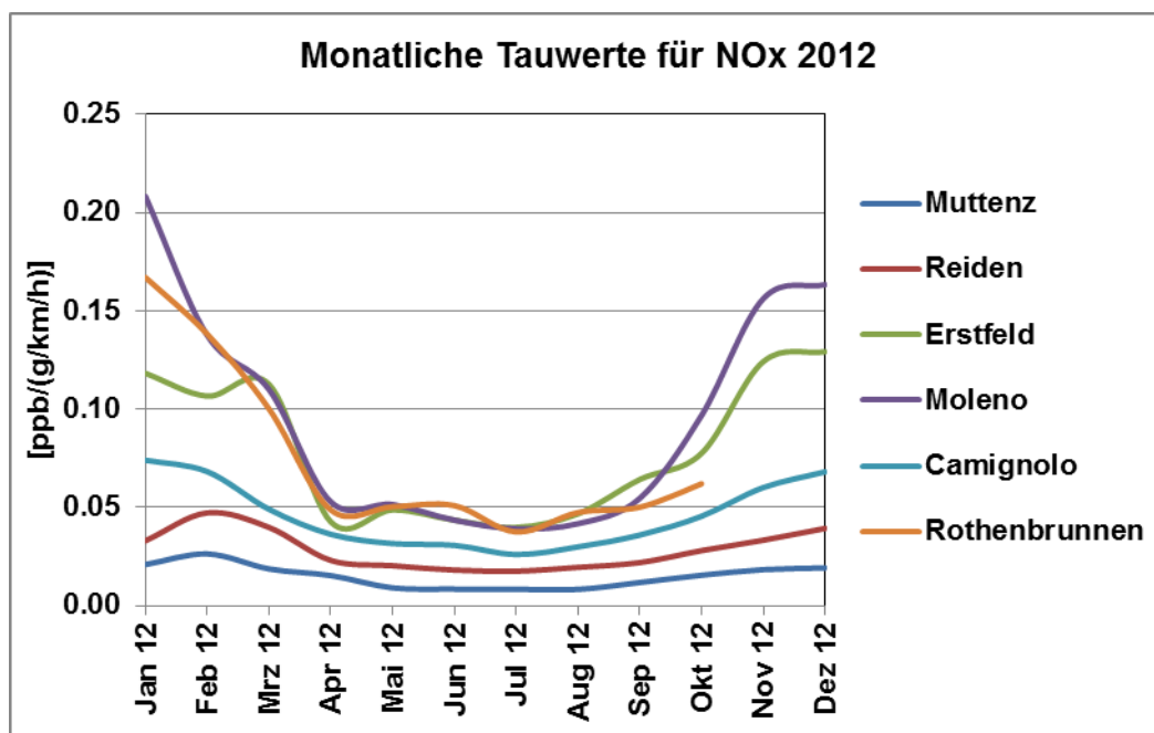
Abbildung 3.2: Monatliche Mittelwerte für Tau von NOx 2012 an den sechs MfMU-Standorten.
