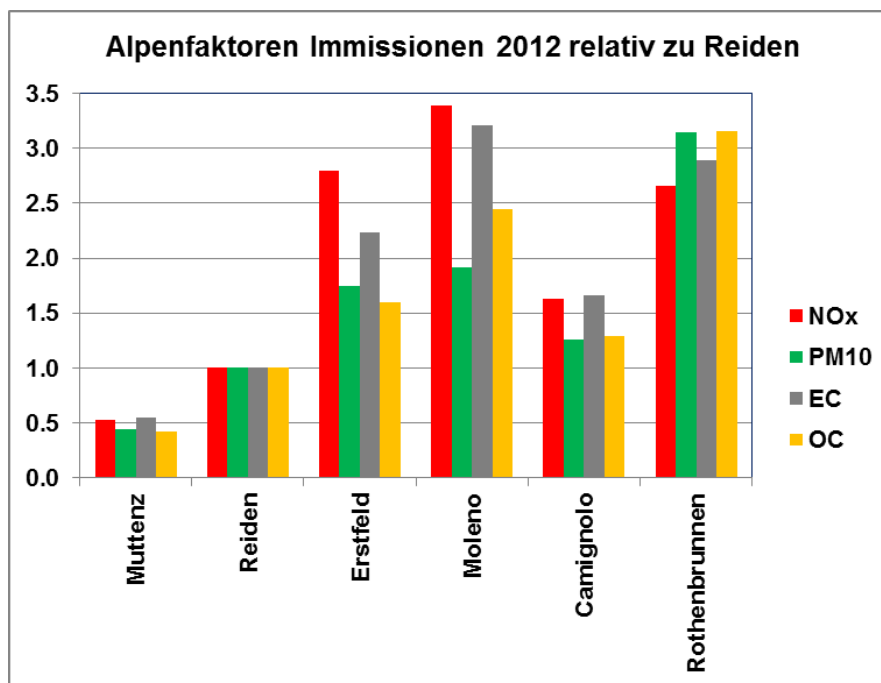
Abbildung 4.1: Alpenfaktoren der Immissionen an NO x , PM 10 , EC und OC für die MfMU-Stationen relativ zu Reiden, 2012.
