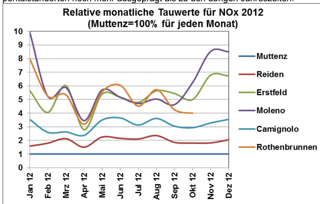
Abbildung 3.3: Relative monatliche Mittelwerte für Tau von NOx 2012 an den sechs MfMU-Standorten, Wert für MuttENZ=1 für jeden Monat.
