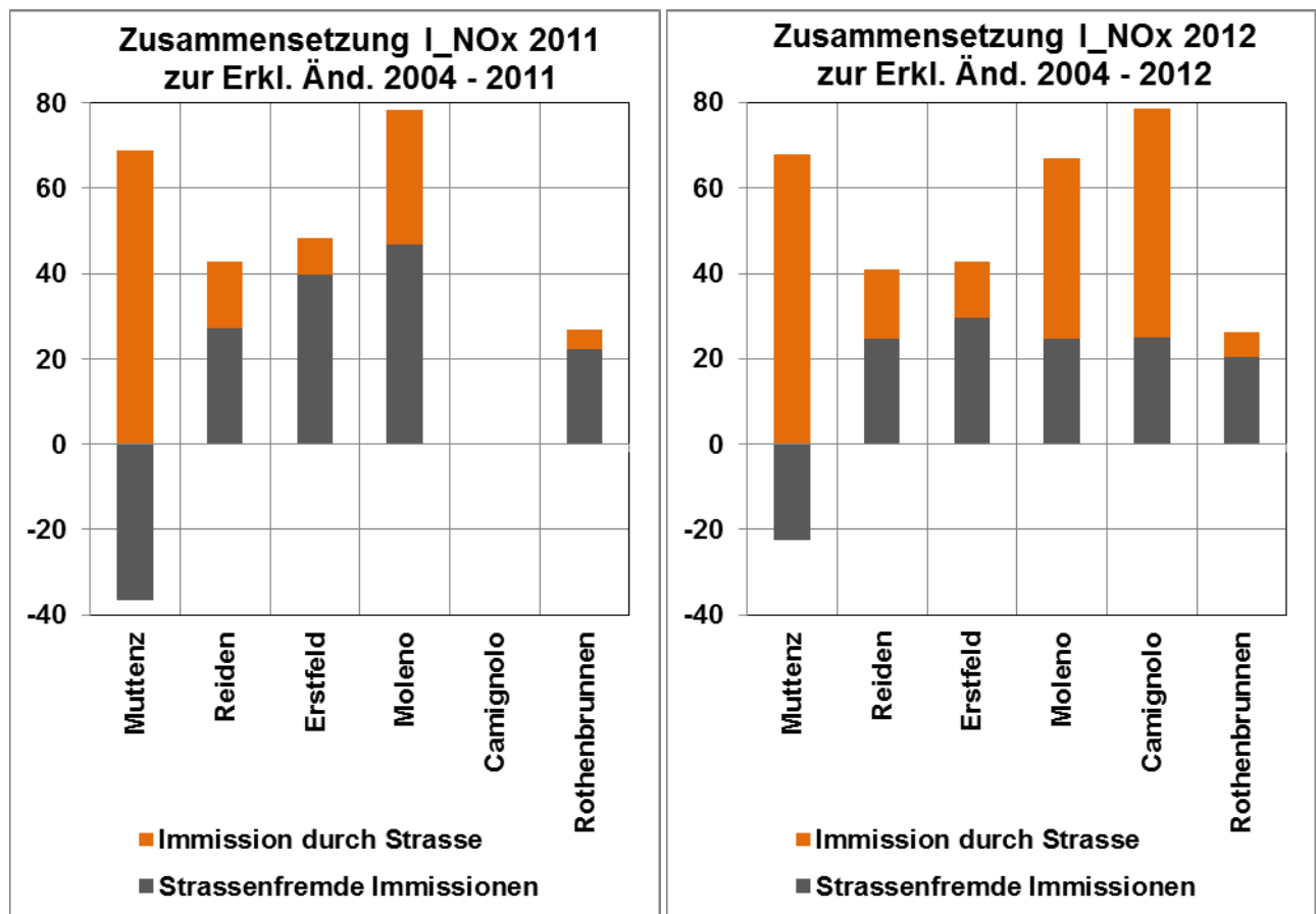
Abbildung 5.1: (Virtuelle!) Zusammensetzung der NO x -Immissionen an den MfMU-Standorten nach strassenseitigen und strassenfremden Anteilen zur Erklärung der unterschiedlichen Entwicklung der NO x -Emissionen und –Immissionen 2004-2011 (links) bzw. 2004-2012 (rechts).
