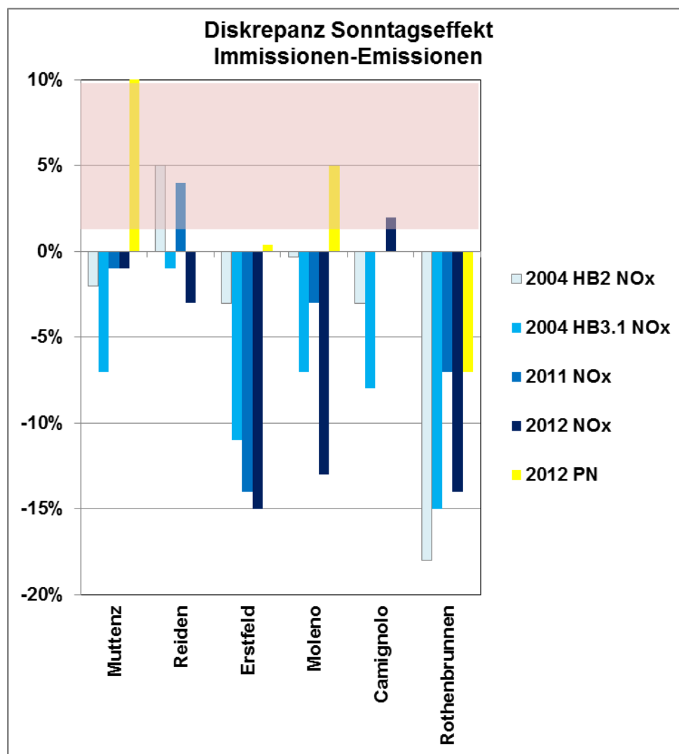
Abbildung 5.2: Sonntagseffekte an den MfMU-Standorten für NOx 2004-2012 und Partikelanzahlkonzentration (PN) 2012. Rosa Zone: Erwartungsbereich der Differenz Immissionen – Emissionen bei den Sonntagseffekten.
