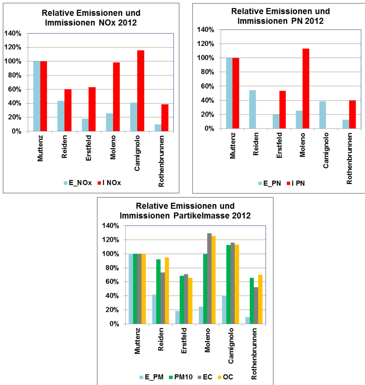
Abbildung 2.1: Emissionen und Immissionen bei den MfMU-Standorten 2012 relativ zu Muttentz (Wert bei Muttentz = 100% für jede Komponente). PN: Partikelanzahlkonzentration.
