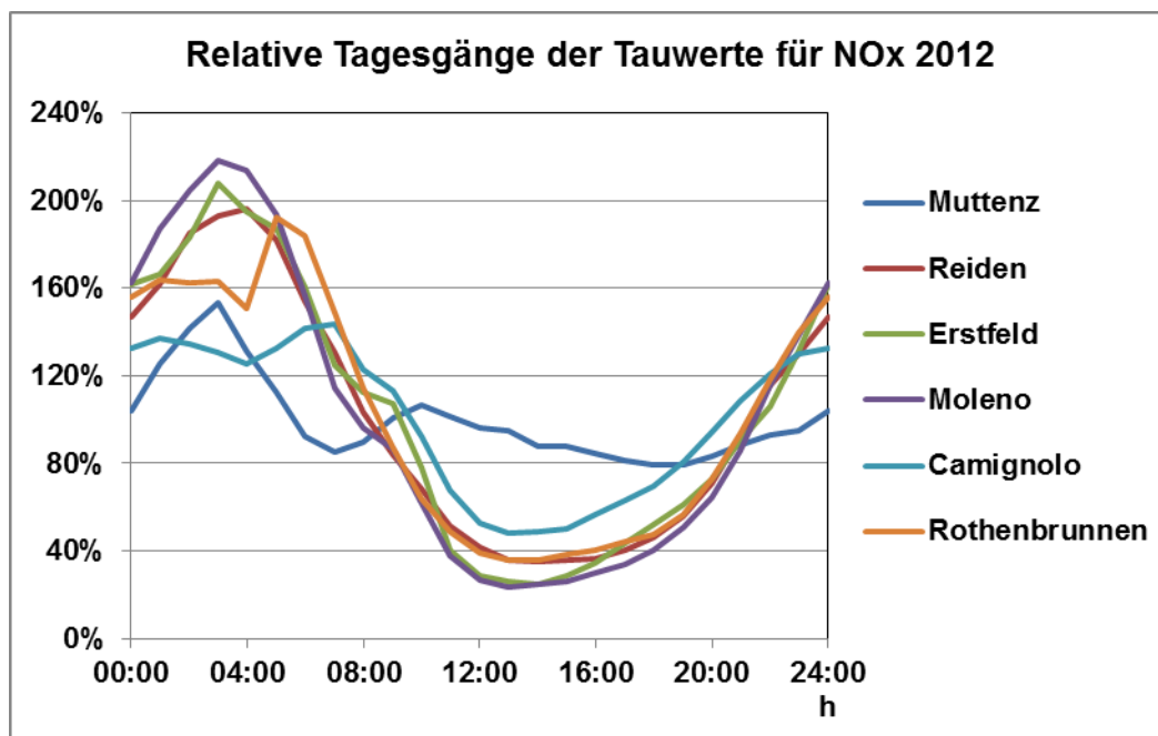
Abbildung 3.4: Relative Tagesgänge der Tauwerte für NOx 2012 an den sechs MfMU-Standorten. 100% = Jahresmittel je Standort.
