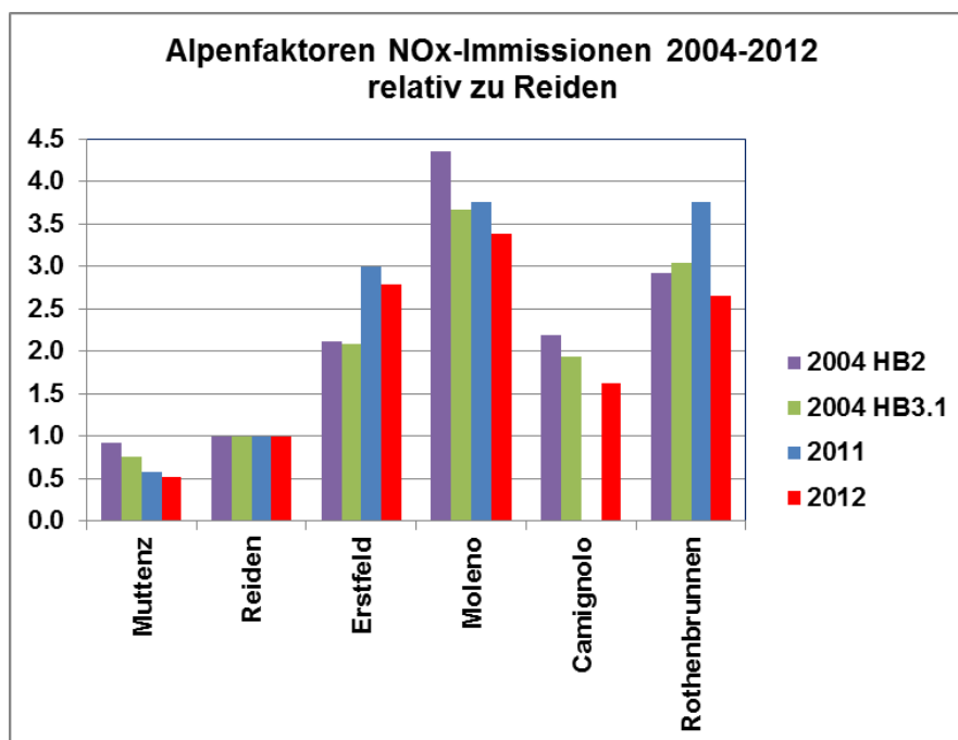
Abbildung 4.2: Alpenfaktoren der NO x -Immissionen für die MfMU-Stationen relativ zu Reiden, Entwicklung von 2004 – 2012.
