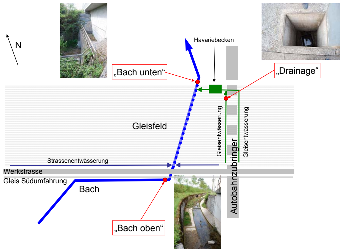
Abb. 2 Schematischer Situationsplan vom Standort RBL. Die Probenahmestellen sind rot eingezeichnet.
