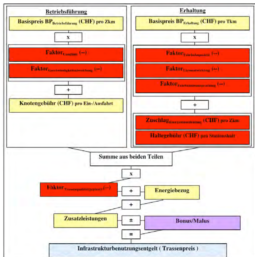
Abbildung 1 Systemansatz und Struktur des IVT-Trassenpreissystems, Arbeitsstand Nov. 2007
