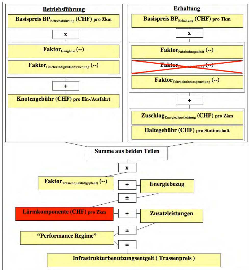
Abbildung 19 Angepasste Struktur des IVT-Trassenpreissystems
