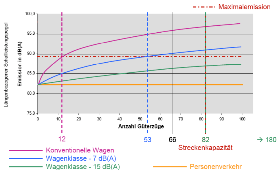
Abbildung 2 Berechnungsmodell „Lärmkapazität“; Quelle [6]
