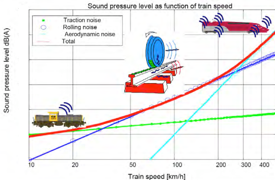
Abbildung 5 Geräuschquellen und ihre typische Geschwindigkeitsabhängigkeit; Quelle [14]
