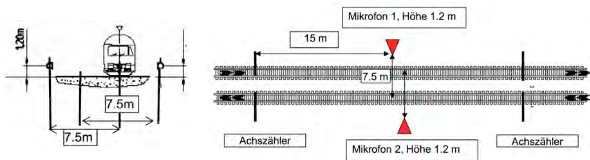
Abbildung 14 Aufbau Messstandort für das Monitoring Eisenbahnlärm Schweiz; Quelle [17]
