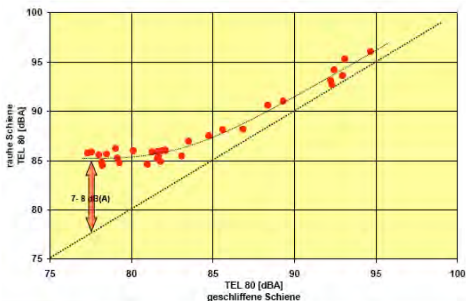
Abbildung 6 Vergleich der Emissionswerte auf geschliffener und rauer Schiene; Quelle [17]
