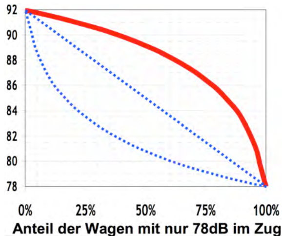
Abbildung 15 Gesamtpegel des Zuges, abhängig vom Anteil Wagen mit 78 dB(A); Quelle [7]
