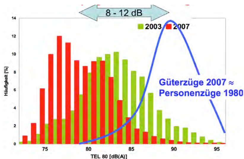
Abbildung 13 Vorbeifahrtspegel Güter- und Personenzüge; Quelle [23]
